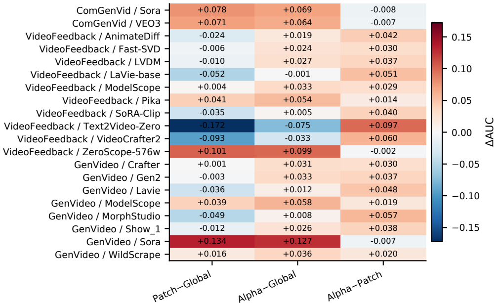
Per-generator AUC deltas
