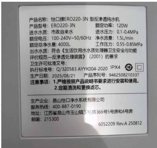
ERO220-3N(铭牌)
