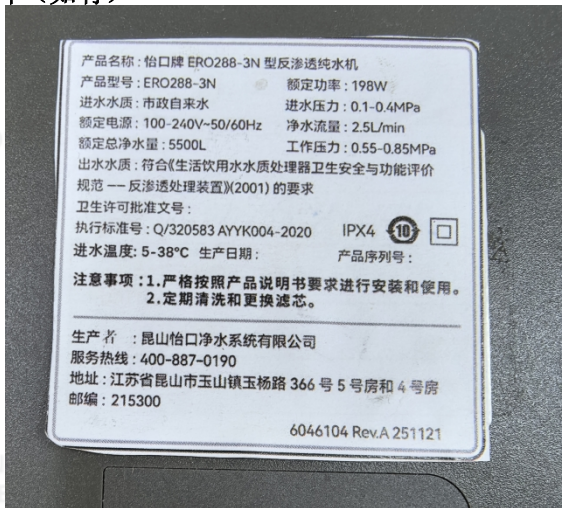
ERO288-3N(铭牌)
