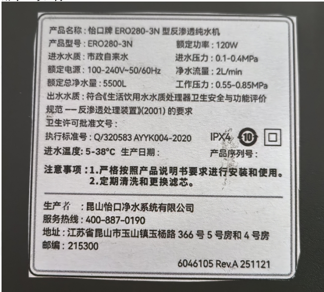
ERO280-3N(铭牌)
