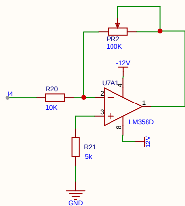
P 比例调节设计
