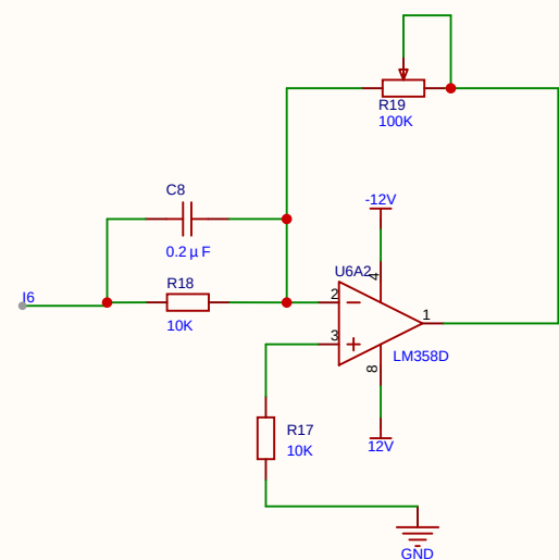
D微分调节设计
