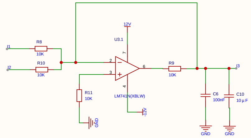
运放加法器电路
