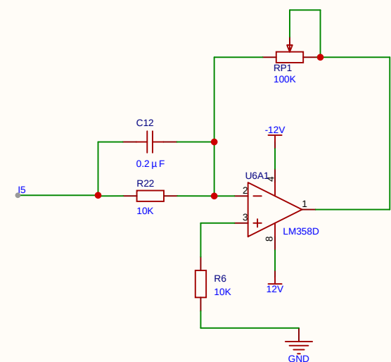
I 积分调节设计
