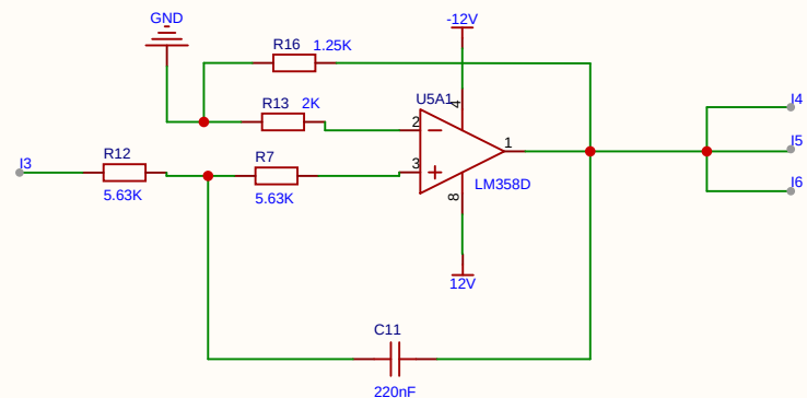
巴特沃斯一阶低通滤波器设计
