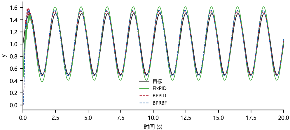
16. Plant3 正弦低频 r=1+0.5\sin
