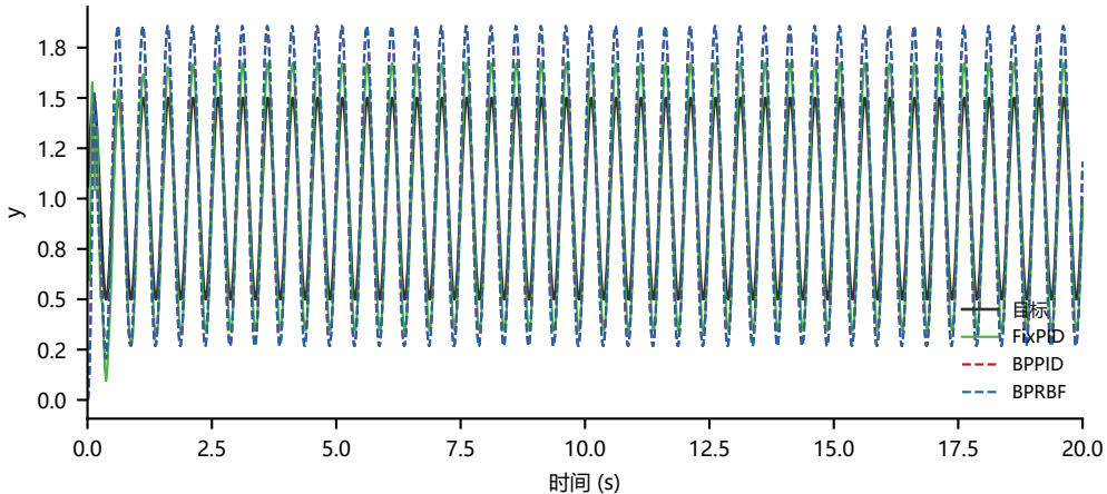
17. Plant3 正弦高频 r=1+0.5\sin
