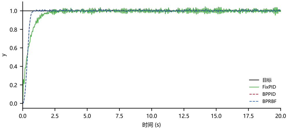
20. Plant3 量测噪声
