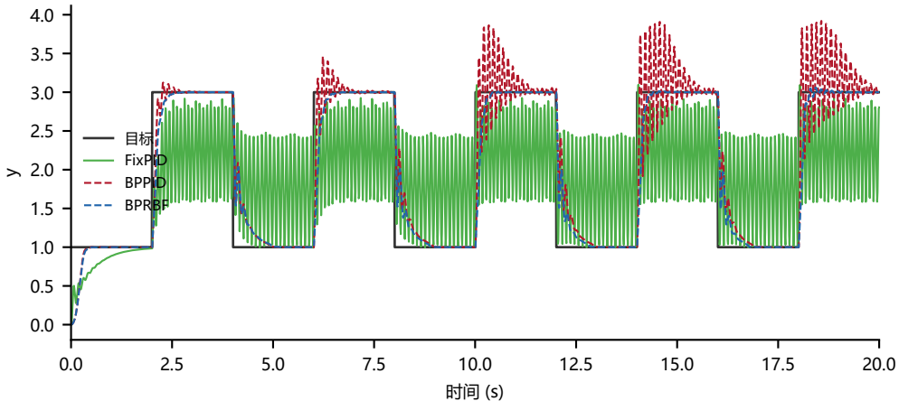
21. Plant3 方波 (1 3)
