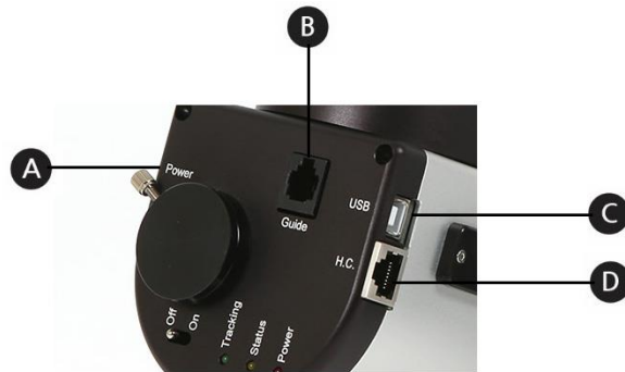
그림 3-2 케이블 연결
