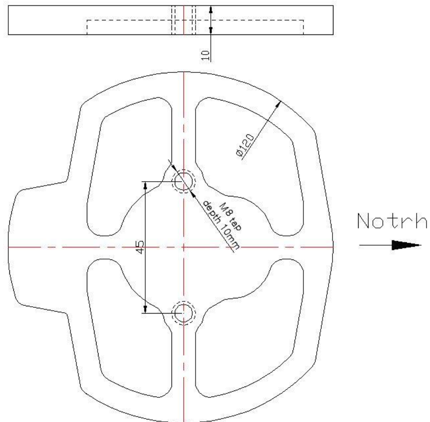
그림 4-2 적도의 하단(피어) 연결부 도면
