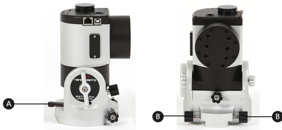
그림 3-3 방위 조절 위치
