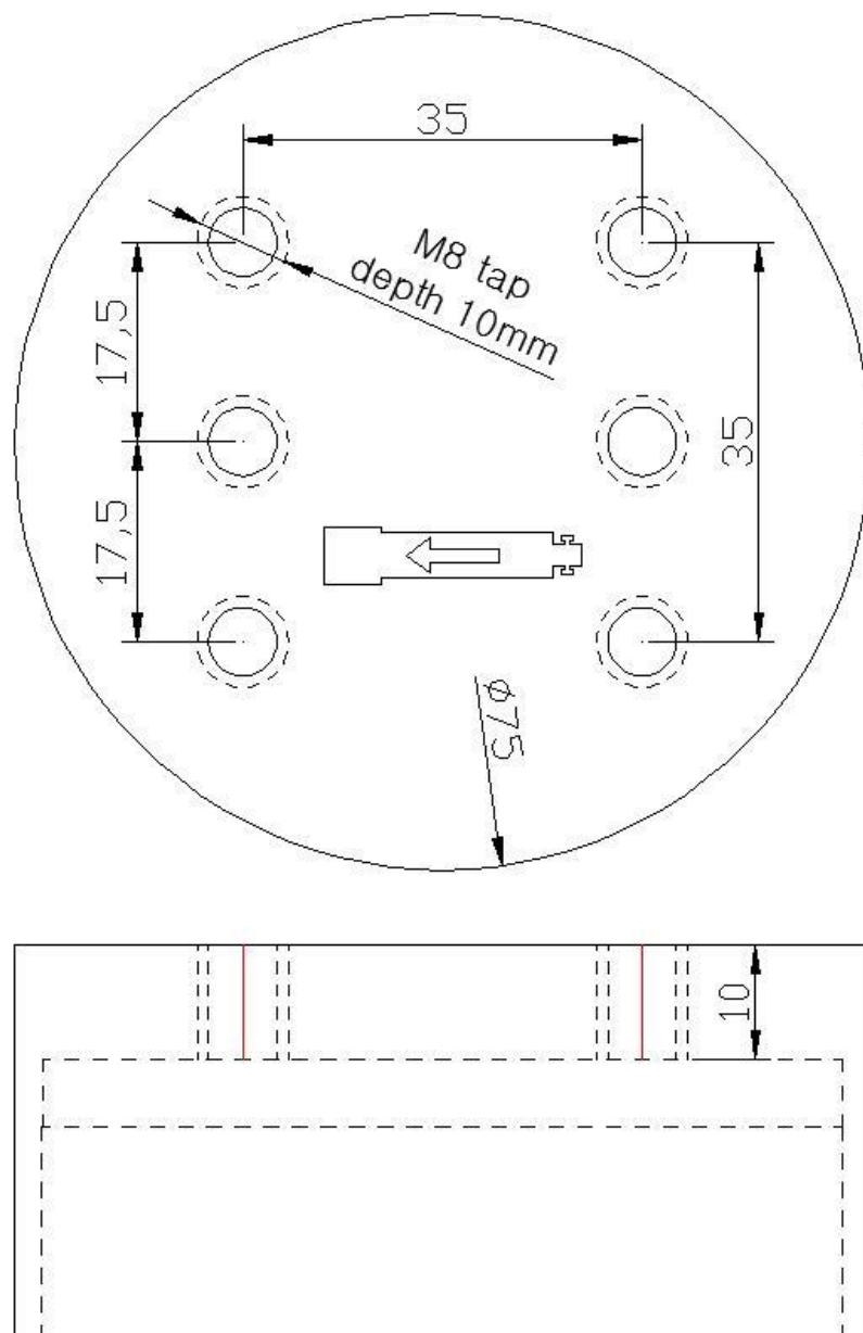
그림 4-1 적위 헤드 도면
