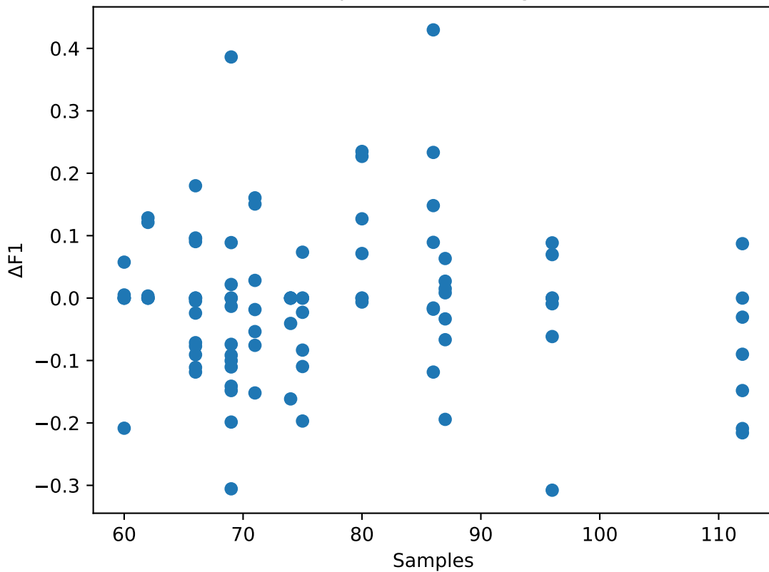
Samples vs \Delta F1 - Logistic
