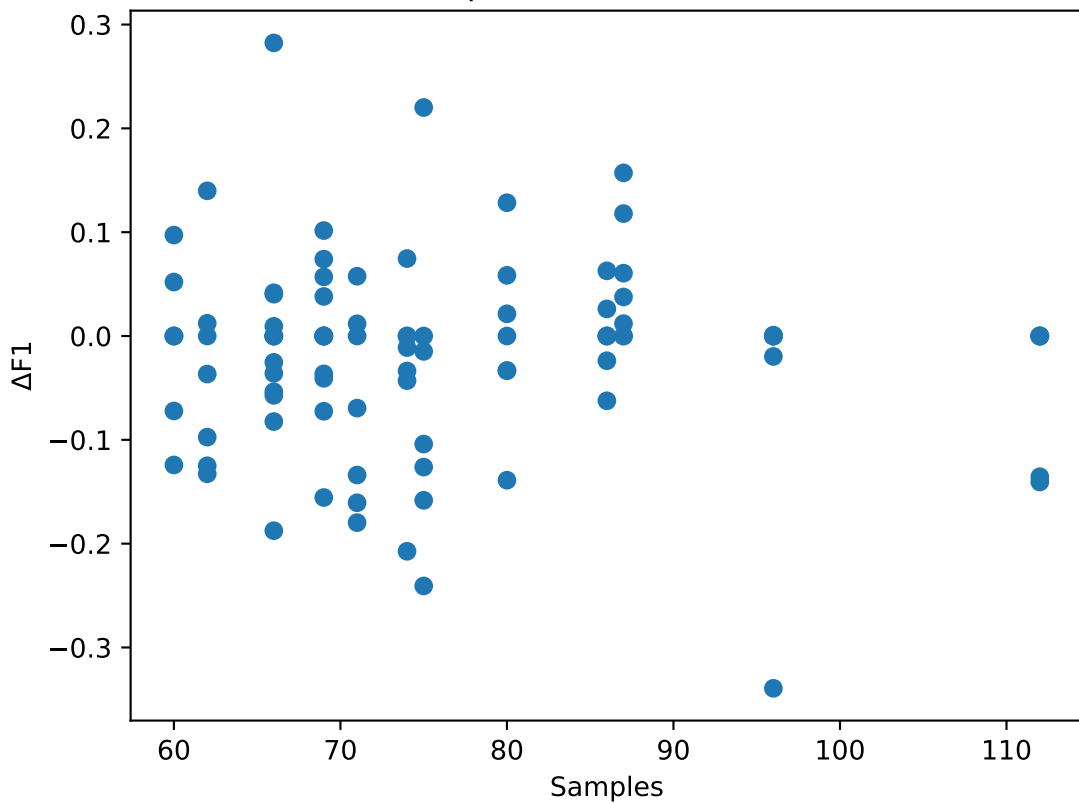
Samples vs \Delta F1 - XGBoost
