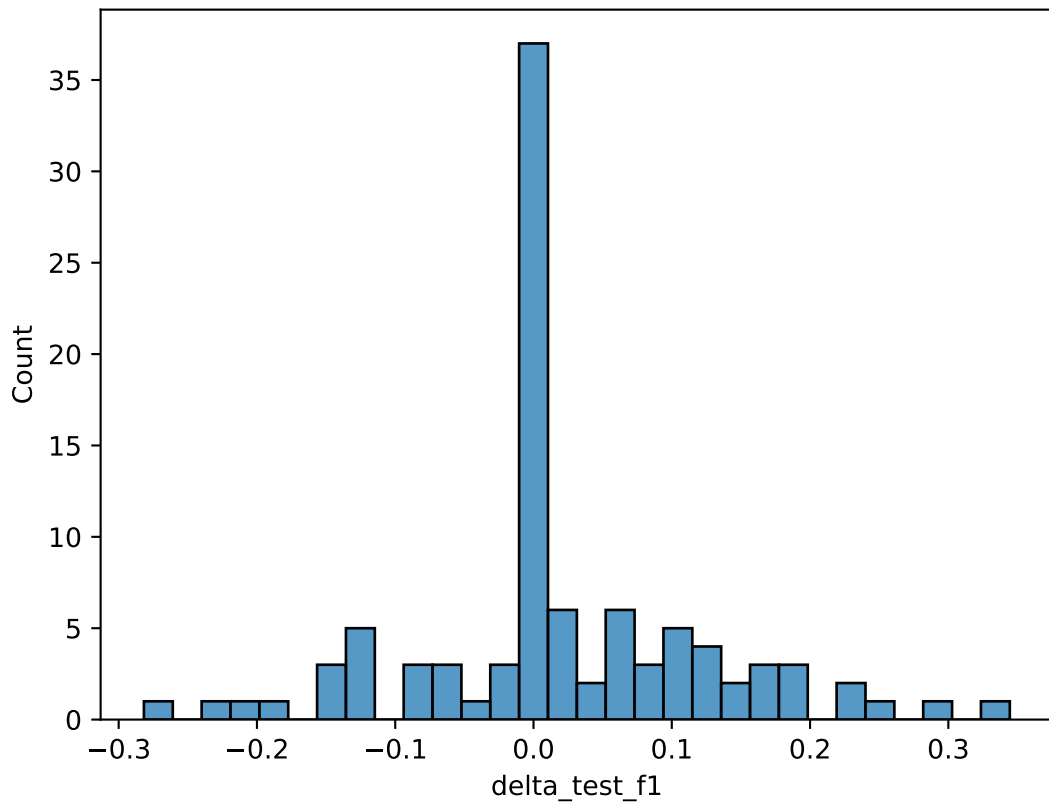
\Delta F1 Distribution - RandomForest
