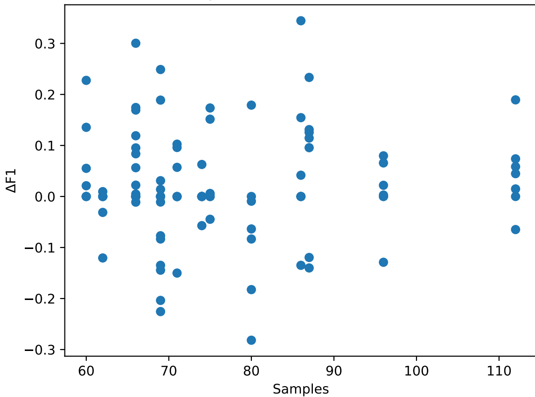
Samples vs \Delta F1 - RandomForest
