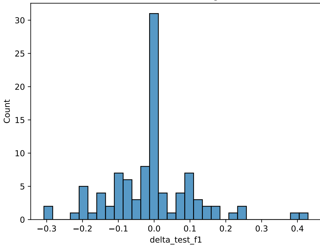
\Delta F1 Distribution - Logistic
