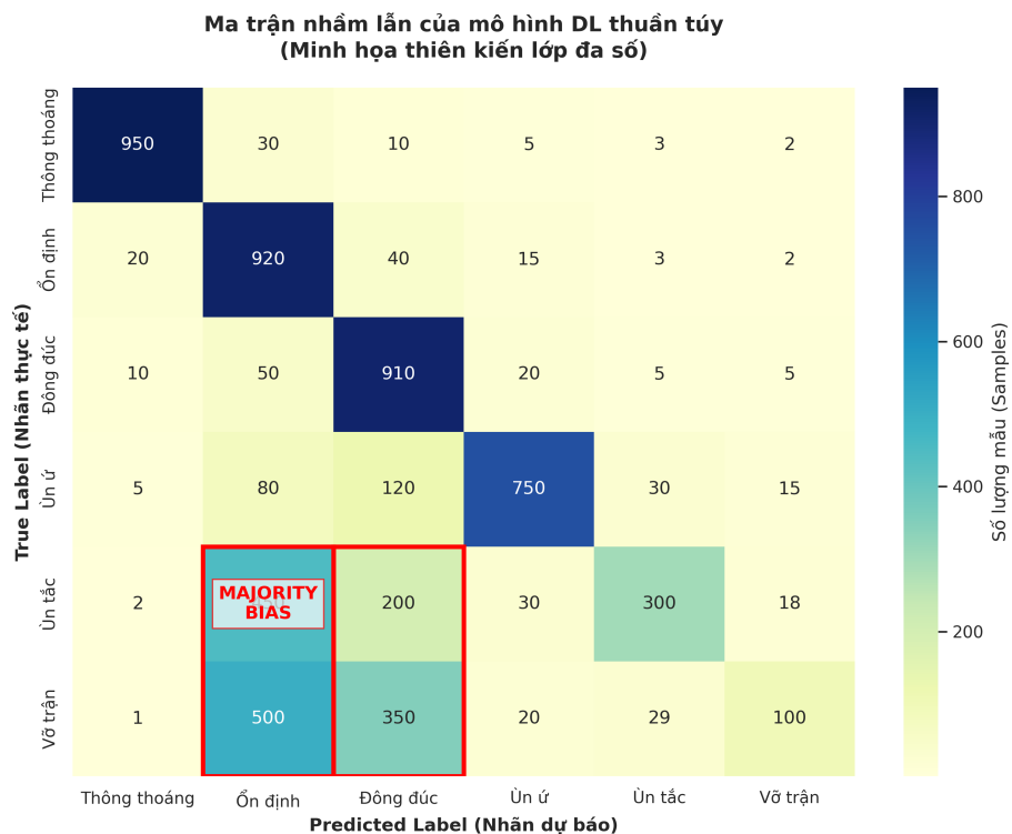
Hình 16: Ma trận nhầm lẫn mô hình DL thuần túy
