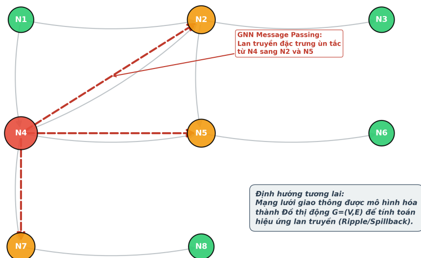
Hình 37: Tích hợp Mạng Nơ-ron Đồ thị (GNN)
