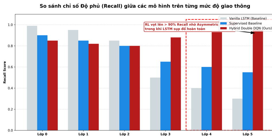
Hình 36: So sánh Độ phủ (Recall) chi tiết trên từng mức độ giao thông
