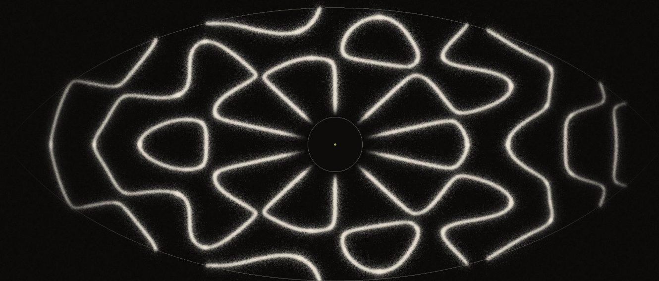
— PL. I · MODOS 5,5 + 12,3 · 432 Hz · AREIA SOBRE PLACA EM VIBRAÇÃO
