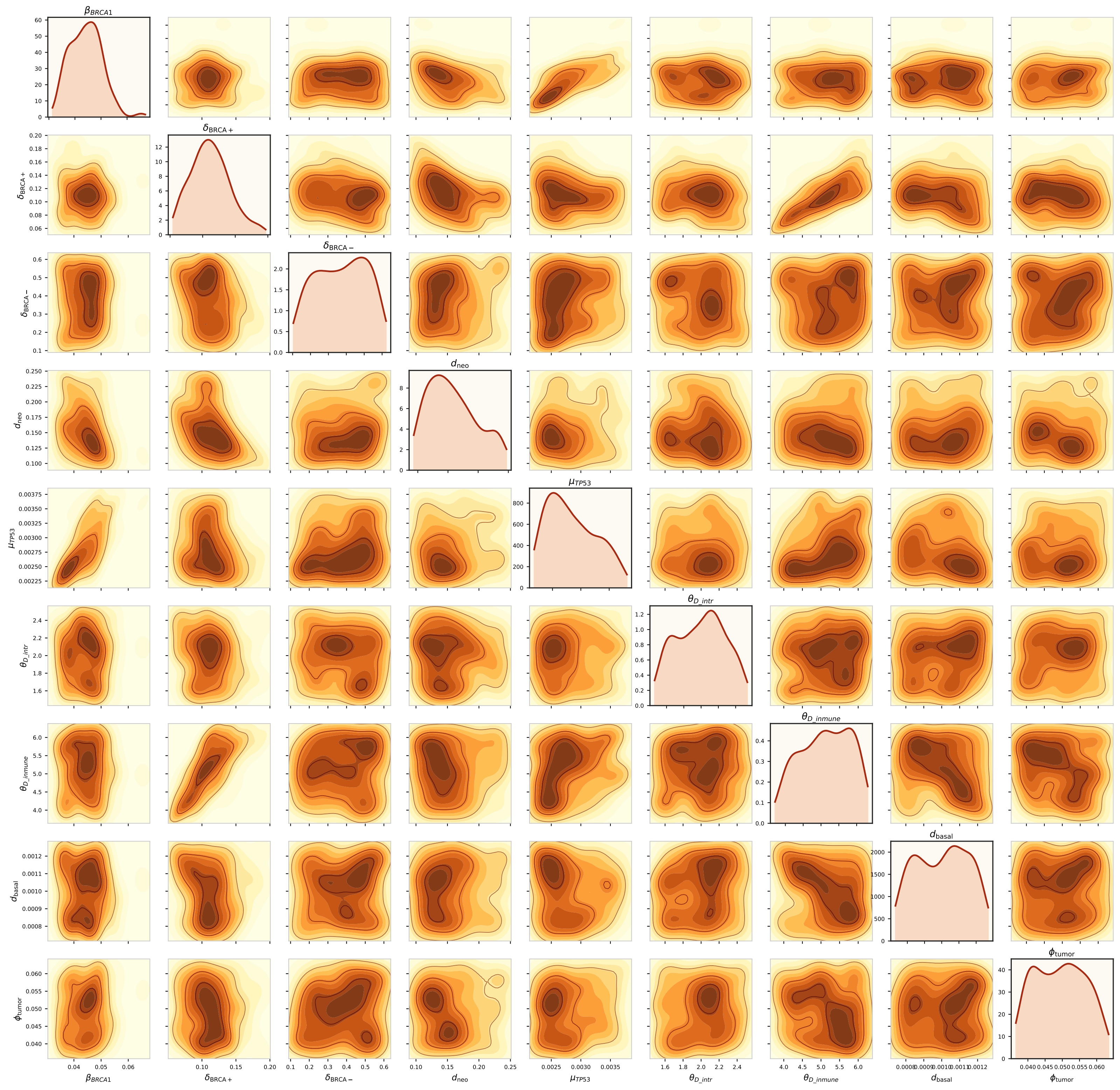
Full 9-Dimensional Parameter Posterior Space: Nivel 2 ( \pm 25\% - Variabilidad Moderada)
