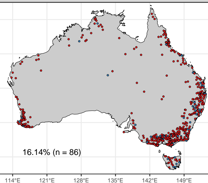
CO2 Slope
