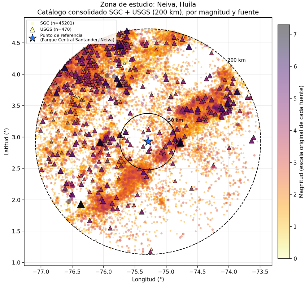
Figura 2: Epicentros del catálogo consolidado SGC + USGS dentro de 200 km alrededor de Neiva, coloreados por magnitud y diferenciados por fuente.
