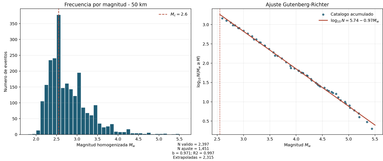
Figura 3: Frecuencia y ajuste Gutenberg–Richter del catálogo homogenizado dentro de 50 km. La línea vertical indica la magnitud de completitud exploratoria M_c = 2,55 .
