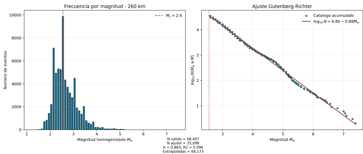
Figura 4: Frecuencia y ajuste Gutenberg–Richter del catálogo homogenizado dentro de 260 km. La línea vertical indica la magnitud de completitud exploratoria M_c = 2,55 .
