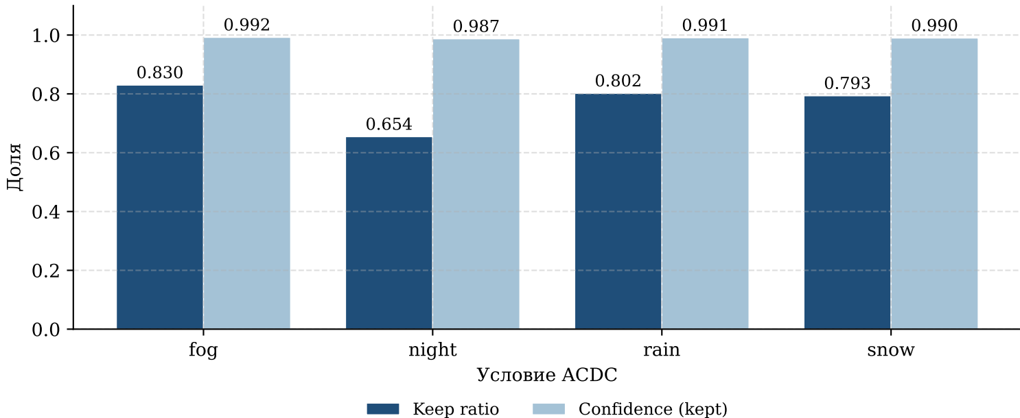
U1: фильтрация pseudo-labels на ACDC train, \tau = 0.90
