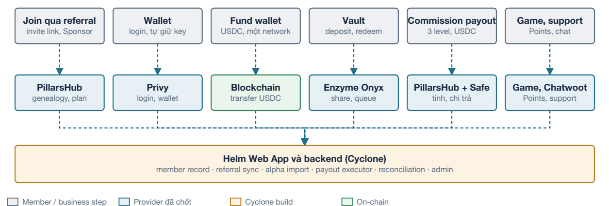
Hình 1: Các business capability, platform cung cấp từng capability và phần Cyclone build.
