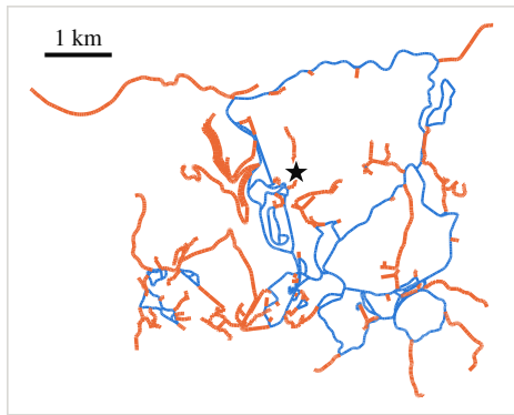
(a) Pontes identificadas por Tarjan
