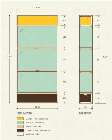
结构图 · 正立面与侧剖面尺寸标注
