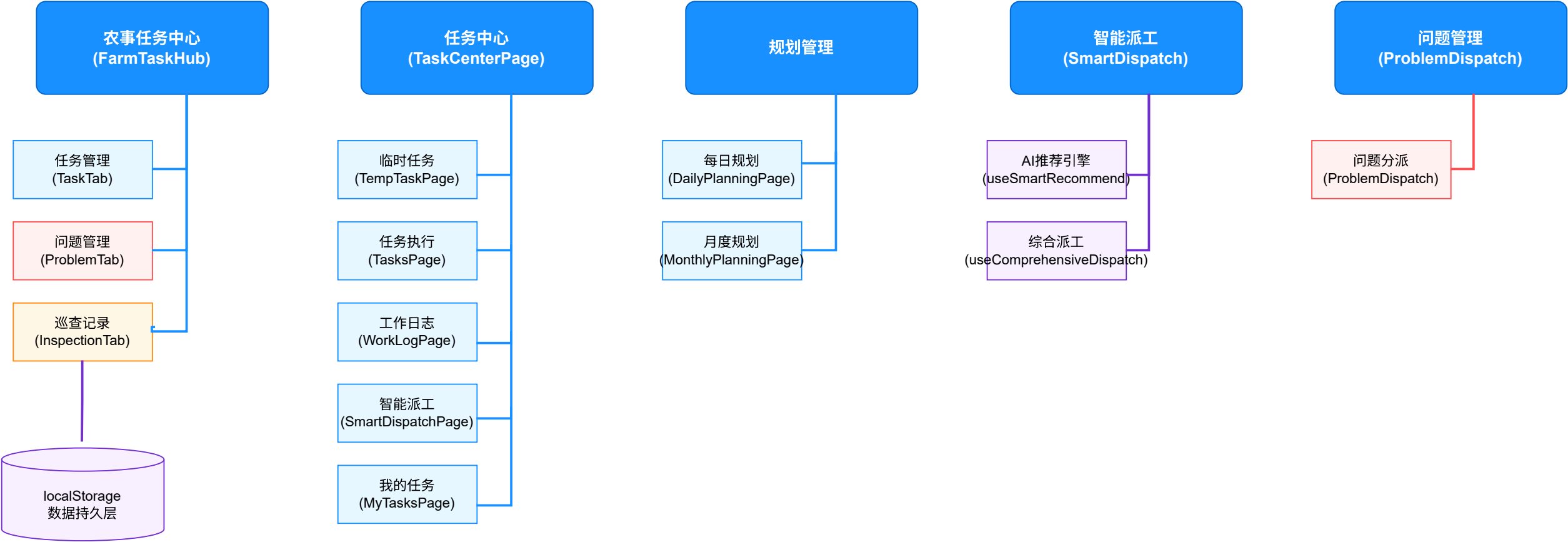
农事管理模块整体架构图
