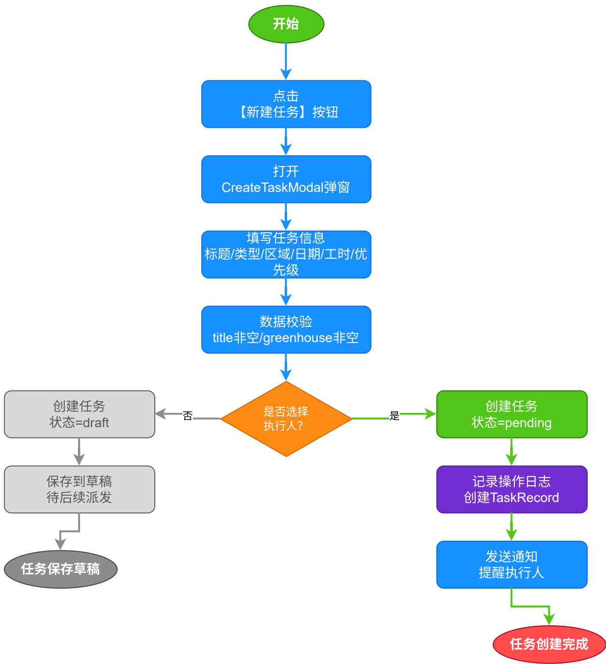
F01 任务创建流程图
