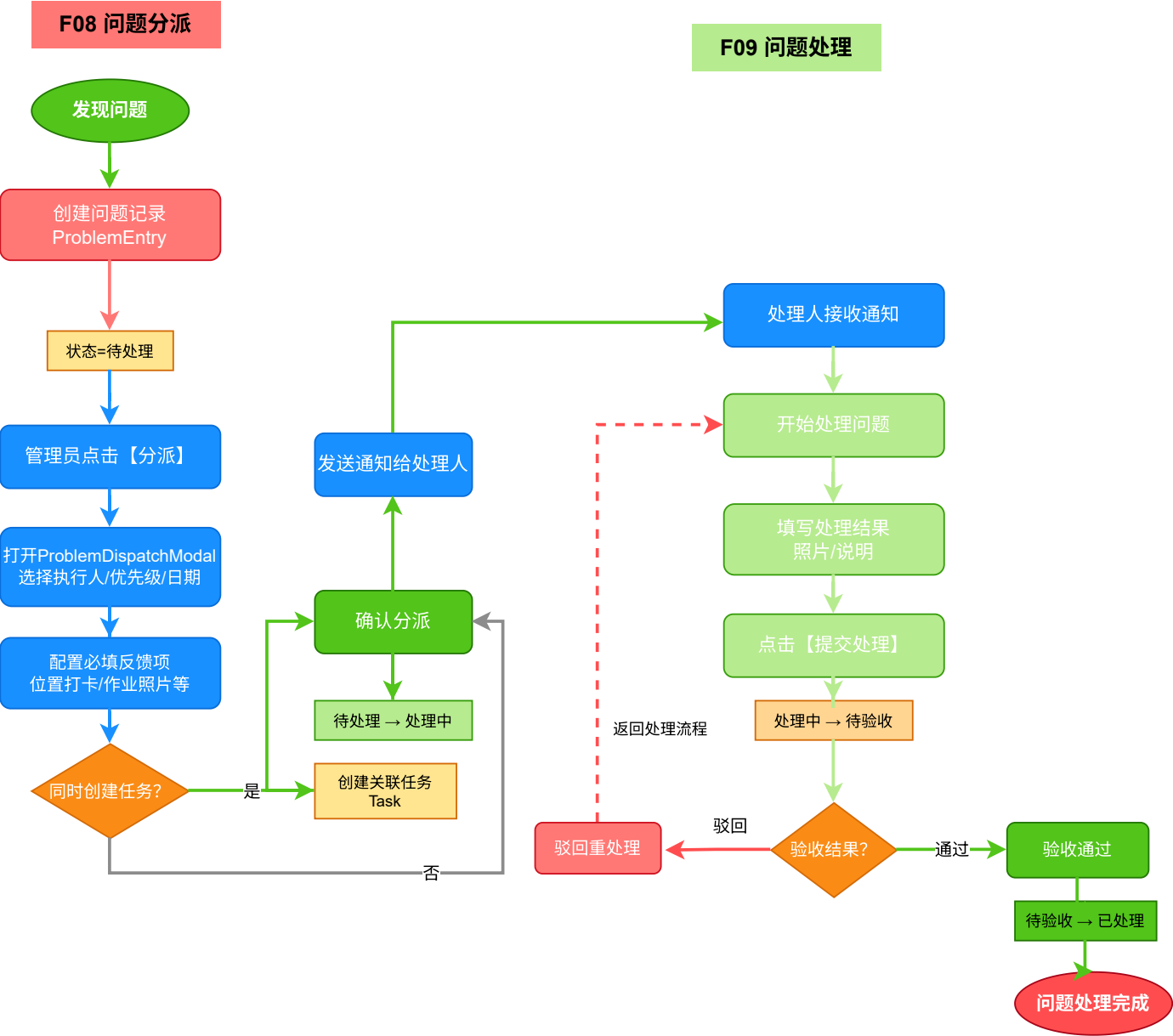
F08/F09 问题分派-处理流程图
