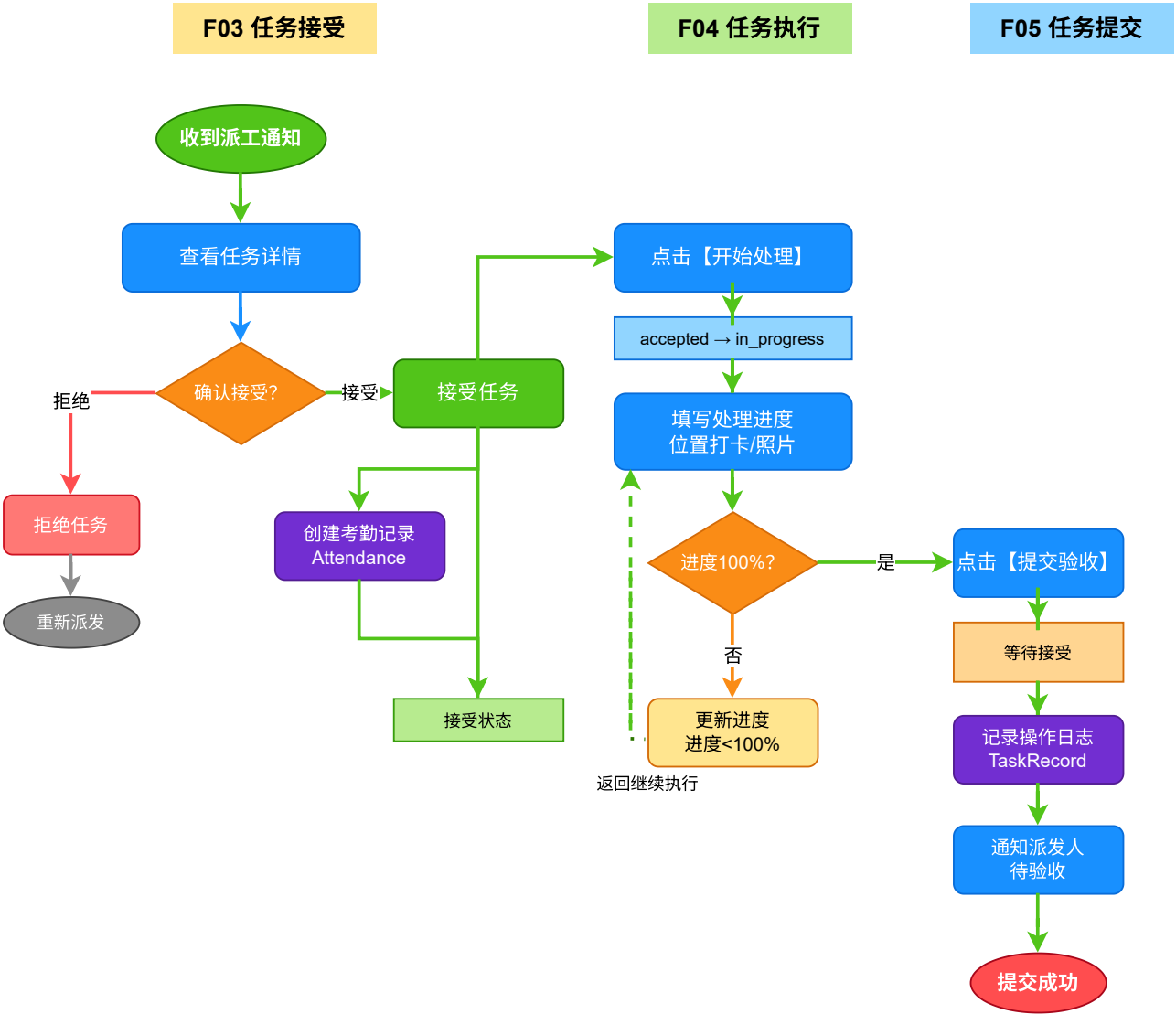
F03/F04/F05 任务接受-执行-提交流程图
