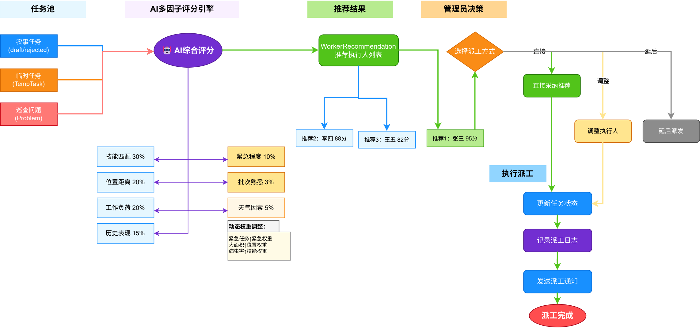
智能派工流程图（AI 7因子评分）
