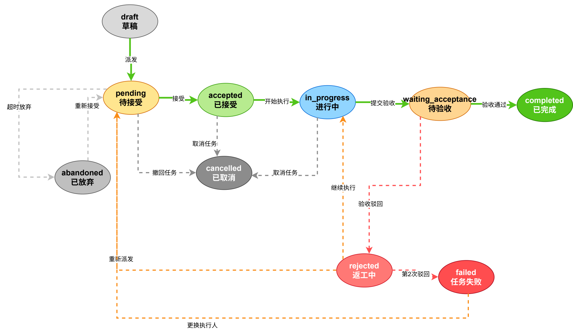
任务状态流转图（10种状态）
