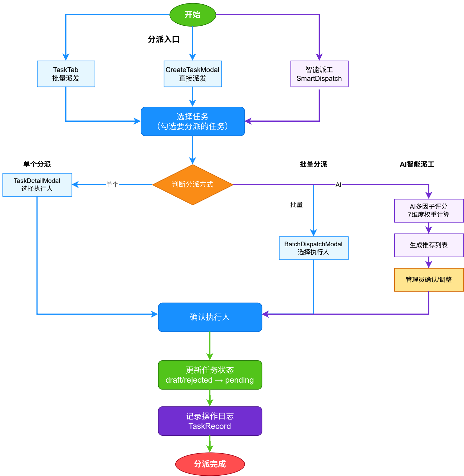
F02 任务分派流程图
