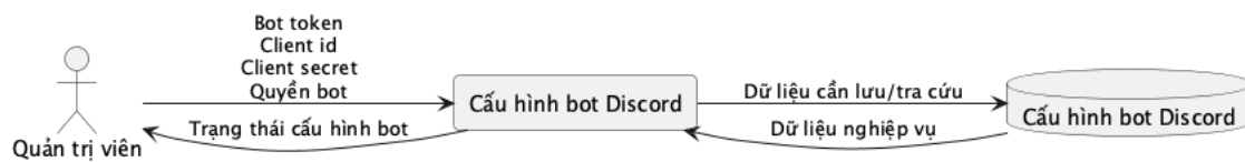
Hình 45: Sơ đồ luồng dữ liệu: undefined
