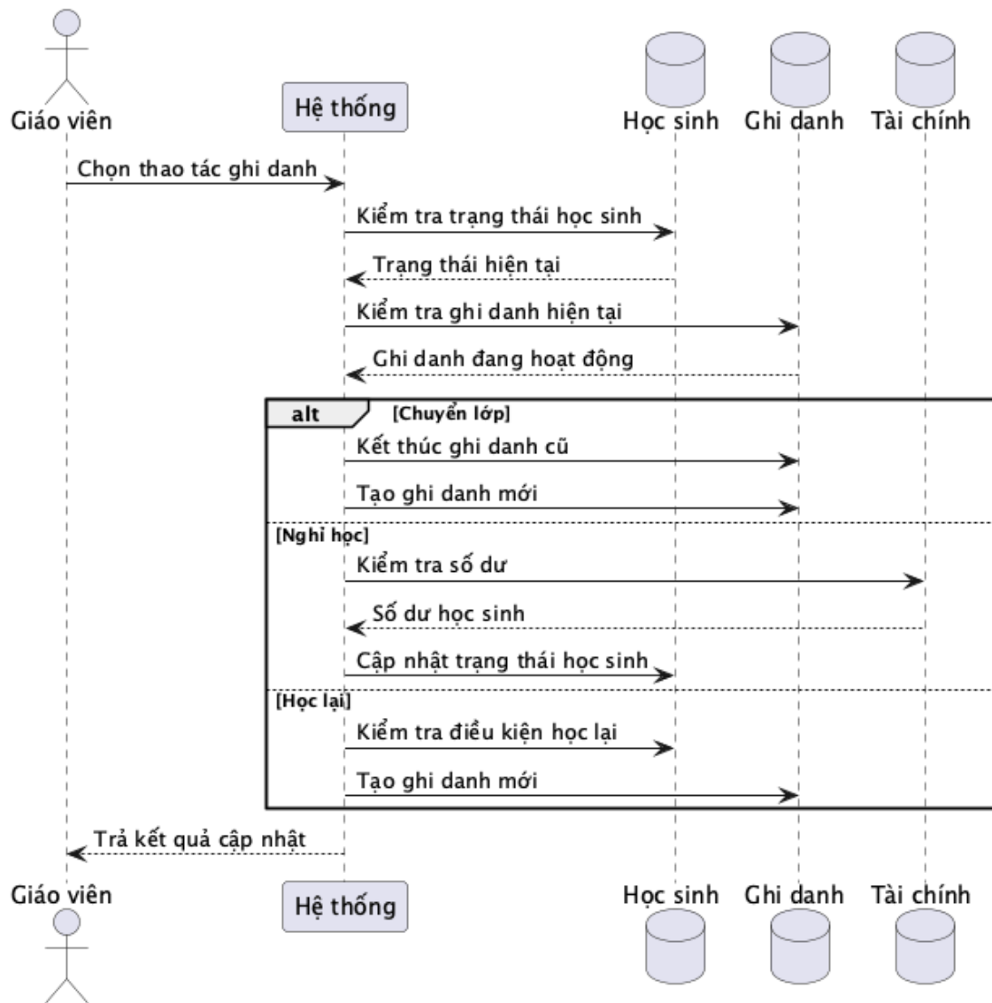
Hình 15: Sơ đồ tuần tự: undefined
