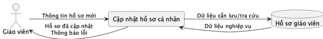
Hình 7: Sơ đồ luồng dữ liệu: undefined
