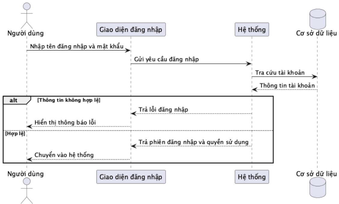
Hình 4: Sơ đồ tuần tự: undefined
