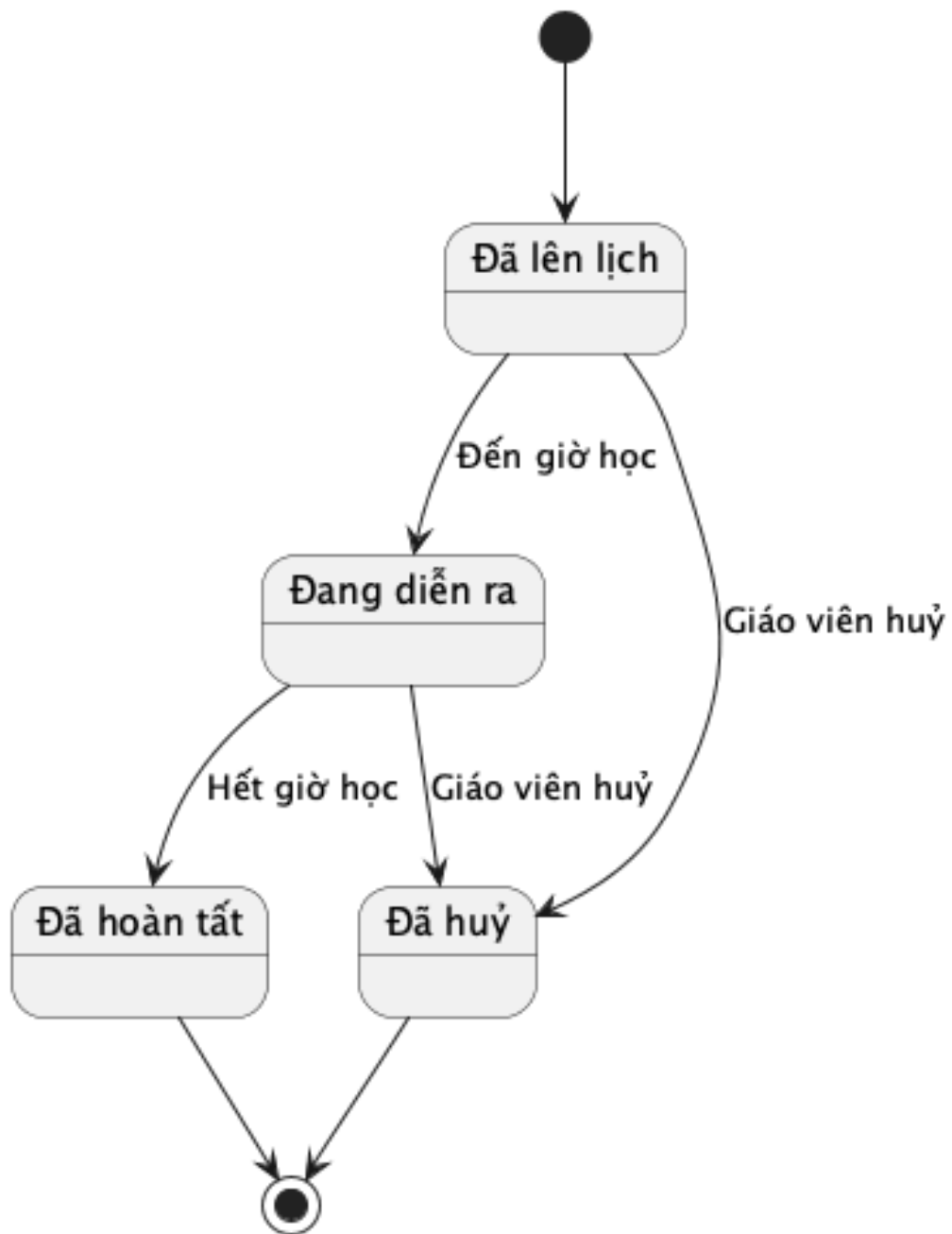
Hình 50: Sơ đồ trạng thái đối tượng Buổi học
