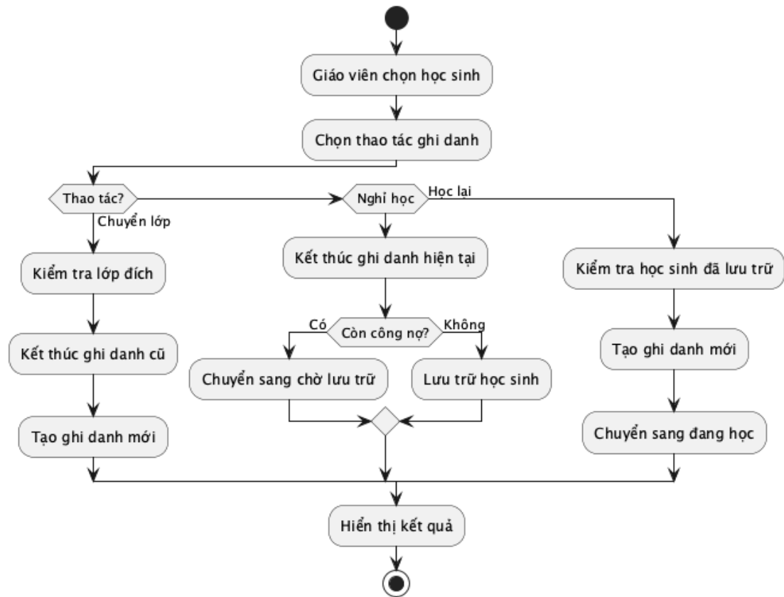
Hình 14: Sơ đồ hoạt động: undefined
