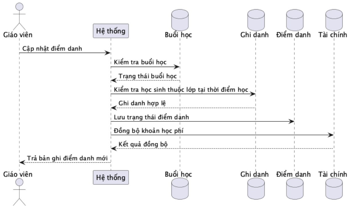
Hình 27: Sơ đồ tuần tự: undefined
