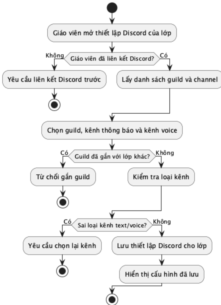
Hình 36: Sơ đồ hoạt động: undefined
