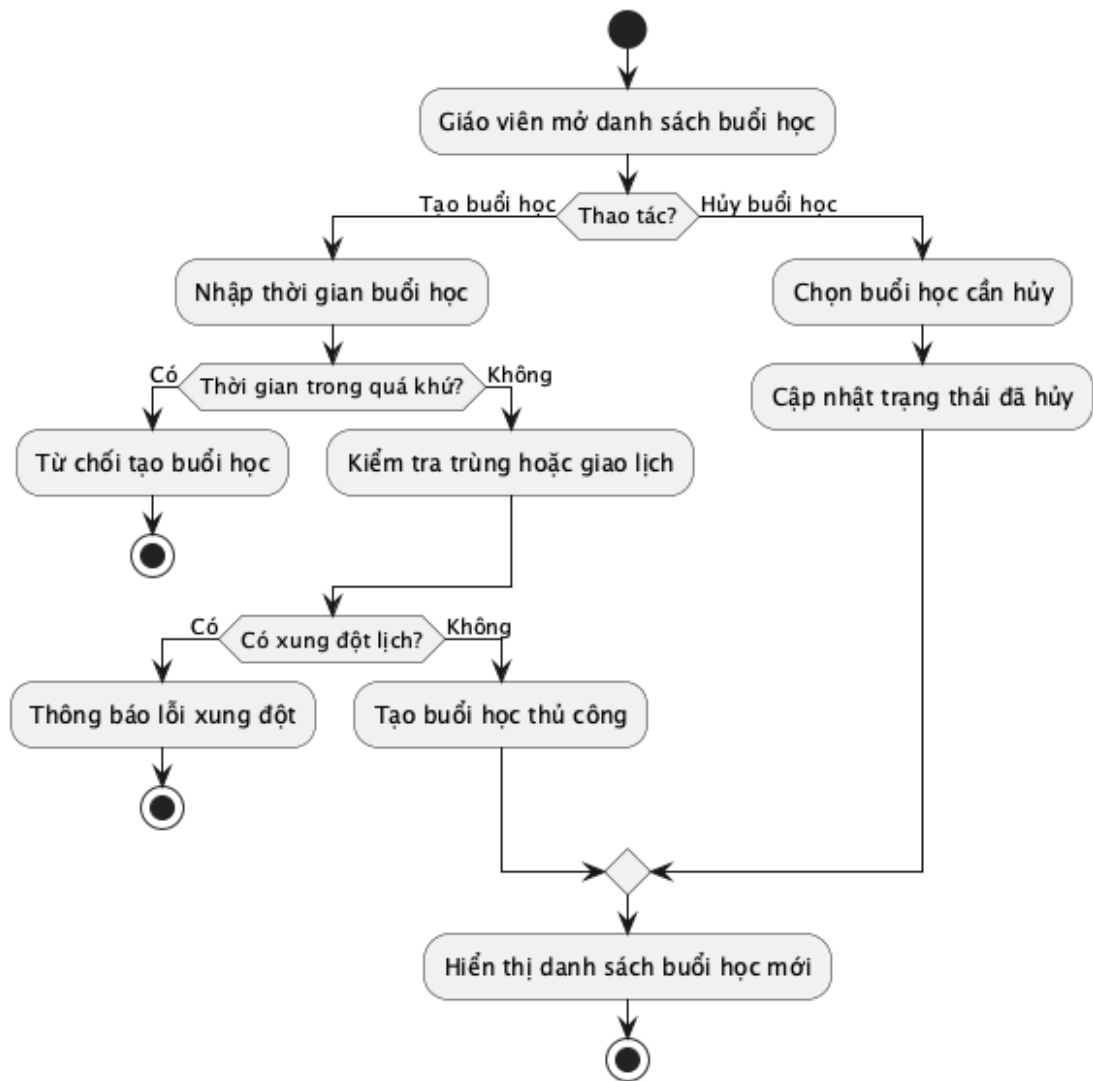
Hình 24: Sơ đồ hoạt động: undefined
