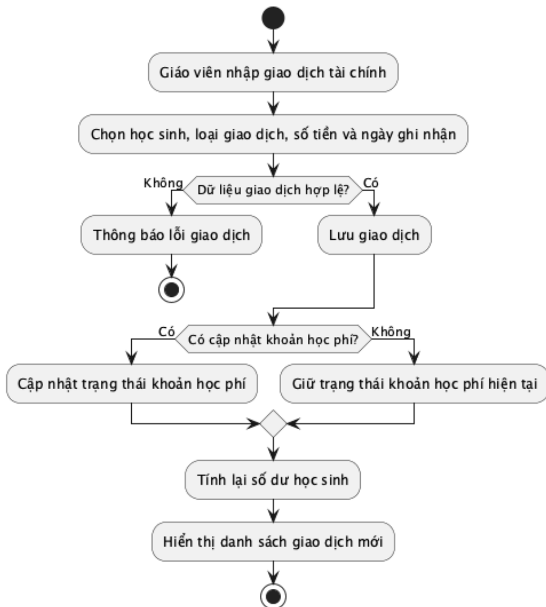
Hình 32: Sơ đồ hoạt động: undefined
