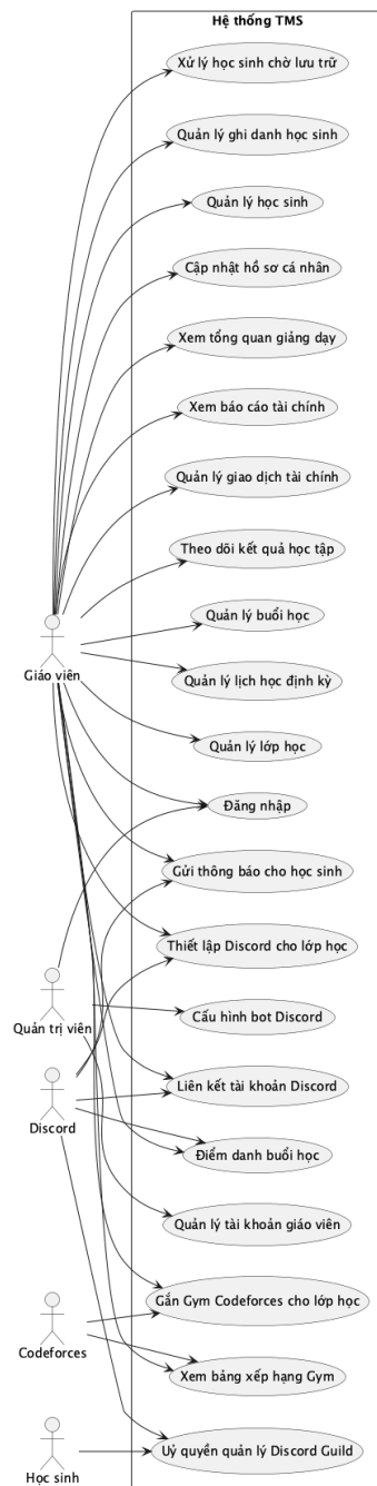
Hình 1: Sơ đồ use case tổng quan
