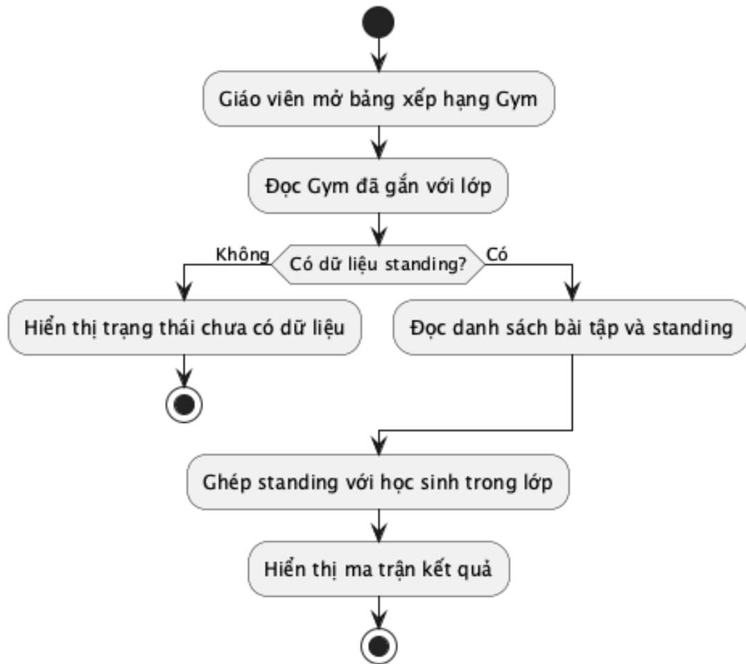
Hình 42: Sơ đồ hoạt động: undefined
