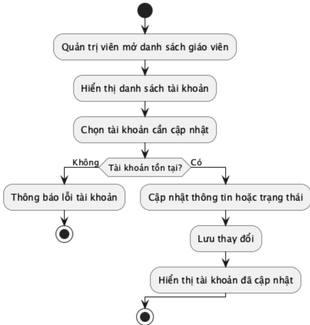
Hình 44: Sơ đồ hoạt động: undefined
