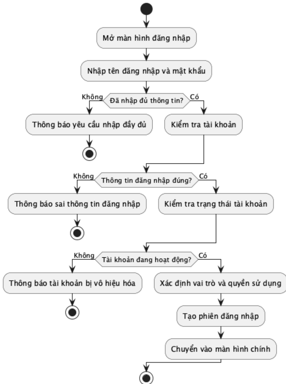
Hình 3: Sơ đồ hoạt động: undefined
