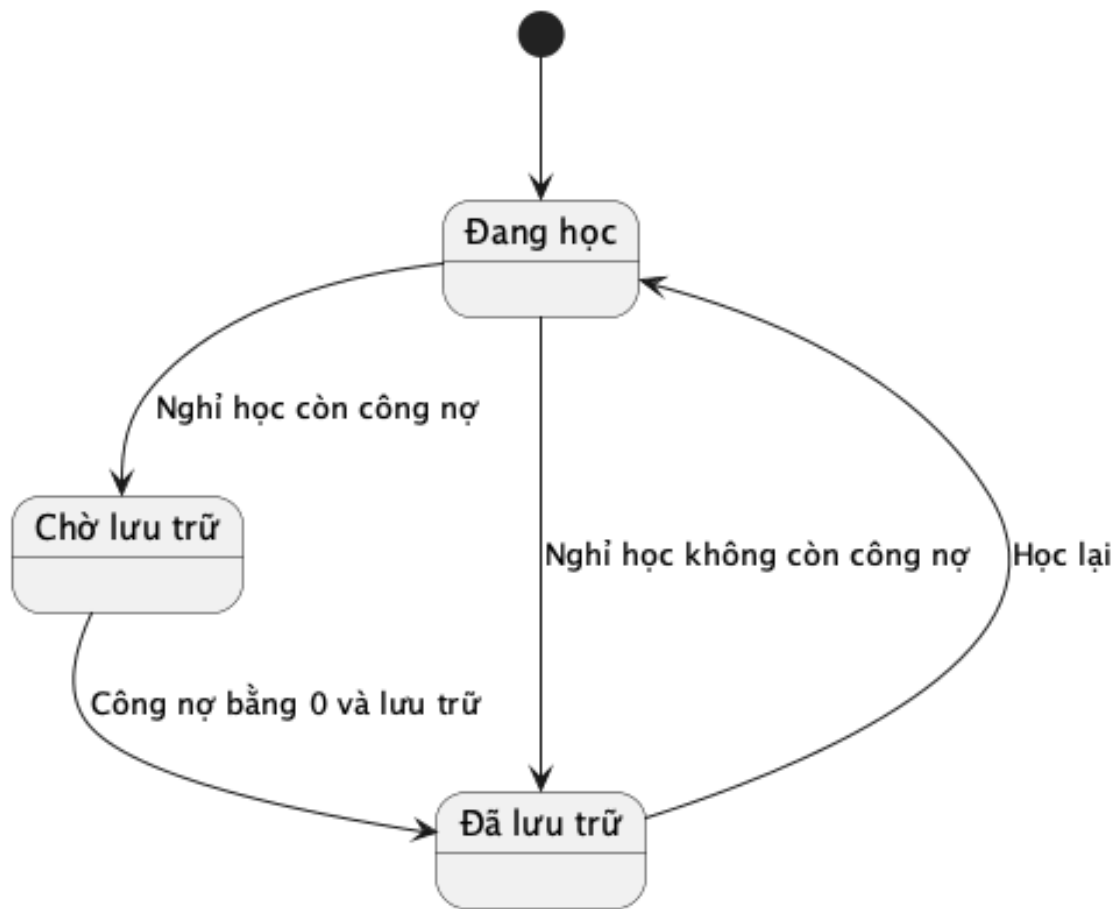
Hình 49: Sơ đồ trạng thái đối tượng Học sinh
