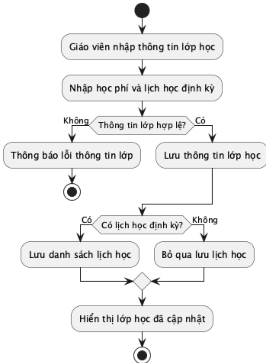
Hình 20: Sơ đồ hoạt động: undefined
