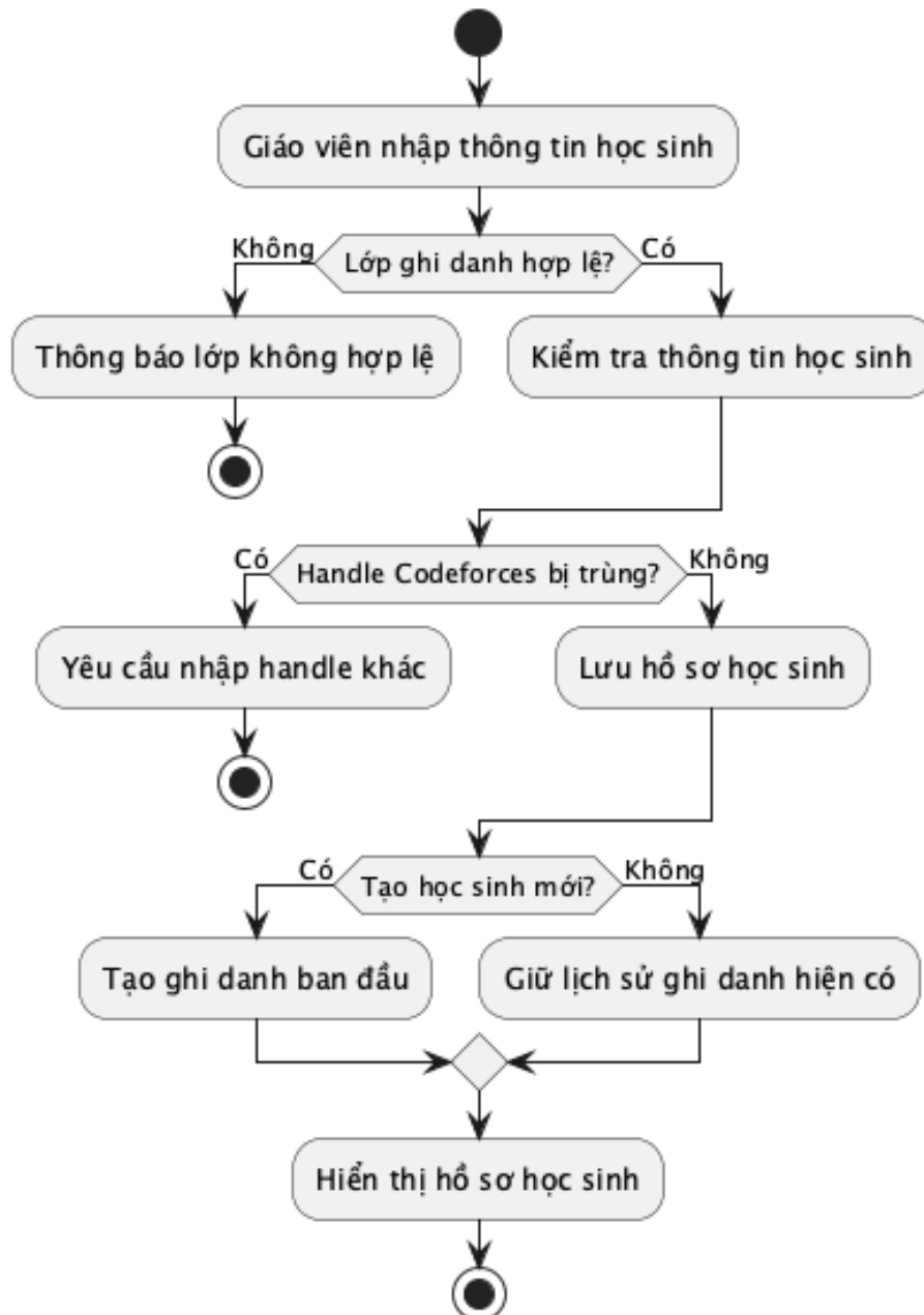
Hình 12: Sơ đồ hoạt động: undefined
