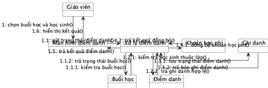
Hình 28: Sơ đồ cộng tác: undefined
