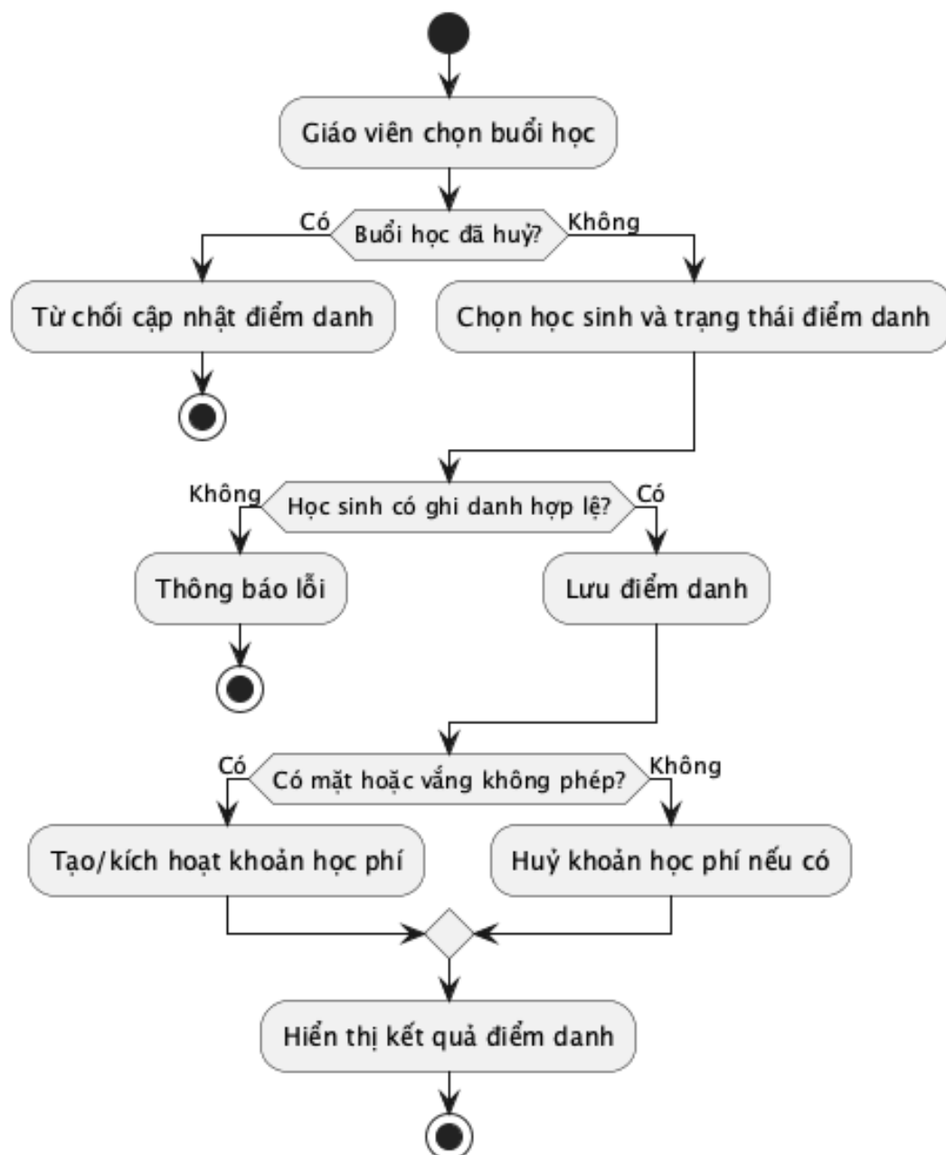
Hình 26: Sơ đồ hoạt động: undefined
