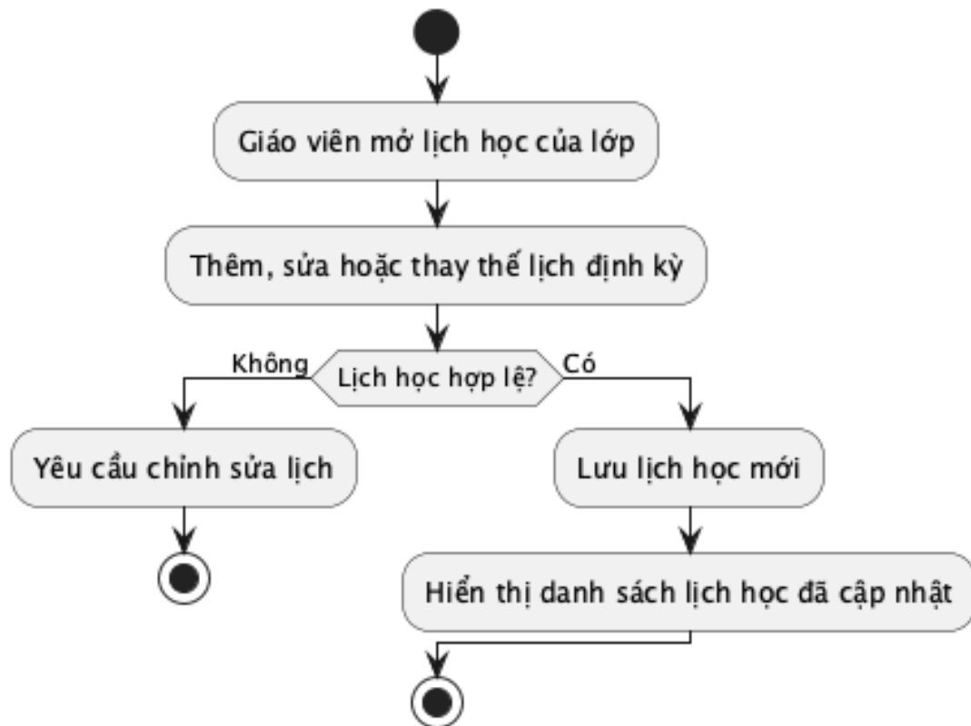
Hình 22: Sơ đồ hoạt động: undefined
