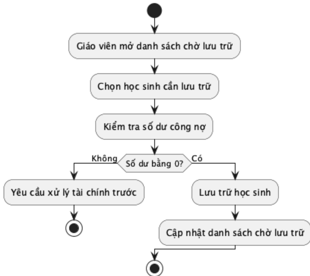
Hình 18: Sơ đồ hoạt động: undefined
