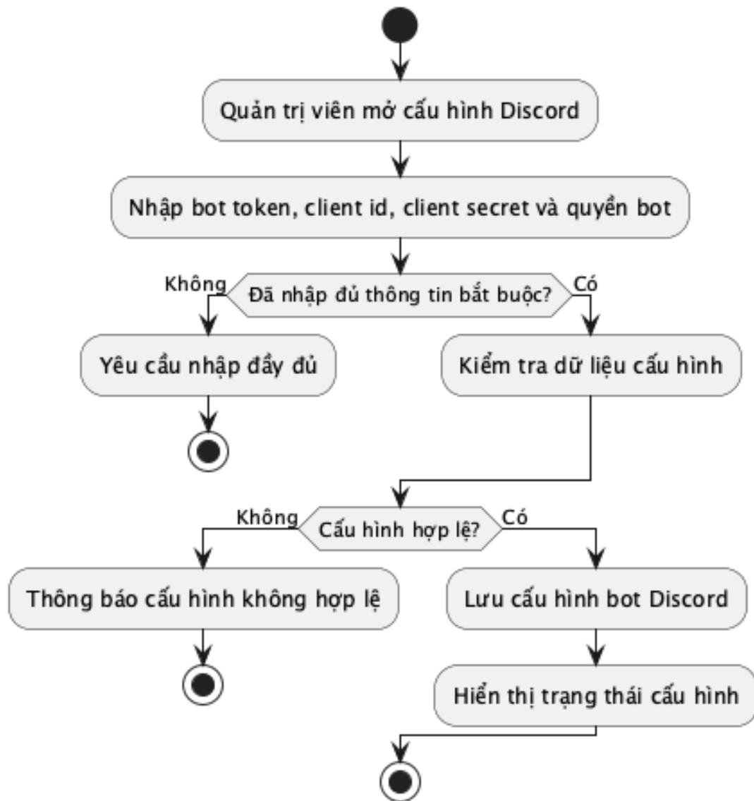
Hình 46: Sơ đồ hoạt động: undefined
