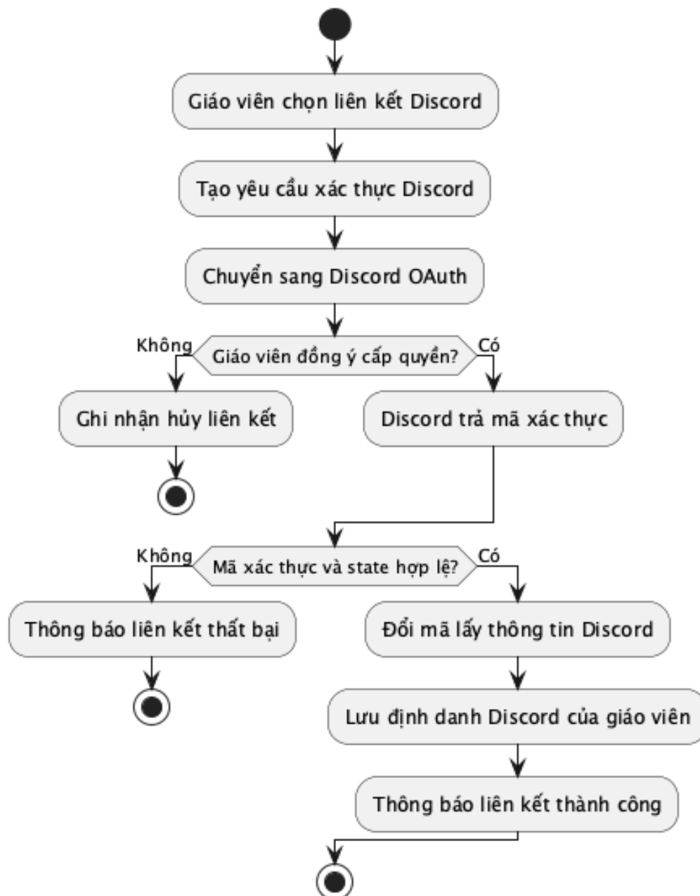
Hình 10: Sơ đồ hoạt động: undefined
