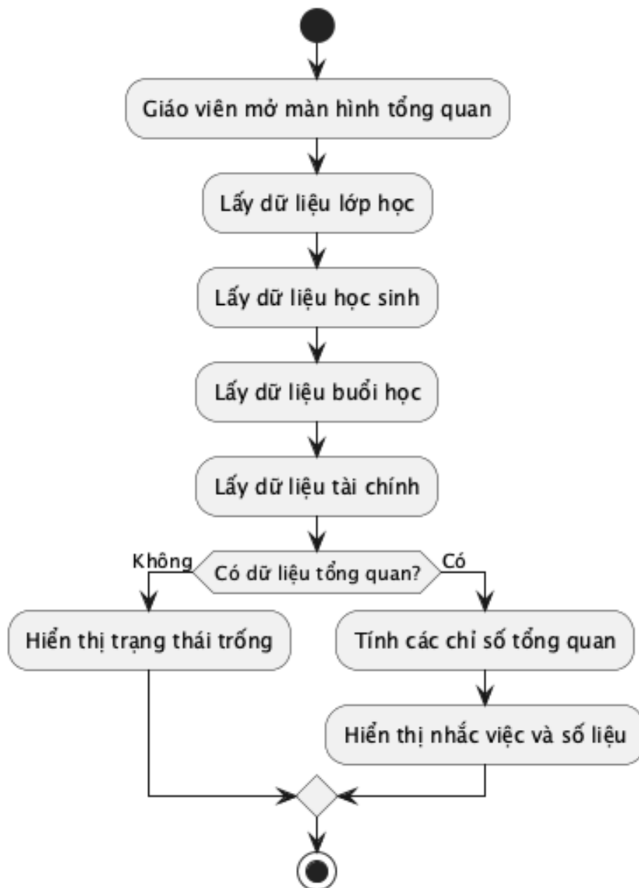
Hình 6: Sơ đồ hoạt động: undefined
