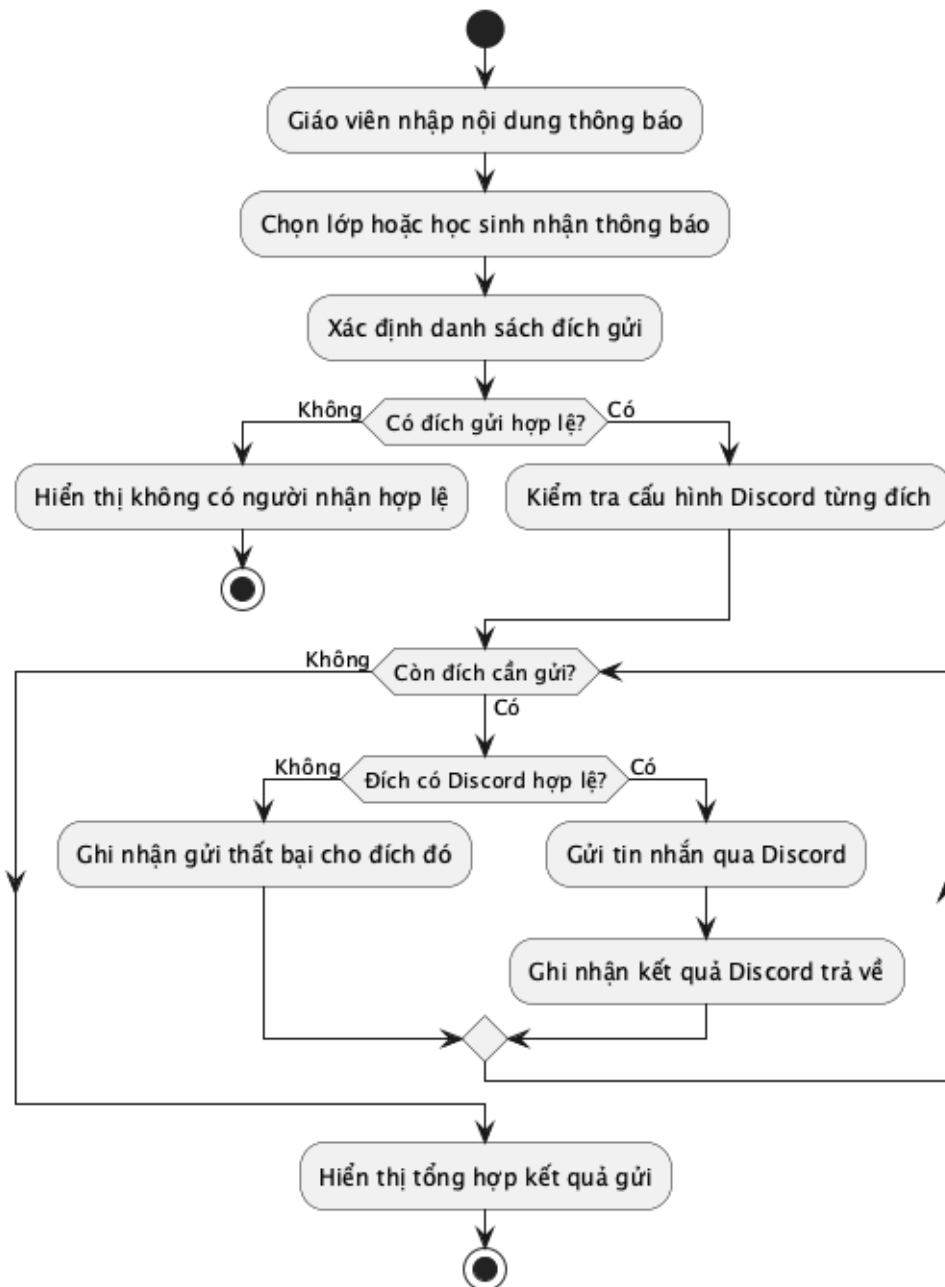
Hình 38: Sơ đồ hoạt động: undefined
