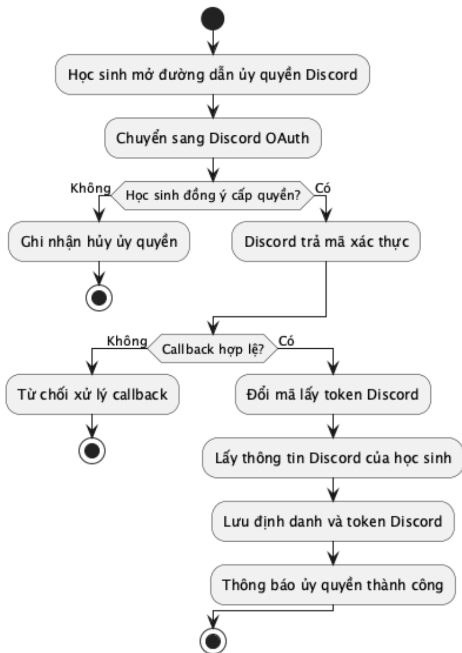
Hình 48: Sơ đồ hoạt động: undefined
