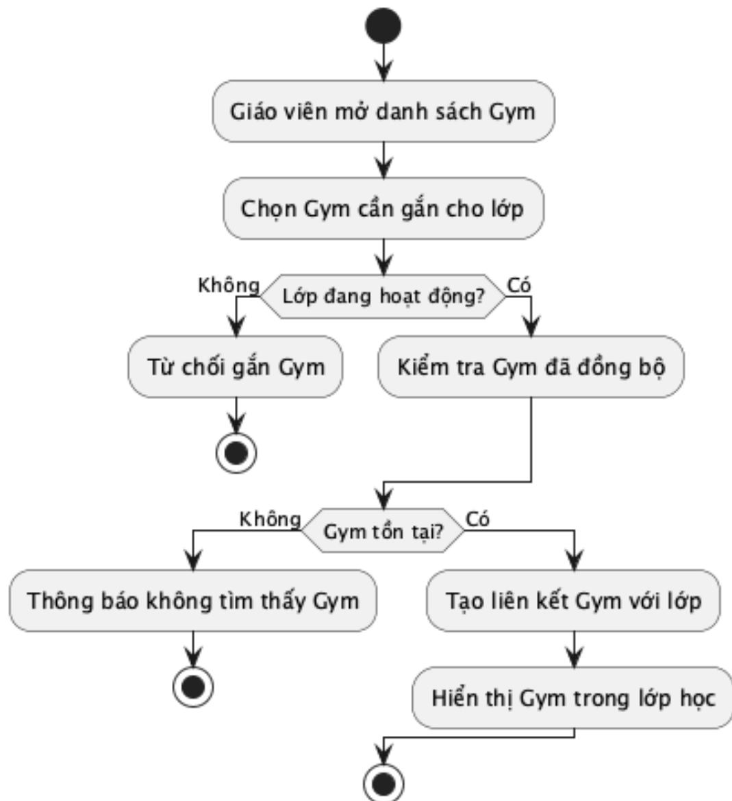
Hình 40: Sơ đồ hoạt động: undefined
