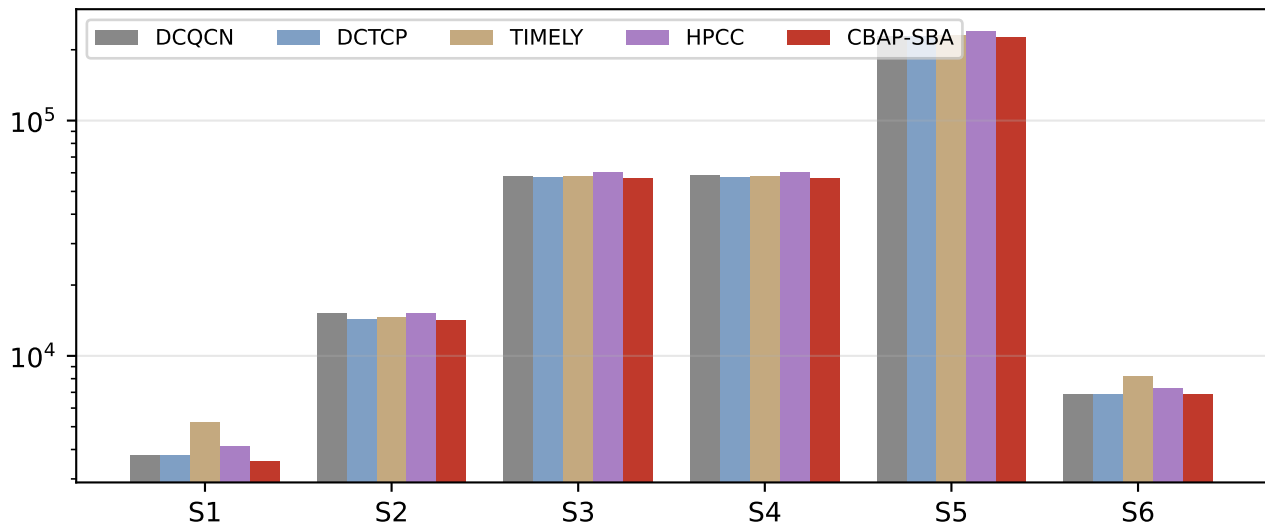
FCT p99 (us)
