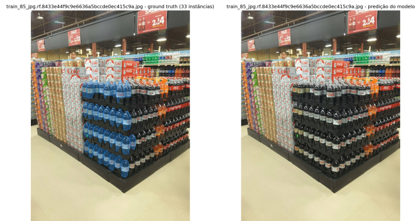
Figura 7: ground truth (esquerda) e predição v1 (direita) em train_85.jpg ...: falso negativo total para bebidas .
