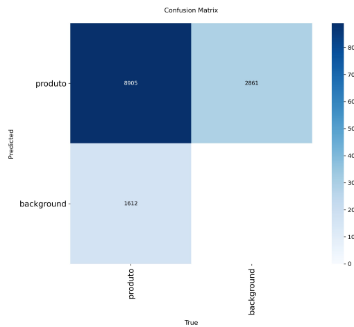
Figura 4: matriz de confusão da detecção no teste.
