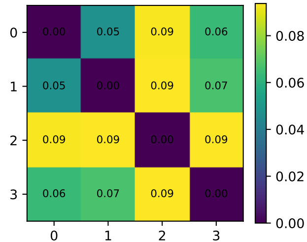
D1 cosine distance qid=10203
