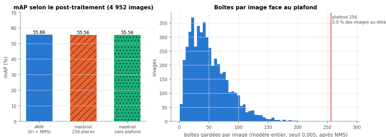
Figure 22 (hw_postproc): mAP avec le post-traitement matériel, avec et sans plafond de boîtes, et nombre de boîtes par image face au plafond.
