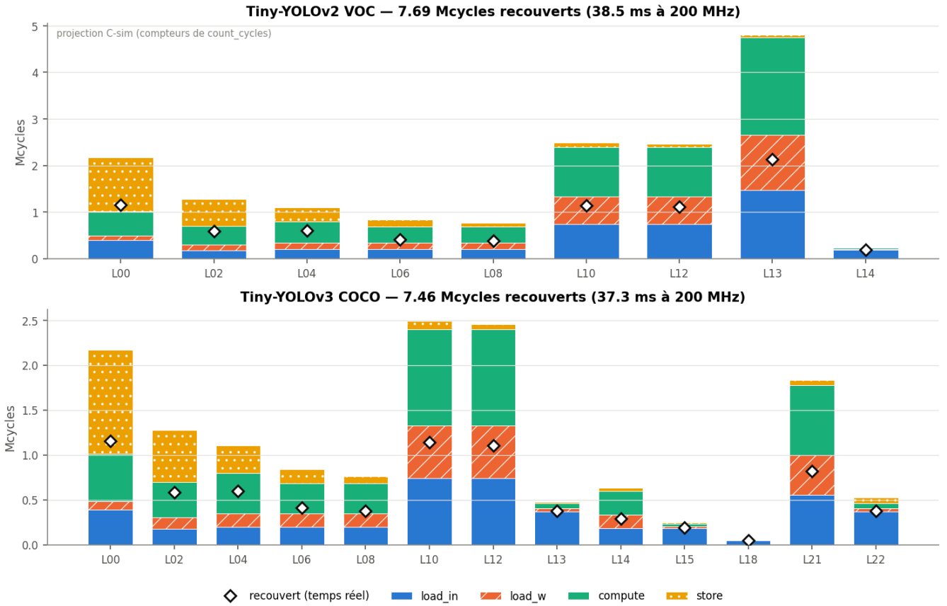
Figure 19 (cycles_couches): Cycles par couche du noyau actuel, décomposés en chargements, calcul et stockage ; le losange donne le temps réel avec recouvrement.
