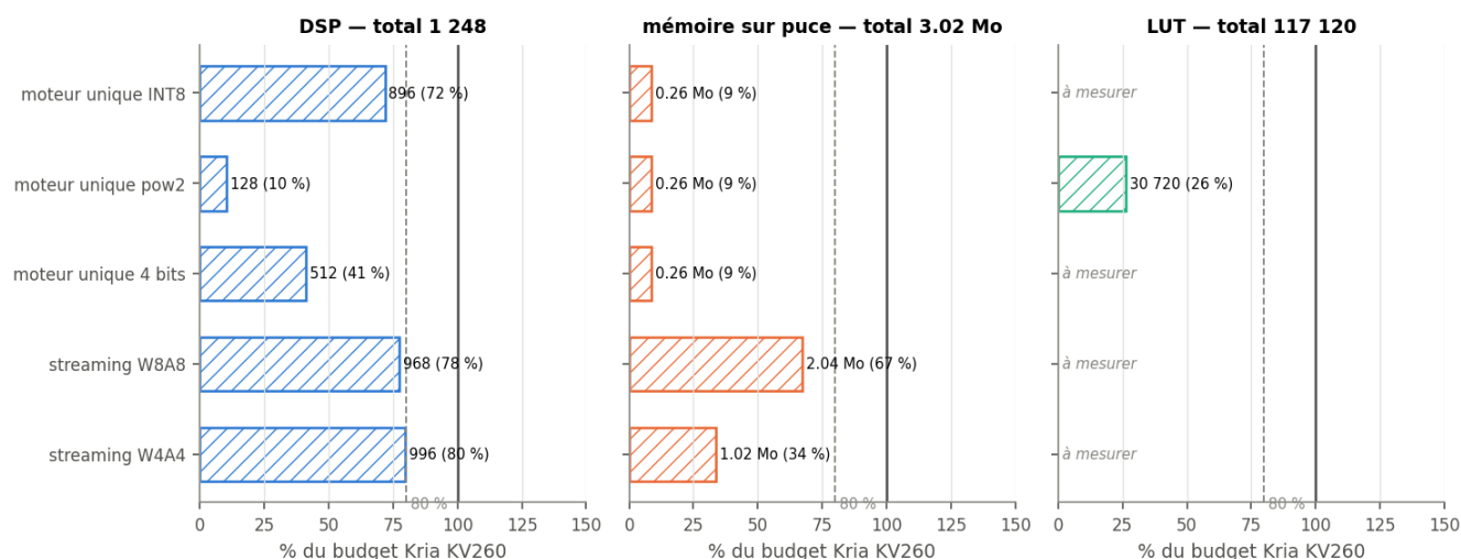
Figure 21 (ressources): DSP, mémoire sur puce et LUT des architectures (moteur unique INT8, pow2 et 4 bits, streaming) face au budget de la KV260 ; hachuré : estimation, plein : synthèse.
