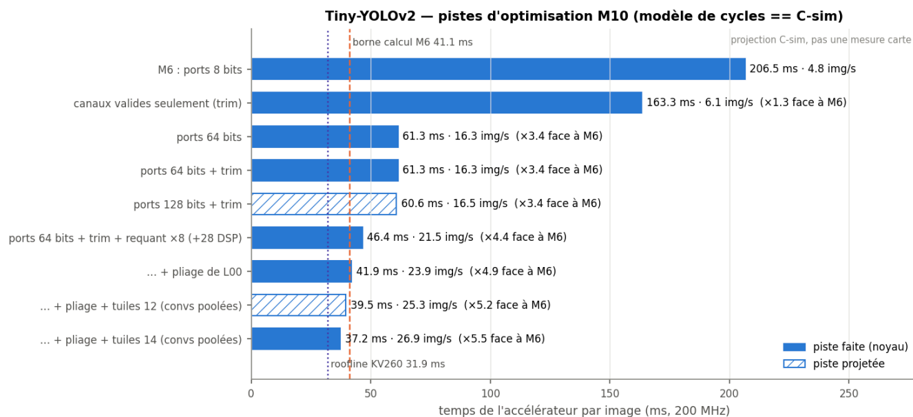
Figure 17 (cascade_m10): Temps par image de Tiny-YOLOv2 à chaque piste d'optimisation M10, face à la borne de calcul et au roofline KV260.
