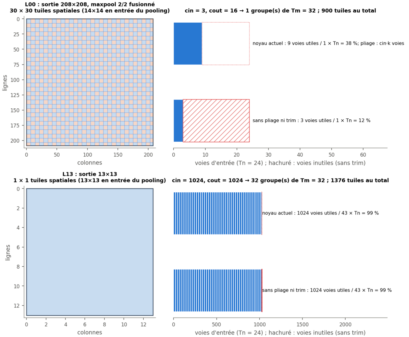
Figure 15 (tuilage): Tuilage de deux couches : tuiles spatiales et voies d'entrée, avec le pliage de L00 (cin = 3) et la couche 13×13 couverte par une seule tuile.
