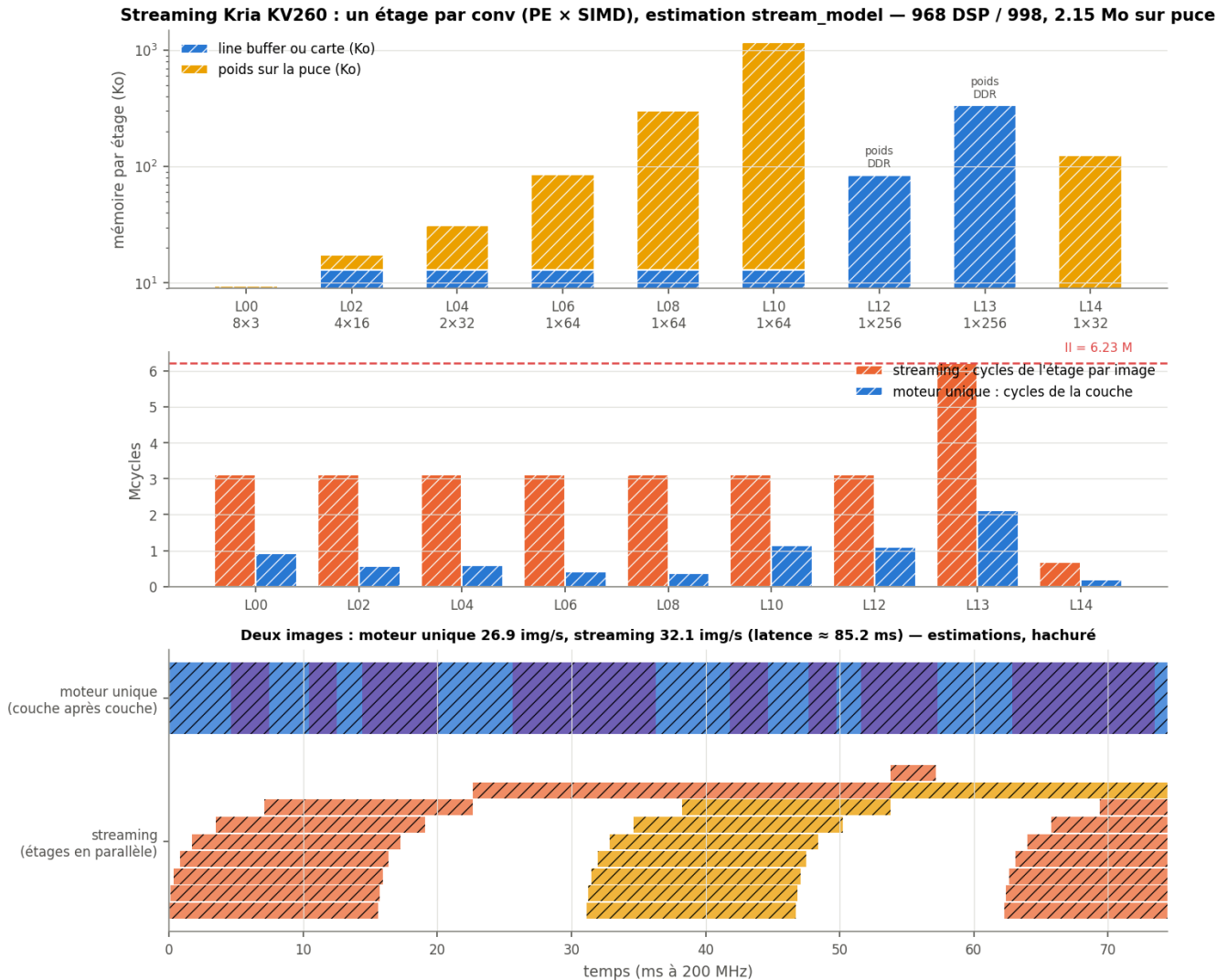
Figure 24 (streaming): Architecture streaming face au moteur unique : mémoire et parallélisme par étage, cycles par couche, chronogramme sur deux images (estimations).
