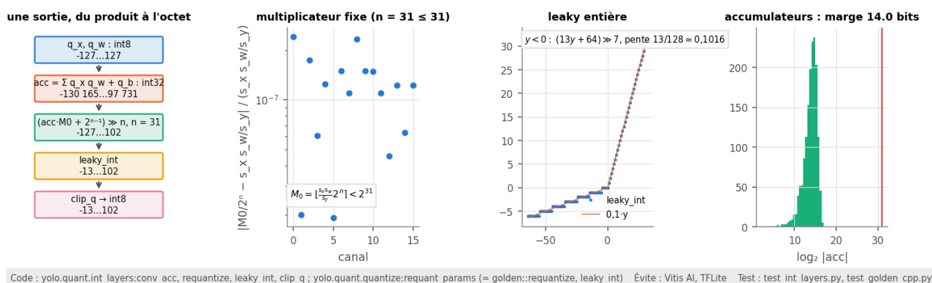
Figure 10 (entier): Arithmétique entière du matériel : chaîne d'une sortie, multiplicateur fixe M_0/2^n , leaky entière 13/128 et marge des accumulateurs int32.
