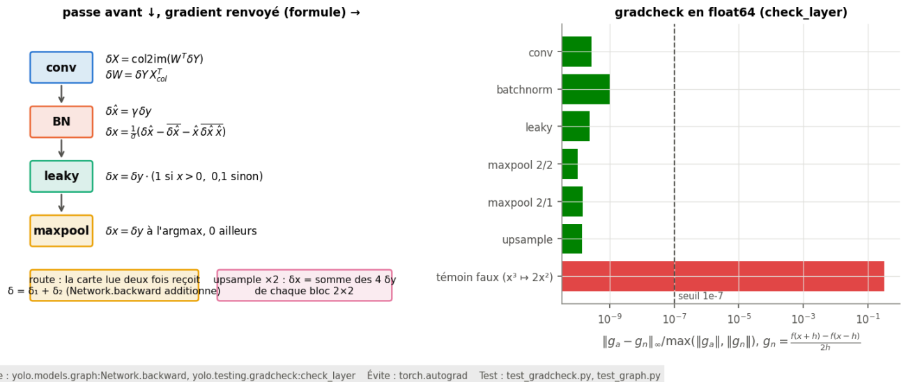
Figure 5 (retropropagation): Rétropropagation écrite à la main : formule du gradient renvoyé par chaque couche, puis l'erreur du gradcheck par couche face au seuil 1e-7 .
