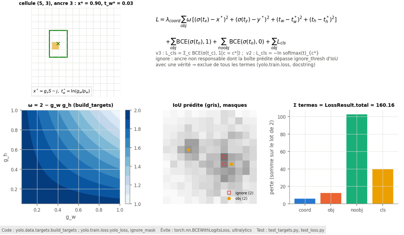
Figure 6 (perte): Cibles et perte YOLO : encodage d'une vérité, la perte terme par terme, le poids \omega = 2 - g_w g_h , le masque ignore et la part de chaque terme sur un lot.
