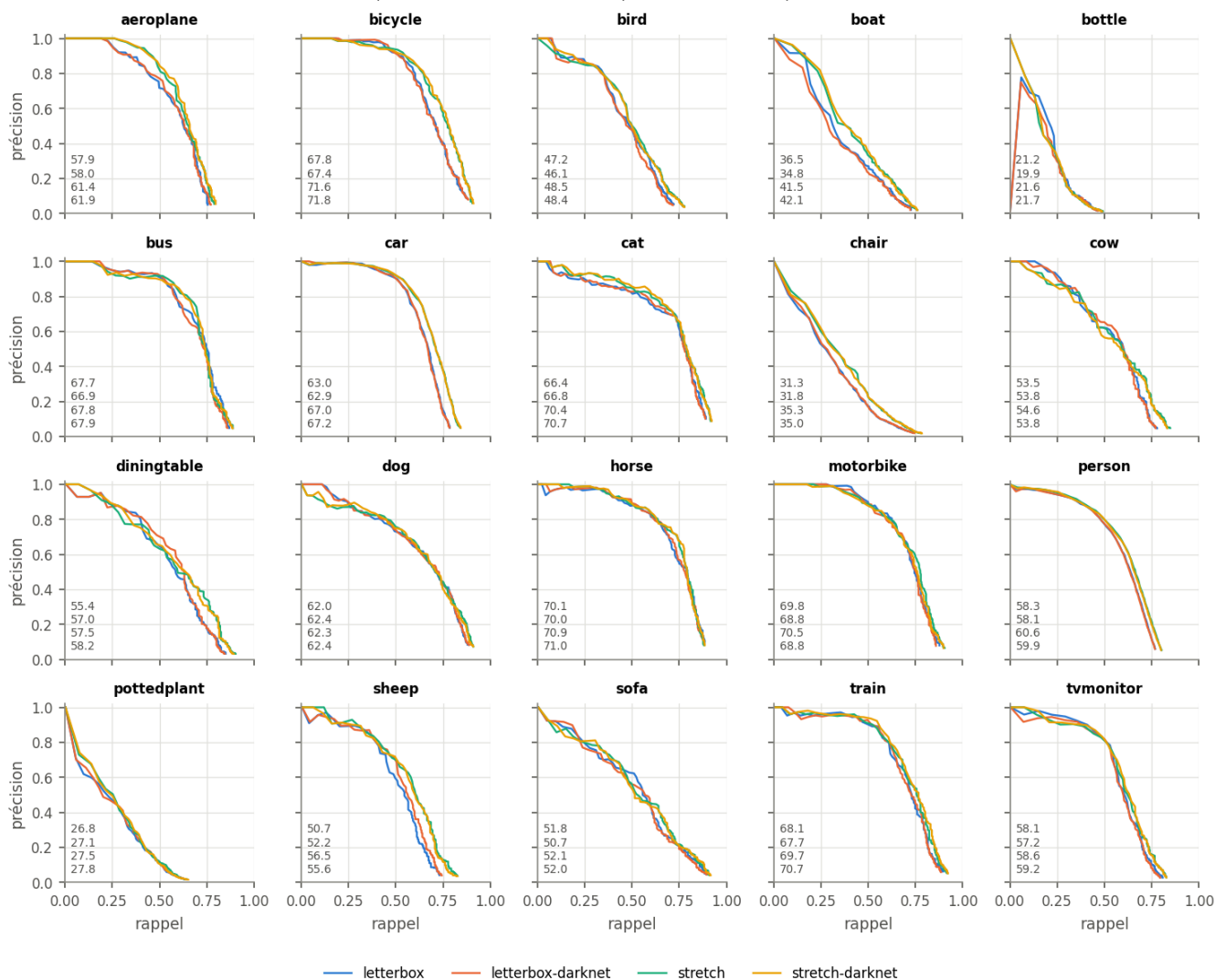
Figure 7 (pr): Courbes précision-rappel par classe (11 points VOC07) pour chaque prétraitement évalué, puis les quatre superposées.
