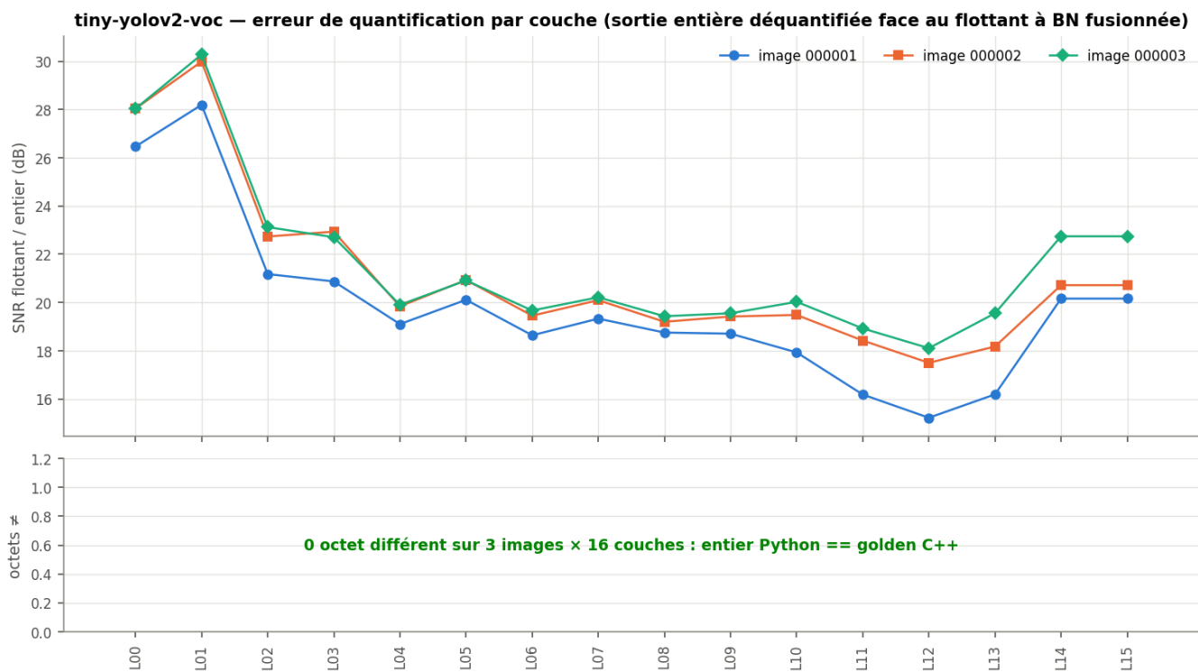
Figure 12 (erreur_couches): SNR par couche entre le flottant et l'entier déquantifié, et écart entier Python ↔ golden C++ (0 partout : bit-exact).
