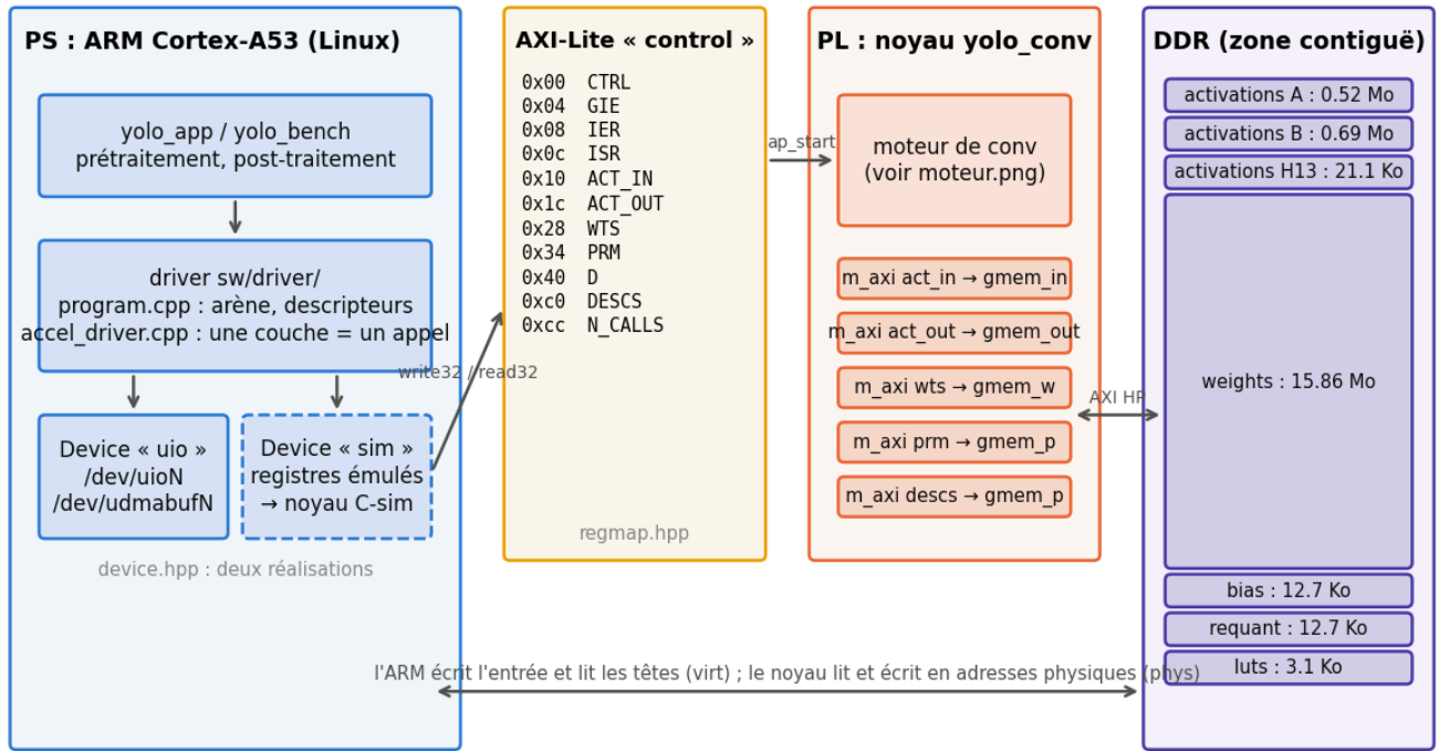
Figure 16 (soc): Schéma du SoC : application et driver sur l'ARM, registres AXI-Lite, ports m_axi du noyau et découpage de l'arène DDR.
