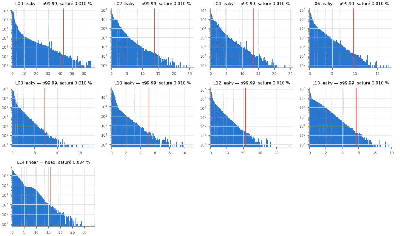
tiny-yolov2-voc — |activations| (log) et seuil de saturation retenu 127-s (rouge) ; candidats en pointillé
