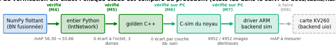
Figure 13 (chaîne_verif): Chaîne de vérification bit-exact, du flottant NumPy à la carte : critère et état de chaque passage.
