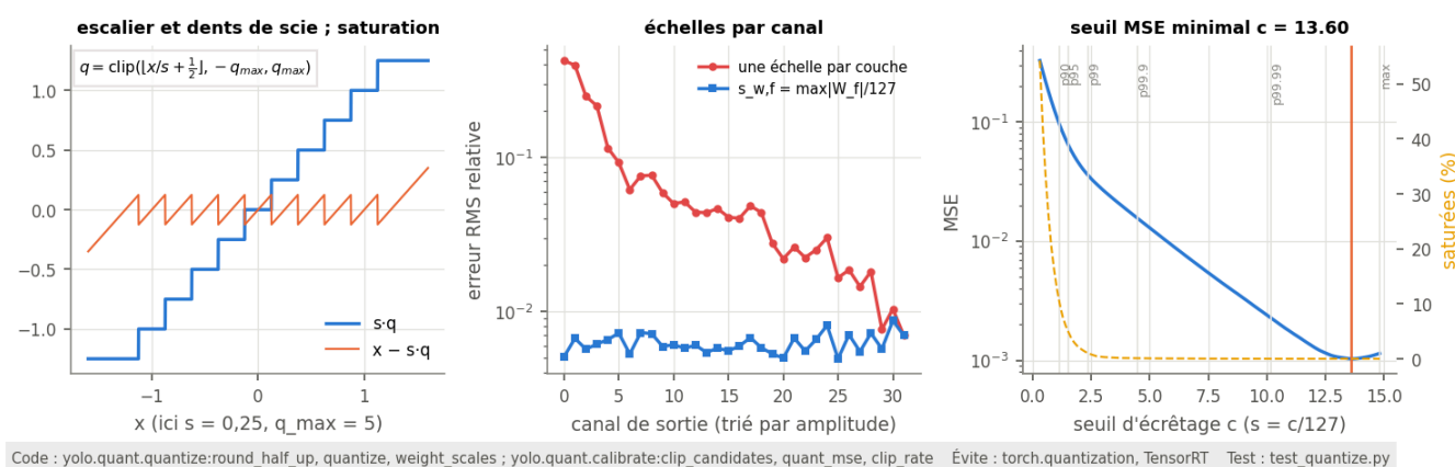
Figure 9 (quantification): Quantification symétrique : l'escalier et son erreur, échelles par canal face à une échelle par couche, choix du seuil d'écrapage par la MSE.
