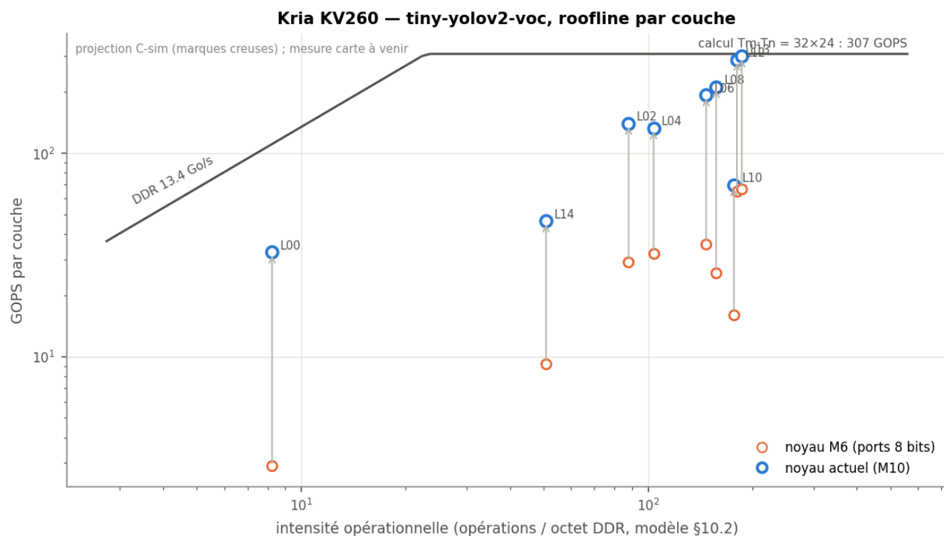
Figure 18 (roofline_couches): Roofline KV260 avec un point par couche de Tiny-YOLOv2, avant et après les optimisations M10.
