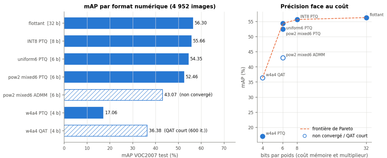
Figure 23 (map_formats): mAP de Tiny-YOLOv2 selon le format des poids (flottant, INT8, puissances de 2, 4 bits), et frontière précision / bits.
