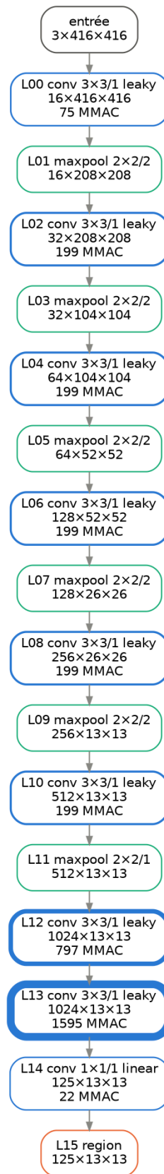
Figure 2 (graphe): Graphe couche par couche (type, noyau et stride, forme de sortie C \times H \times W ; bord épais = beaucoup de MACs).
