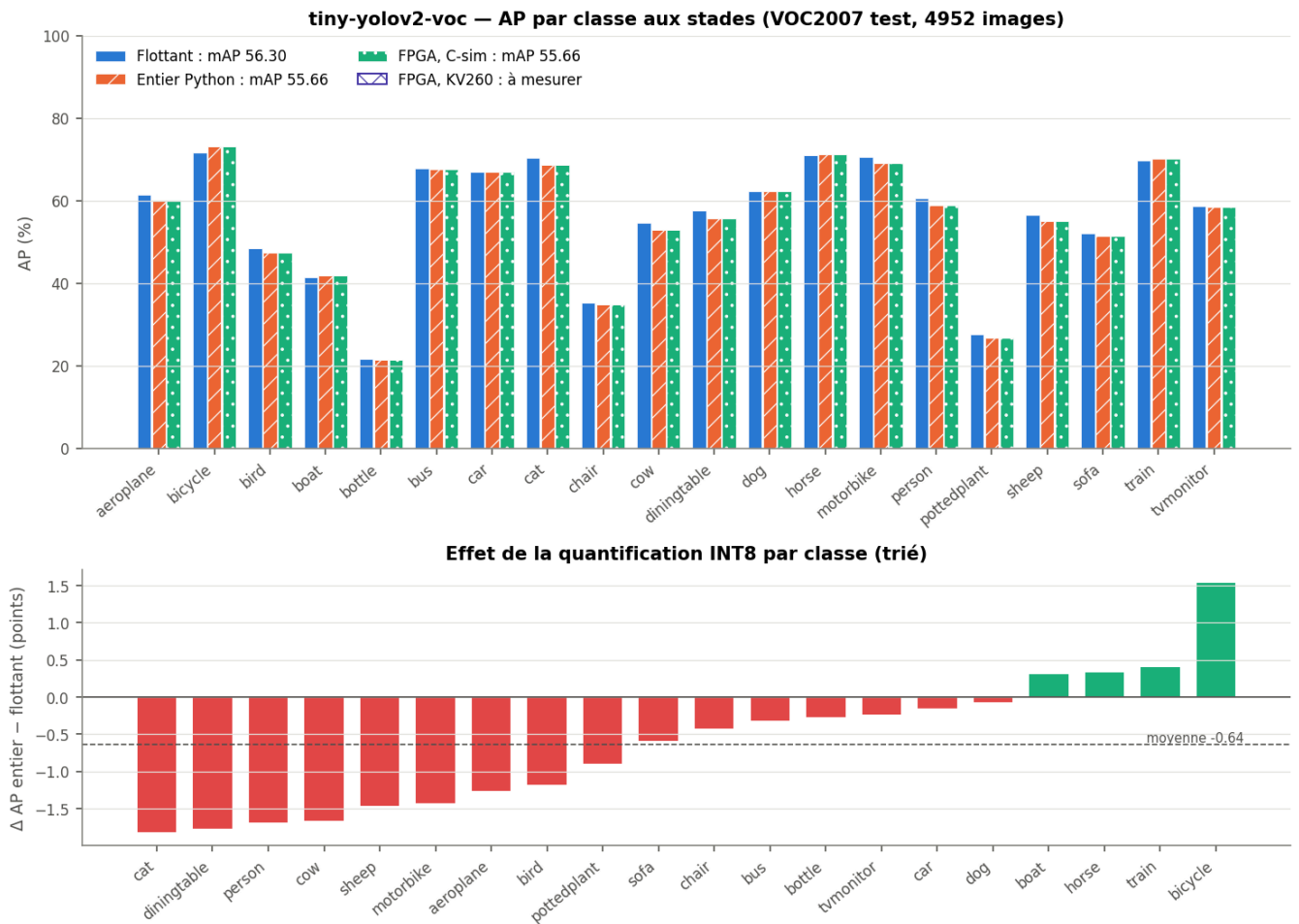
Figure 20 ( map_stades ): AP par classe aux stades flottant, entier et C-sim (la carte quand elle sera mesurée), et écart entier – flottant trié.
