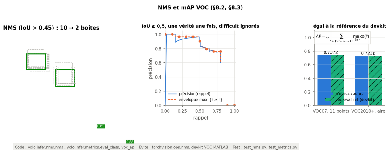
Figure 8: NMS pas à pas, appariement détections / vérités et courbe précision-rappel, AP VOC07 sur 11 points face à l'aire sous l'enveloppe, égale à la référence du devkit. (nms_map)
