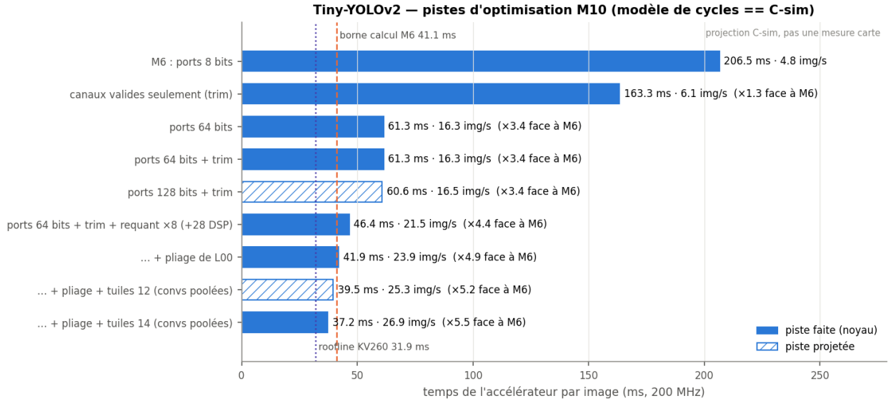
Figure 17: Temps par image de Tiny-YOLOv2 à chaque piste d'optimisation M10, face à la borne de calcul et au roofline KV260. (cascade_m10)
