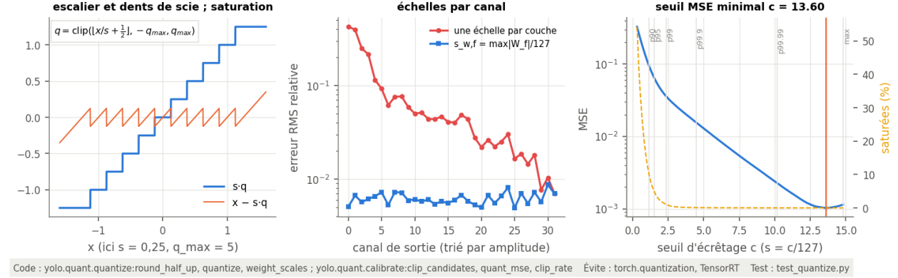
Figure 9: Quantification symétrique : l’escalier et son erreur, échelles par canal face à une échelle par couche, choix du seuil d’écrouissage par la MSE. (quantification)
