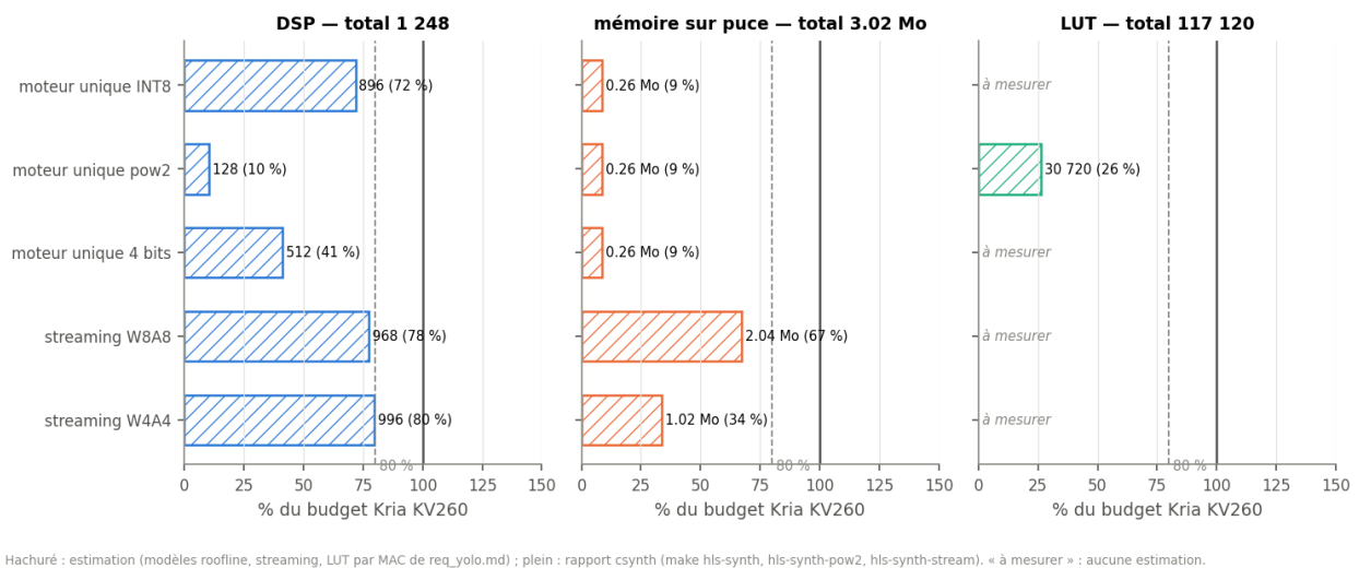
Figure 21: DSP, mémoire sur puce et LUT des architectures (moteur unique INT8, pow2 et 4 bits, streaming) face au budget de la KV260 ; hachuré : estimation, plein : synthèse. (ressources)
