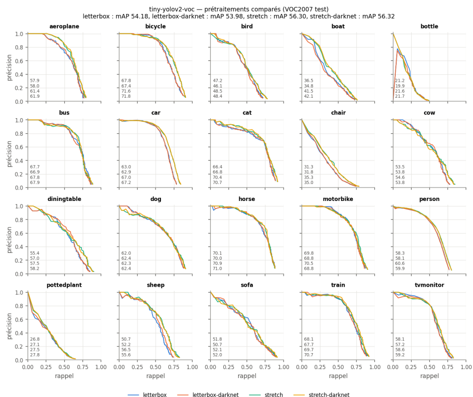
Figure 7: Courbes précision-rappel par classe (11 points VOC07) pour chaque prétraitement évalué, puis les quatre superposées. (pr)
