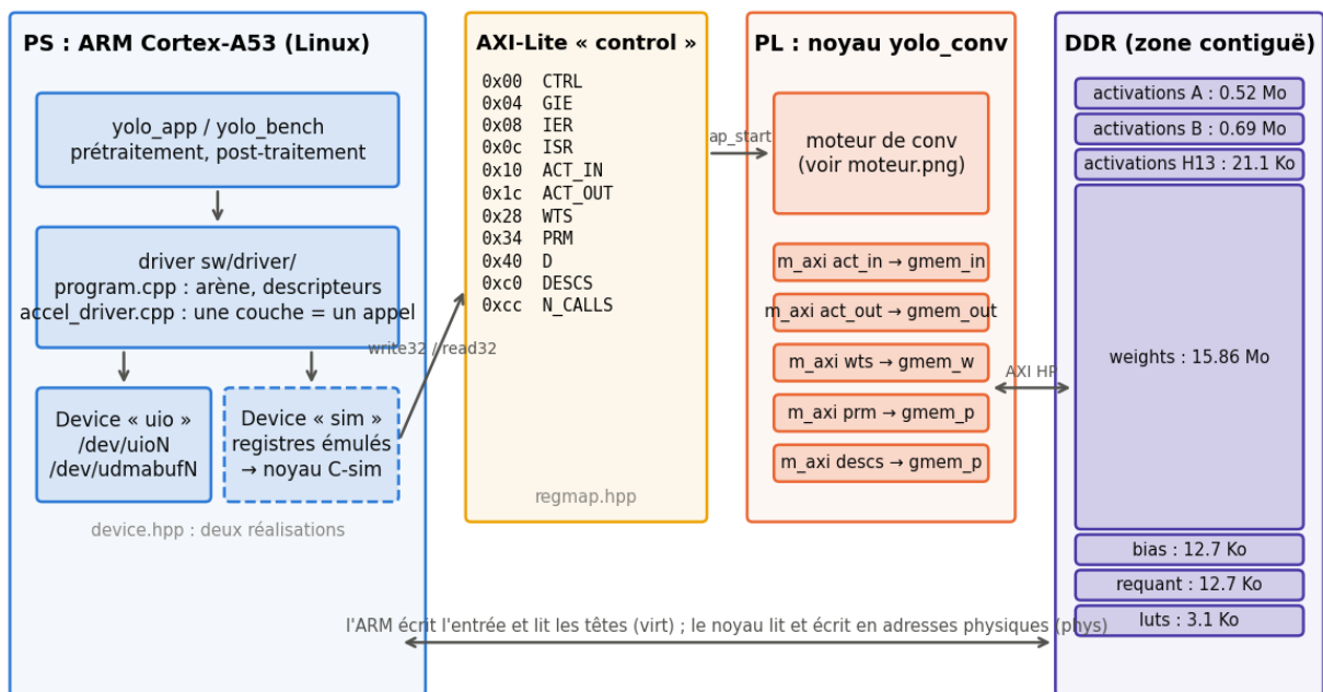
Figure 16: Schéma du SoC : application et driver sur l'ARM, registres AXI-Lite, ports m_axi du noyau et découpage de l'arène DDR. (soc)
