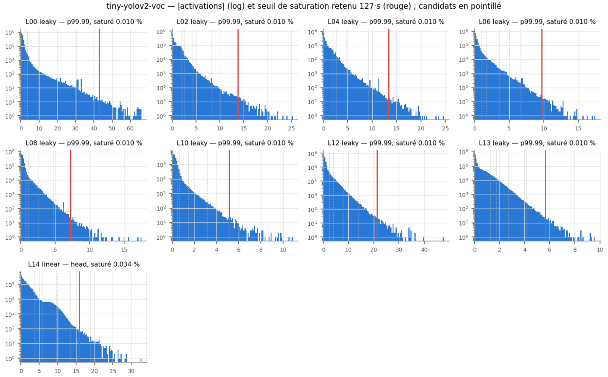
Figure 11: Distribution des activations par couche et seuil de saturation retenu par la calibration ; échelles des poids par canal. (calibration)
