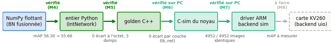
Figure 13: Chaîne de vérification bit-exact, du flottant NumPy à la carte : critère et état de chaque passage. ( chaîne_verif )
