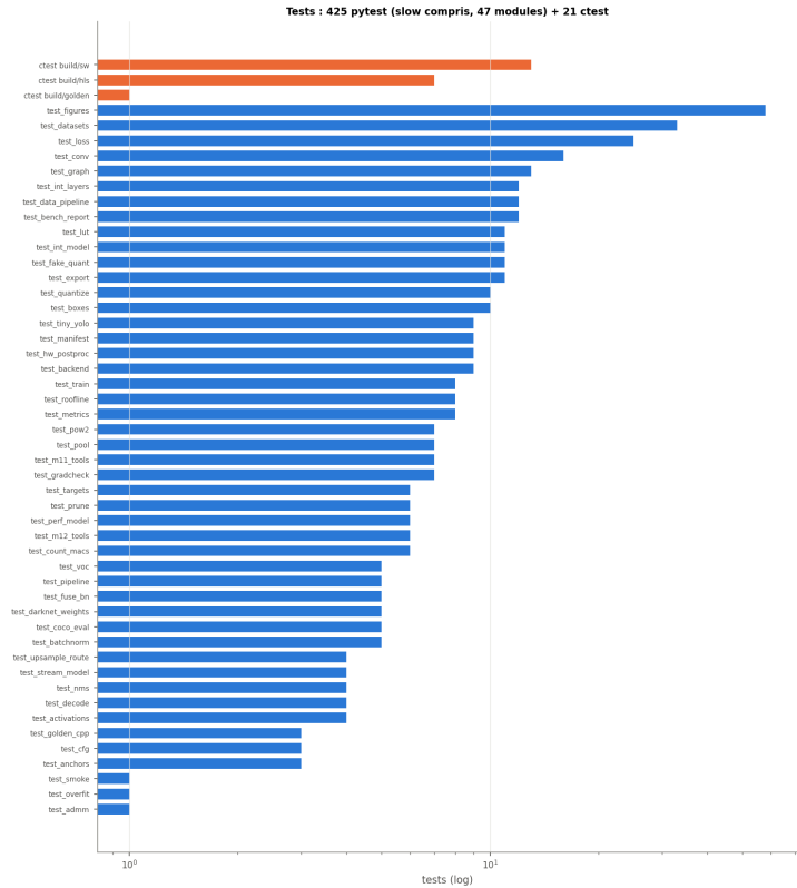
Figure 26: Nombre de tests par module Python (pytest, slow compris) et par build C++ (ctest), et leur durée quand make test-durations a été lancé. (tests)
