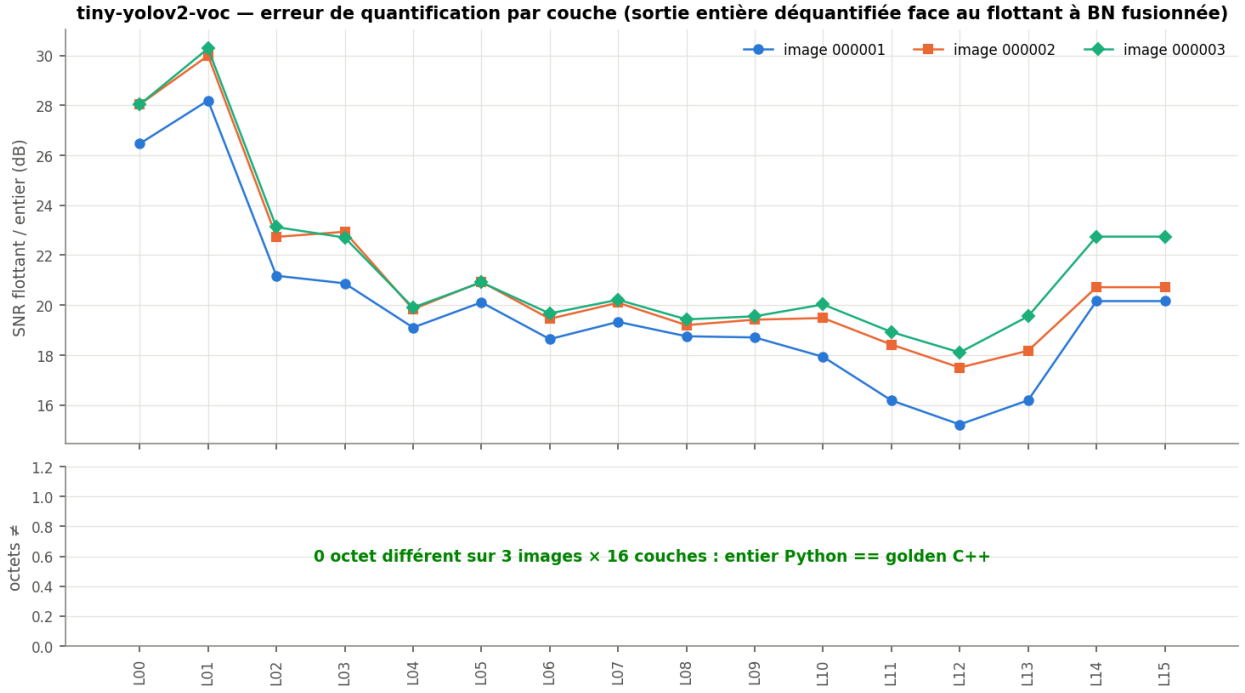
Figure 12: SNR par couche entre le flottant et l'entier déquantifié, et écart entier Python ↔ golden C++ (0 partout : bit-exact). ( erreur_couches )
