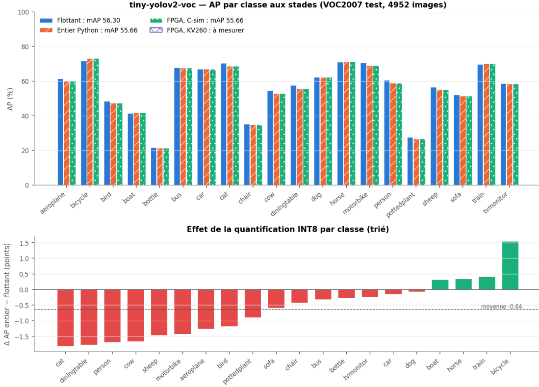
Figure 20: AP par classe aux stades flottant, entier et C-sim (la carte quand elle sera mesurée), et écart entier – flottant trié. (map_stades)
