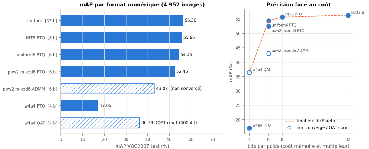
Figure 23: mAP de Tiny-YOLOv2 selon le format des poids (flottant, INT8, puissances de 2, 4 bits), et frontière précision / bits. (map_formats)
