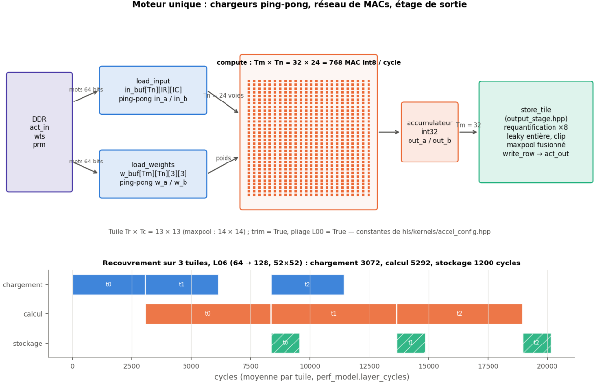
Figure 14: Moteur unique : chargeurs ping-pong, réseau T_m \times T_n de MACs, accumulateur, étage de sortie, et chronogramme du recouvrement sur 3 tuiles. (moteur)
