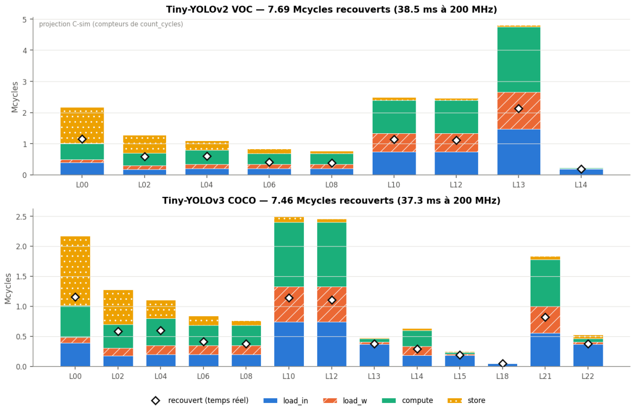
Figure 19: Cycles par couche du noyau actuel, décomposés en chargements, calcul et stockage ; le losange donne le temps réel avec recouvrement. (cycles_couches)
