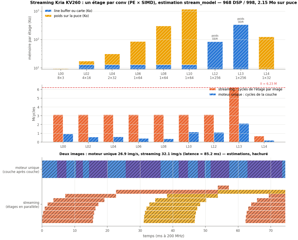
Figure 24: Architecture streaming face au moteur unique : mémoire et parallélisme par étage, cycles par couche, chronogramme sur deux images (estimations). ( streaming )
