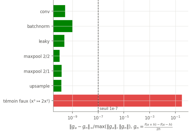
Figure 5: Rétropropagation écrite à la main : formule du gradient renvoyé par chaque couche, puis l'erreur du gradcheck par couche face au seuil 1e-7. (retropropagation)
