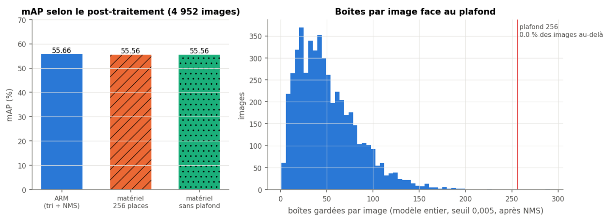
Figure 22: mAP avec le post-traitement matériel, avec et sans plafond de boîtes, et nombre de boîtes par image face au plafond. (hw_postproc)
