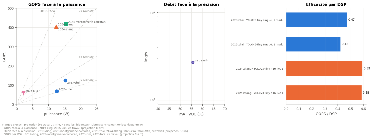
Figure 1: Comparaison aux accélérateurs publiés : GOPS et puissance, débit et mAP, GOPS par DSP (marque creuse : projection de ce travail). ( etat_art )
