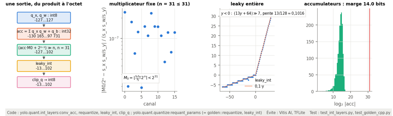
Figure 10: Arithmétique entière du matériel : chaîne d’une sortie, multiplicateur fixe M_0/2^n , leaky entière 13/128 et marge des accumulateurs int32. (entier)
