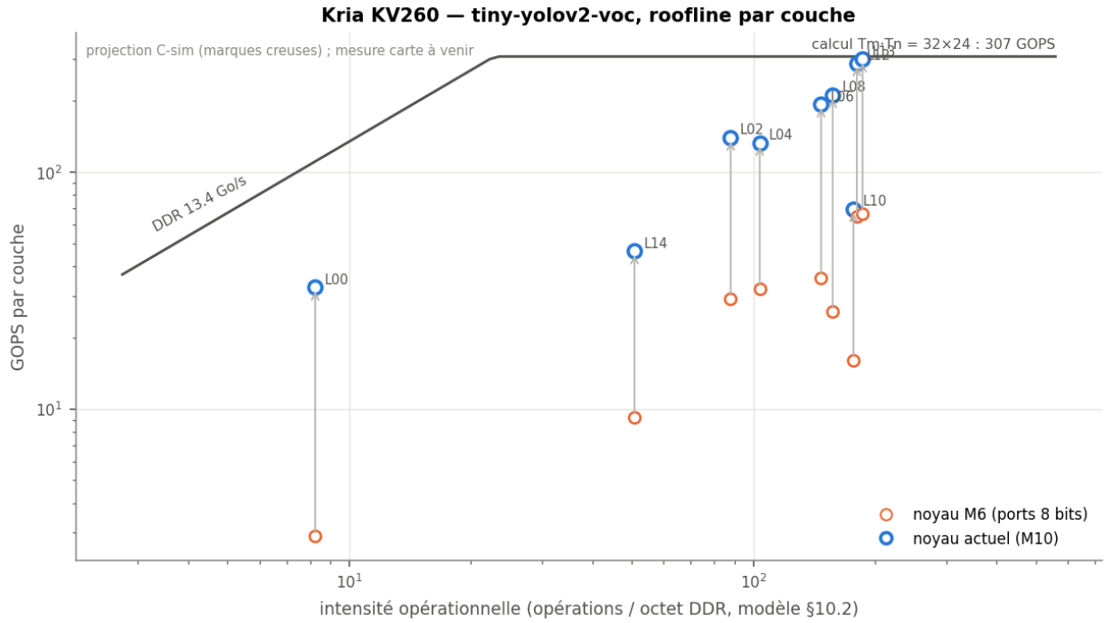
Figure 18: Roofline KV260 avec un point par couche de Tiny-YOLOv2, avant et après les optimisations M10. (roofline_couches)
