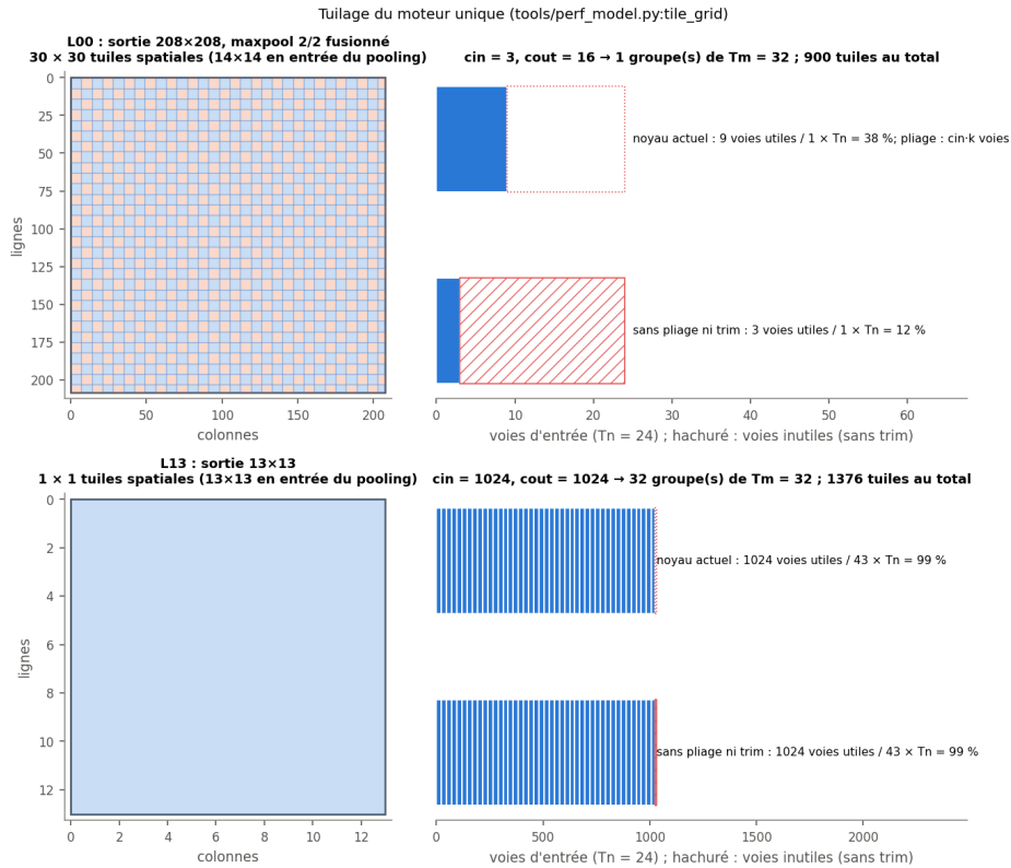
Figure 15: Tuilage de deux couches : tuiles spatiales et voies d'entrée, avec le pliage de L00 (cin = 3) et la couche 13×13 couverte par une seule tuile. (tuilage)
