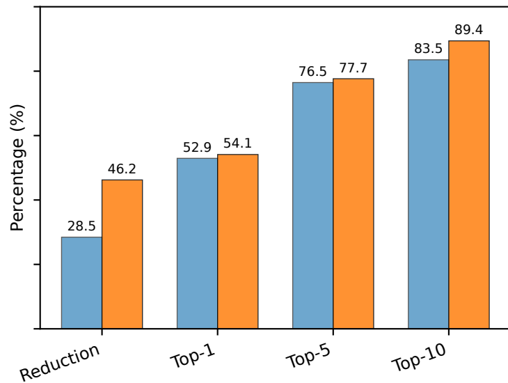
RIKEN-PlaSMA
