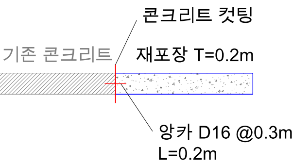
접속부 상세 (NO.0, NO.2+2)
