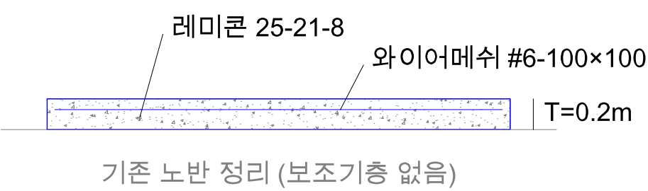
대표 횡단면 (NO.0 ~ NO.2+2)
