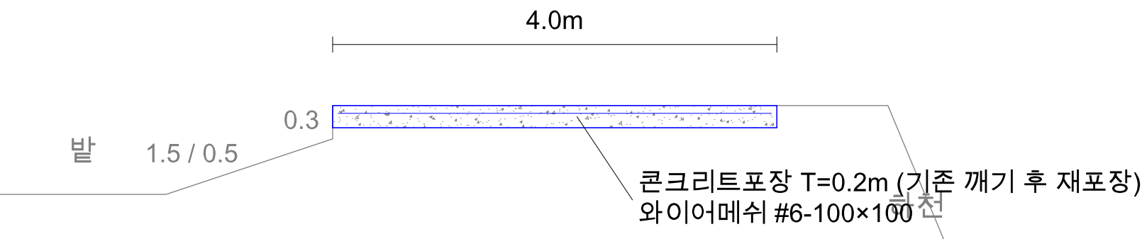
대표 횡단면 (NO.0 ~ NO.2+2)
