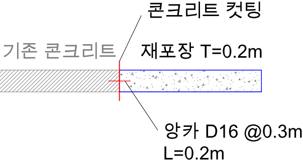
접속부 상세 (NO.0, NO.2+2)
