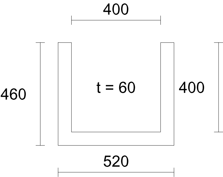
U형 수로관 400C
