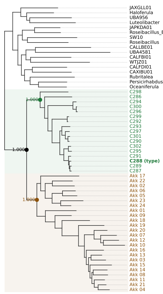
A bac120 phylogeny
