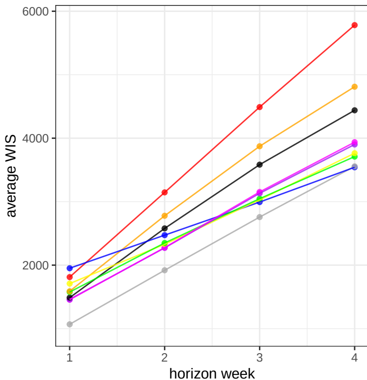
BA.4/BA.5 (US)
