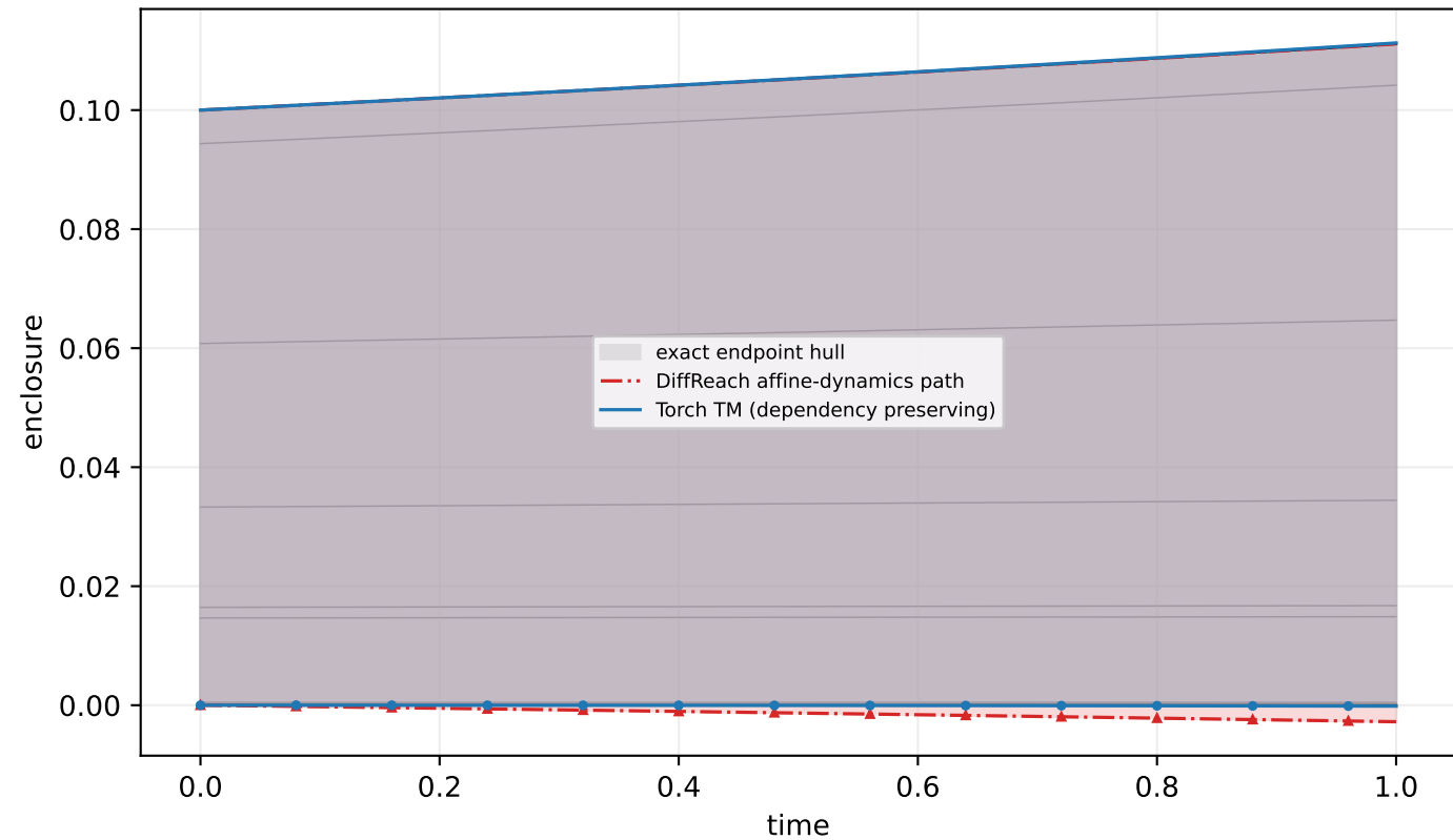
riccati: state 0, h=0.01 , T=1 (primary)
