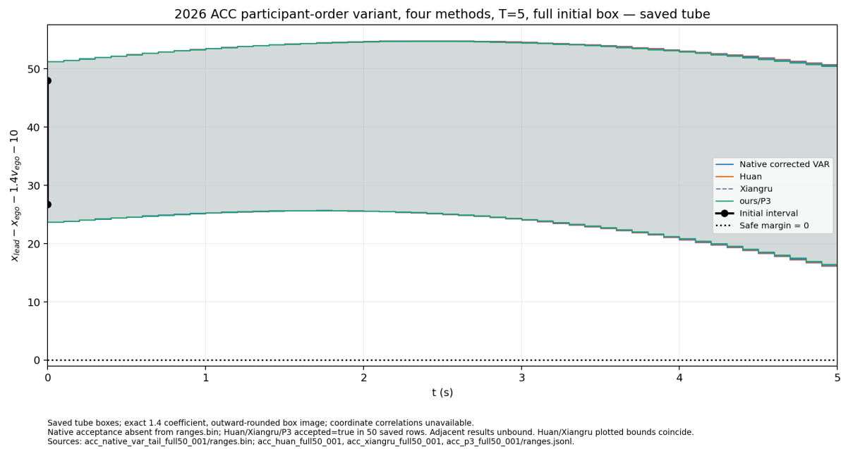
图 4 ACC 四方每期 whole-tube 盒的保守 safe-distance margin；虚线为全时 margin=0 边界。
