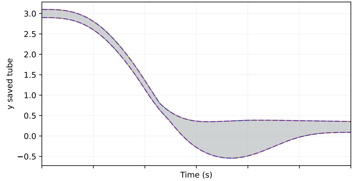
Robust: y
