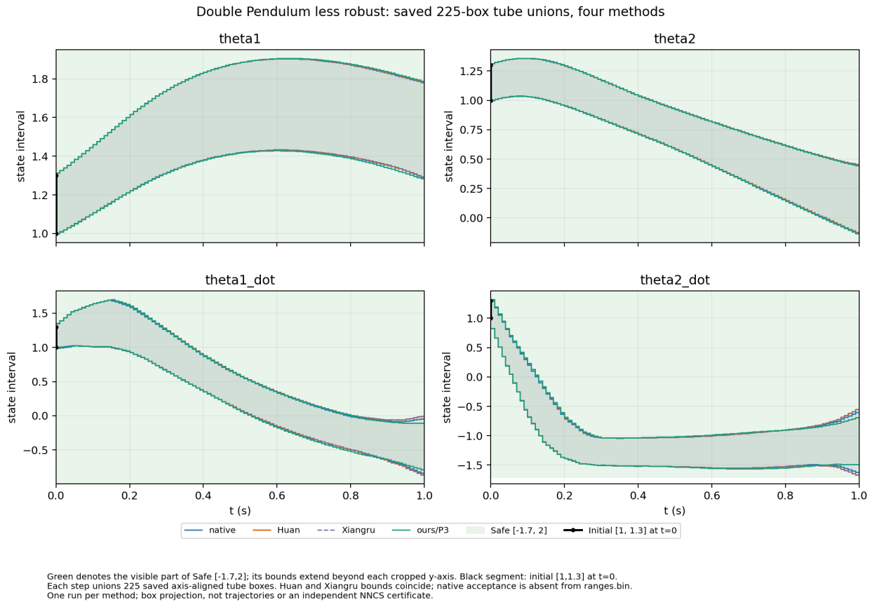
图 4 DP less 四方法完整 225 盒四态 tube union 与全时安全带。
