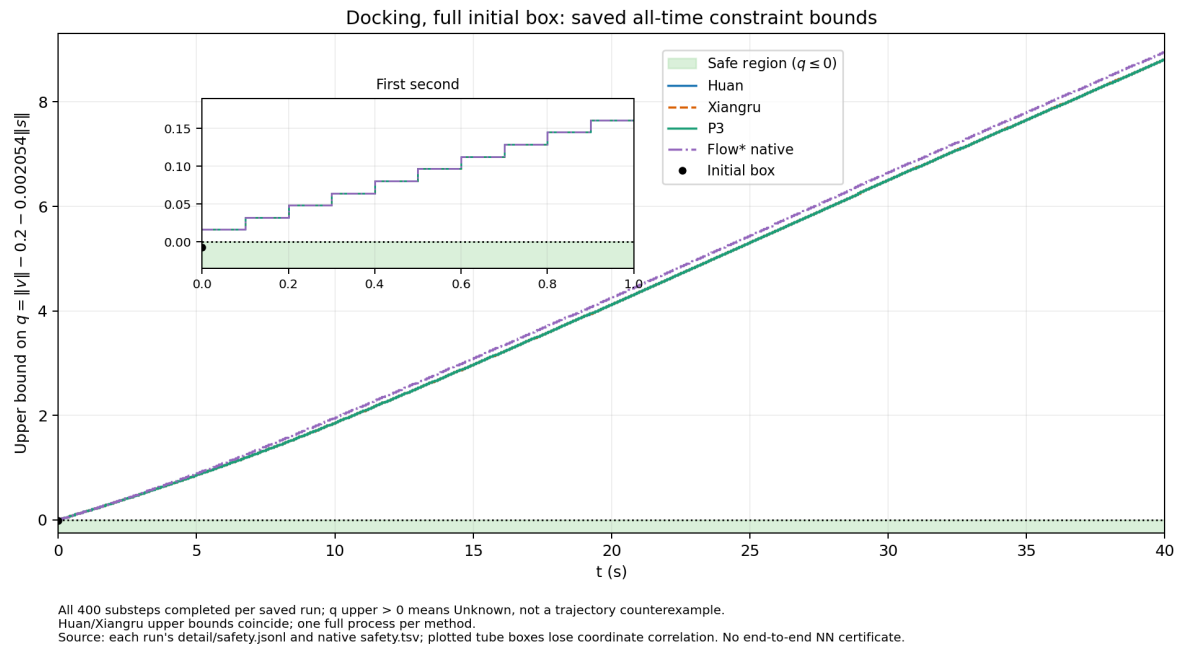
图 6 Docking 四方保存 tube 的 q 上界；绿色为 q \leq 0 安全区域，内框放大第一秒。
