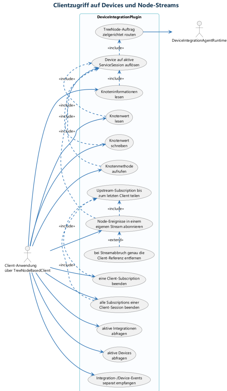
Abbildung 6: TreeNode-Aufrufe und Subscriptions aus Clientsicht (PlantUML)
