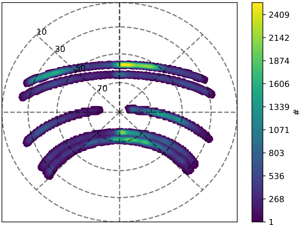
baseline_v5.1.0_10yrs DDFs
