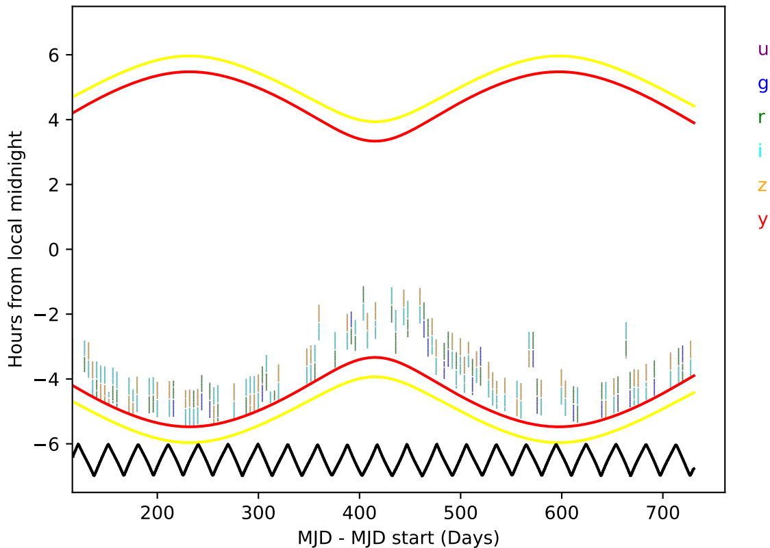
baseline_v5.1.0_10yrs Initial Long night < 730
