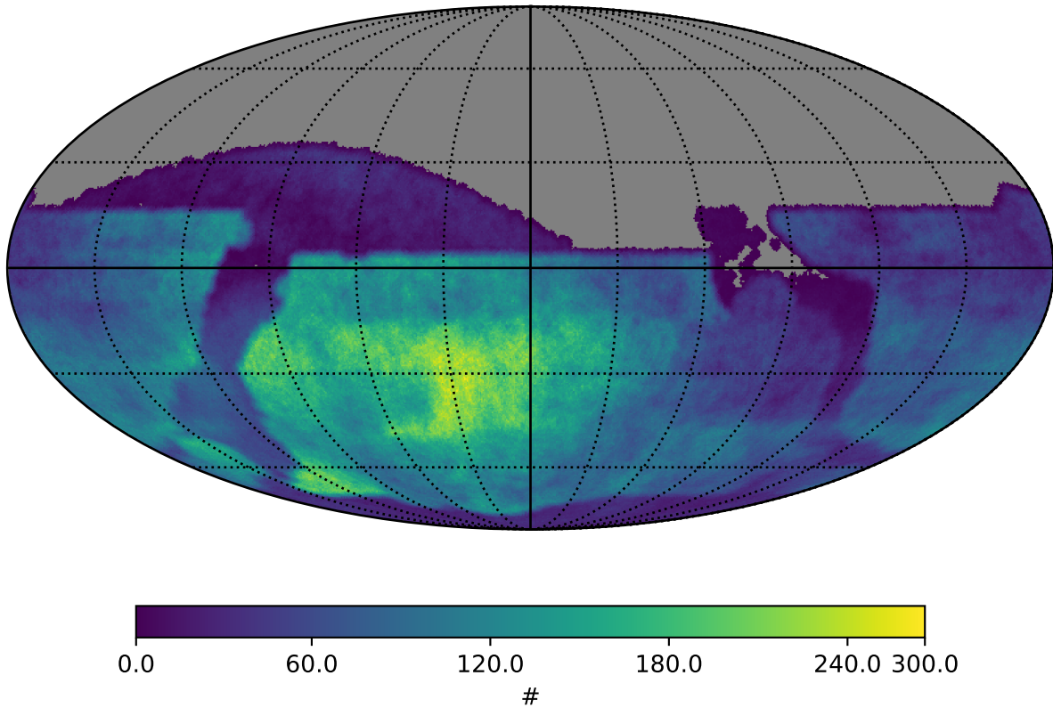
baseline_v5.1.0_10yrs Pair 15
