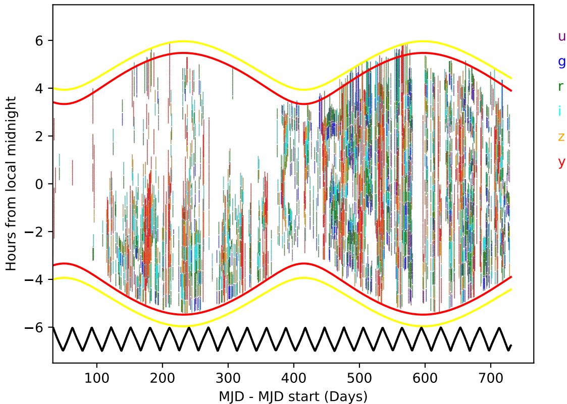
baseline_v5.1.0_10yrs Pair 33 night < 730
