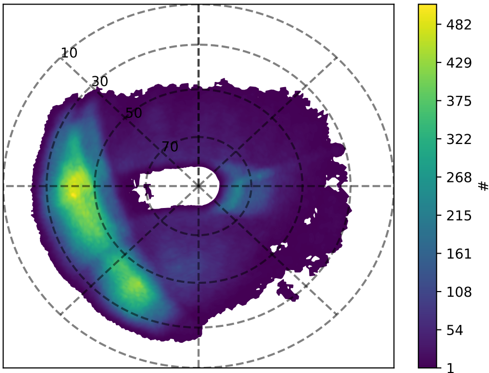
baseline_v5.1.0_10yrs Final Long
