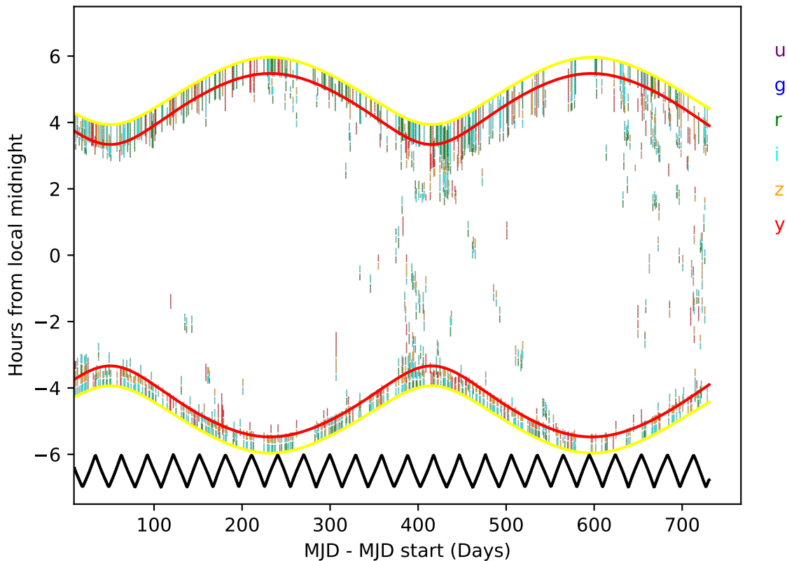
baseline_v5.1.0_10yrs Pair 15 night < 730
