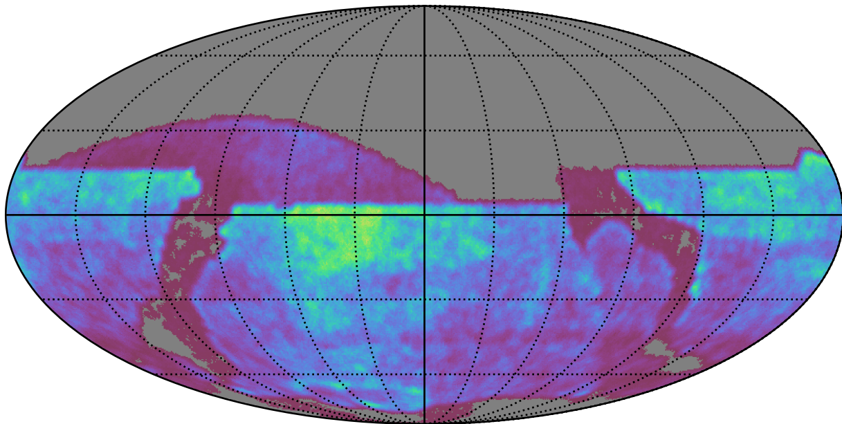
Greedy (v5.1.0)
