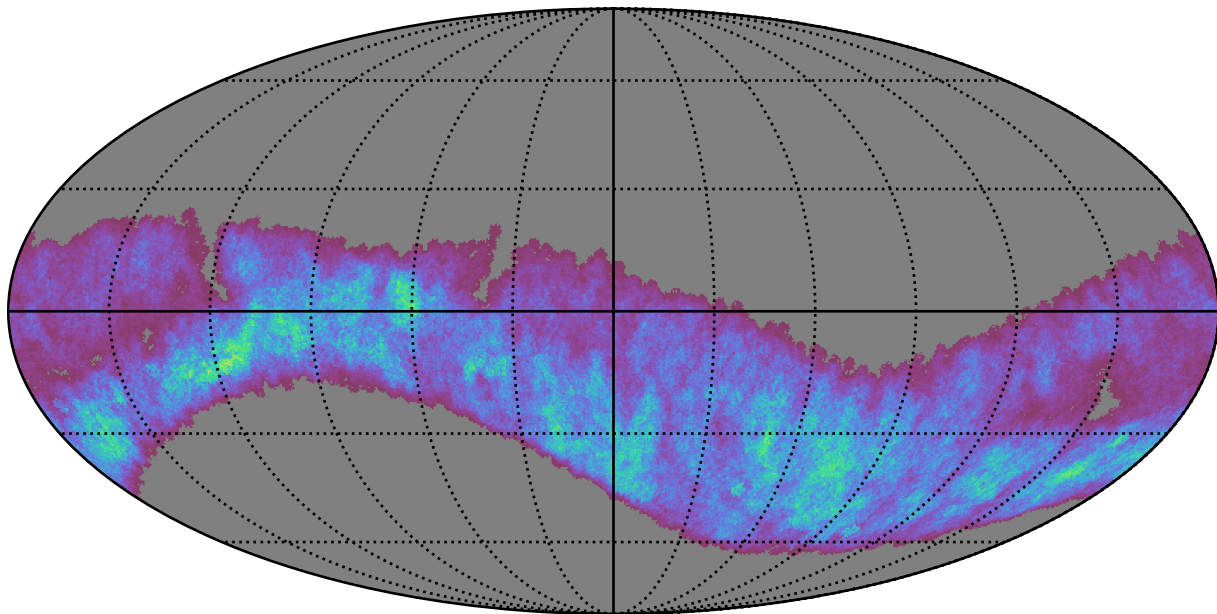
Twilight Earth-Interior (v5.1.0)
