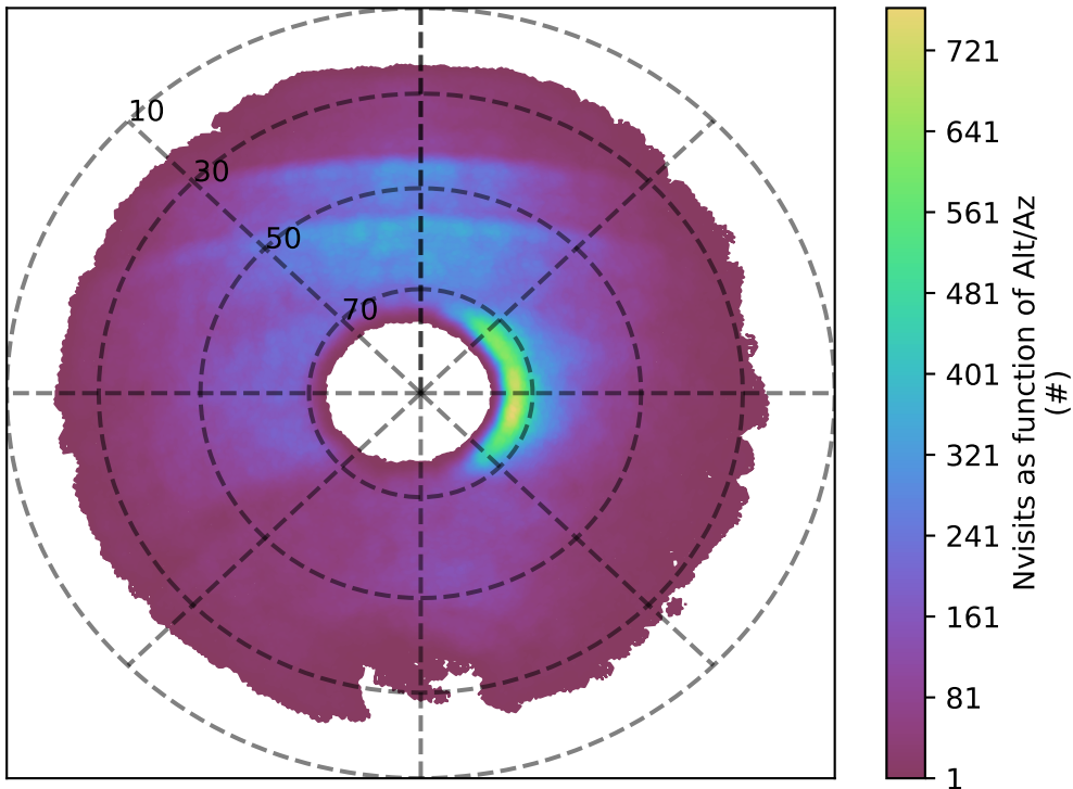
Greedy (v5.1.0)
