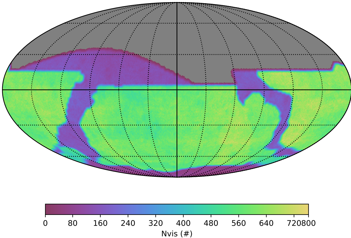
33 Min Pairs
