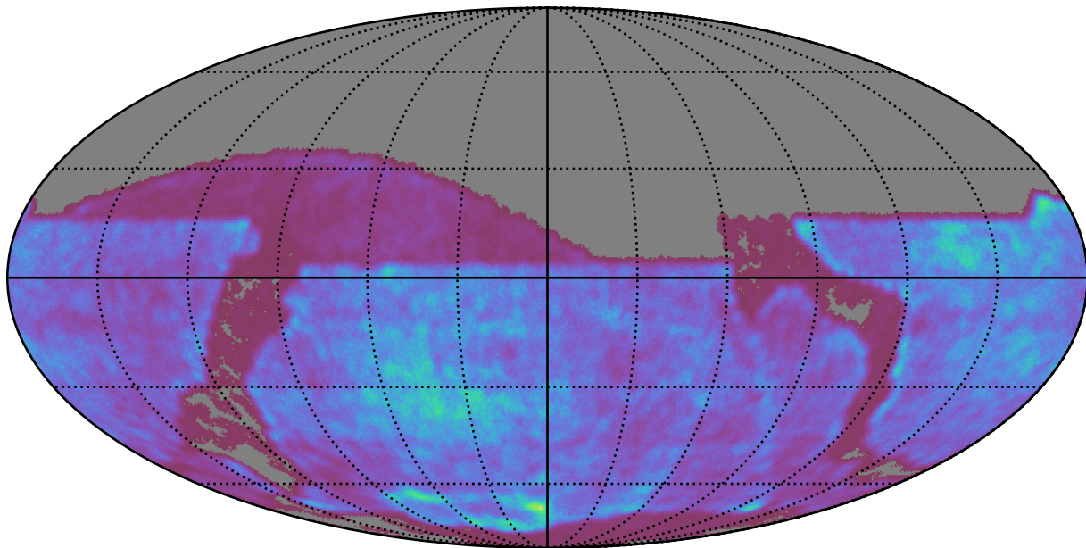
Greedy (v4.3.1)
