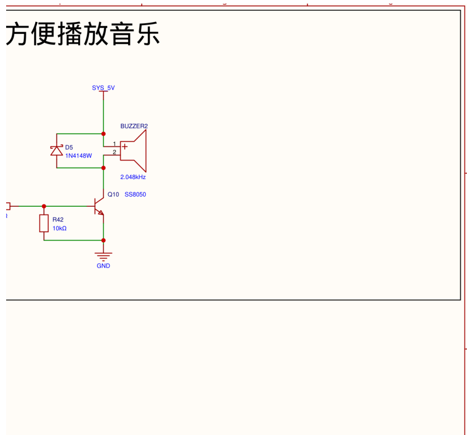
无源蜂鸣器、SS8050 低侧驱动与续流
