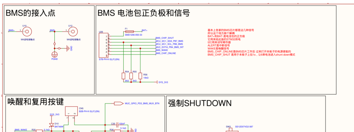
BMS 7P 跨板接口与上拉/辅助 BAT+
