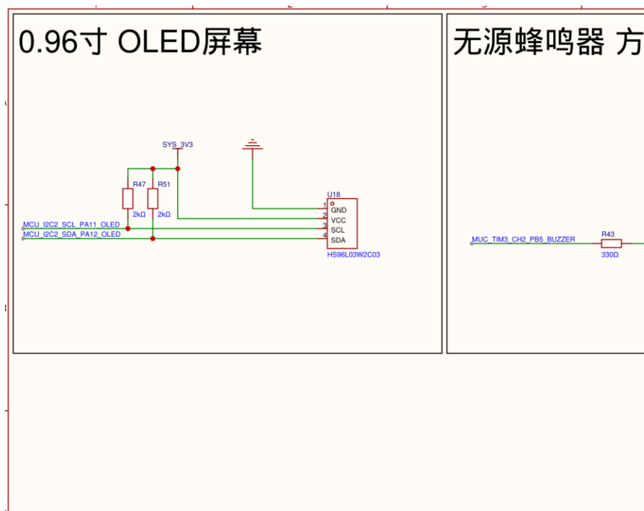
SSD1315 OLED 与 I2C2 上拉
