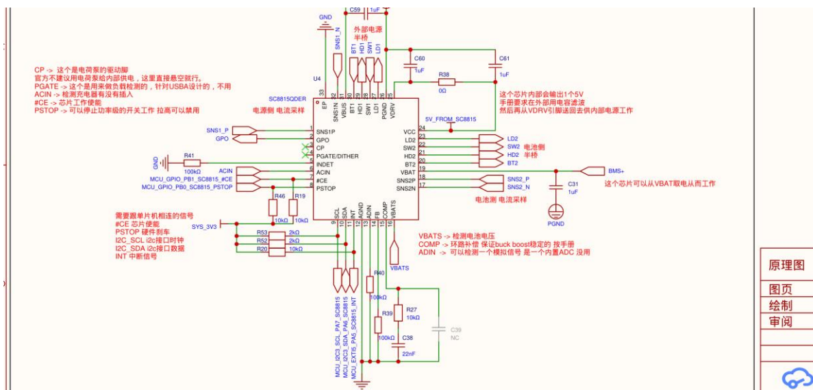
SC8815 控制器、补偿、采样与控制引脚
