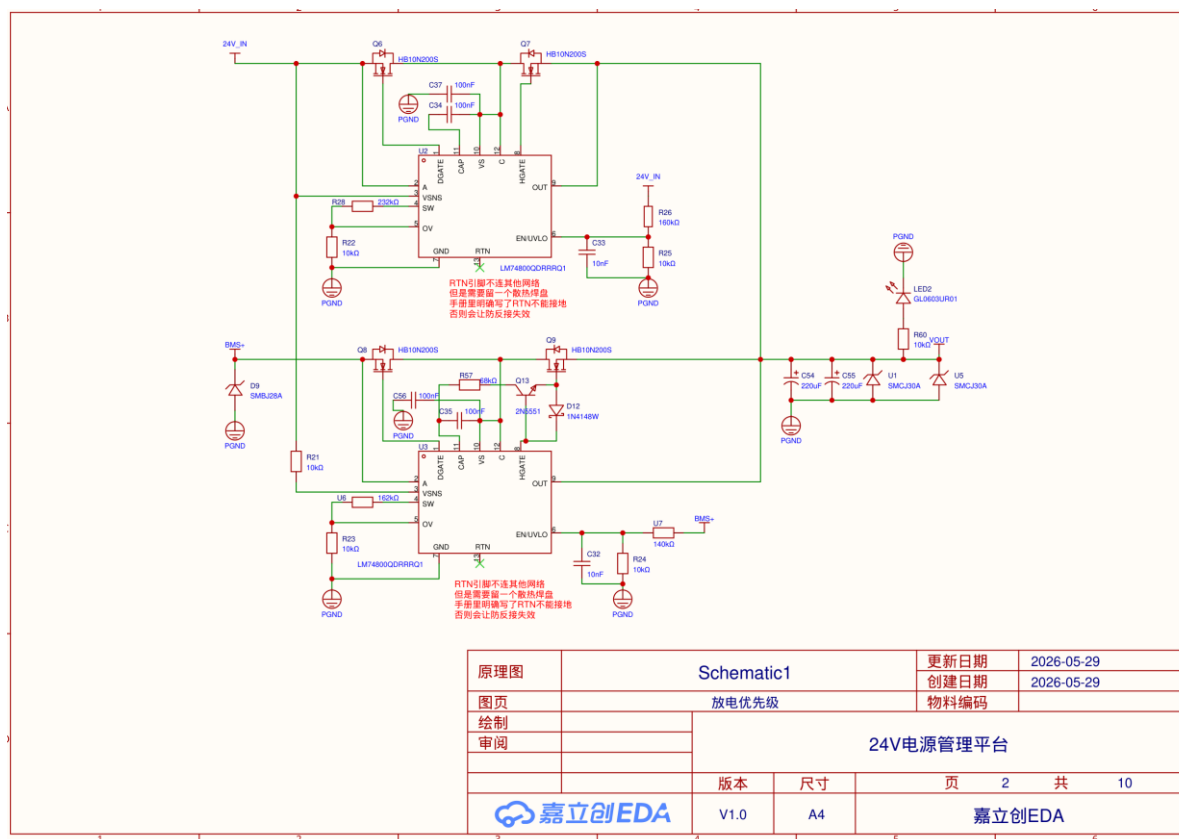
双路LM74800-Q1、背靠背MOS与VOUT 汇流
