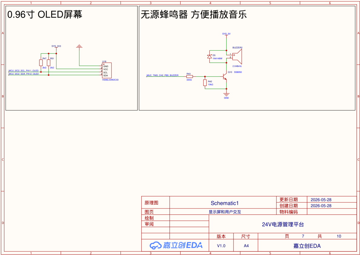
控制板 Page 7: OLED 和蜂鸣器驱动
