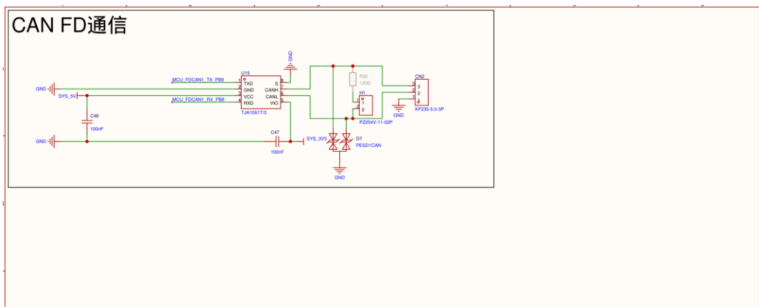
TJA1051T/3 CAN FD 收发器、ESD 与可选终端
