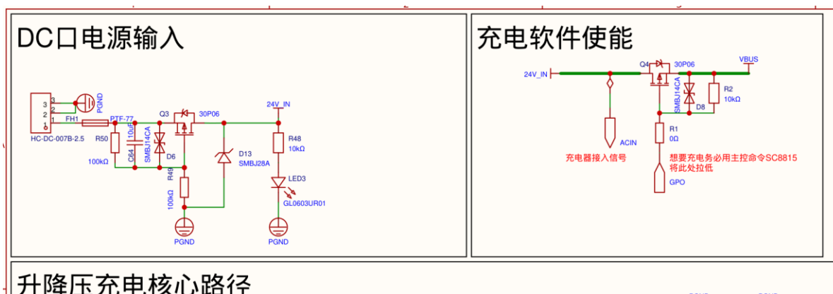
DC 输入、防反与软件高边使能
