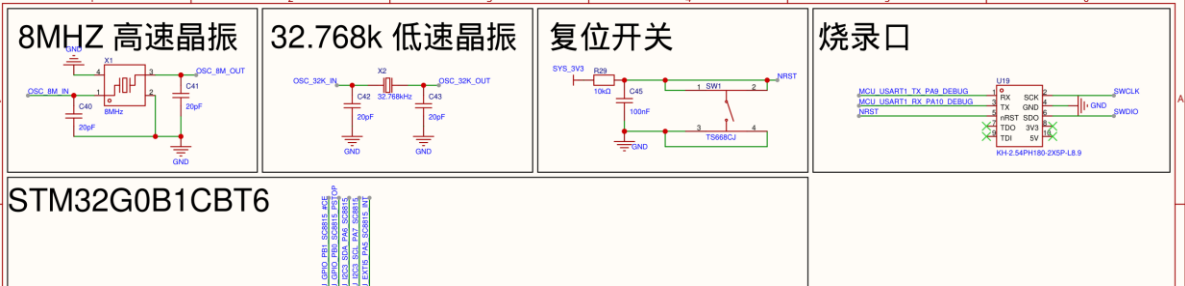
8MHz/32.768kHz 晶体、复位、SWD 与 UART
