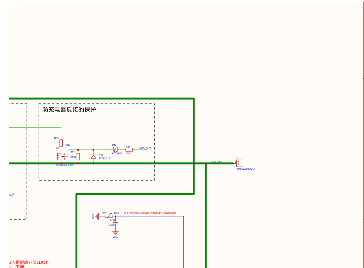
预放电、反接辅助与输出钳位
