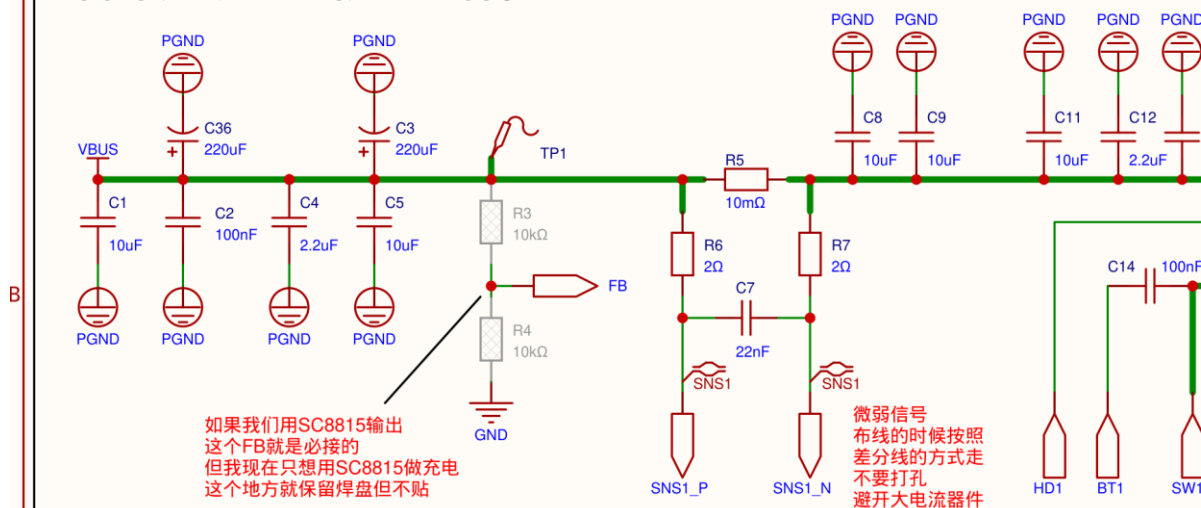
放大分区 1/4 — VBUS 输入、SNS1 分流与输入去耦 (与相邻分区有重叠)
