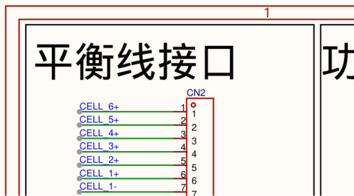
放大分区 1/4 — 平衡线接口 CN2 (与相邻分区有重叠)
