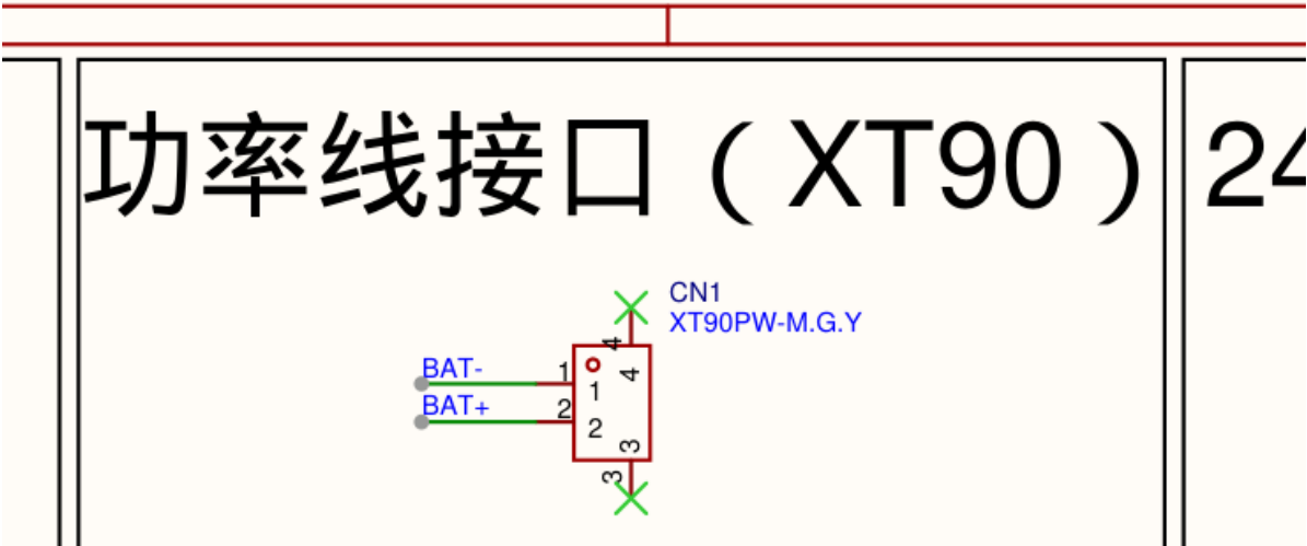
放大分区 2/4 — XT90 功率线接口 CN1（与相邻分区有重叠）
