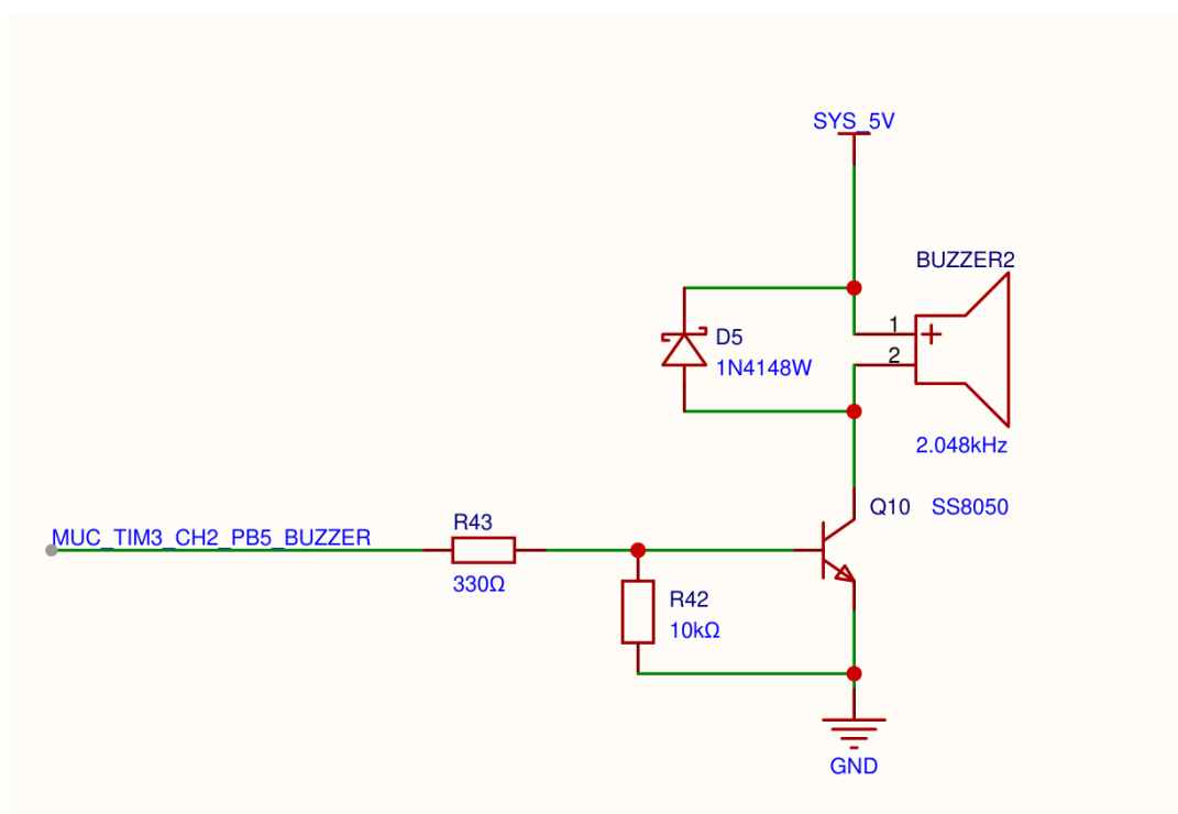
控制板 Page 7: OLED 和蜂鸣器驱动
