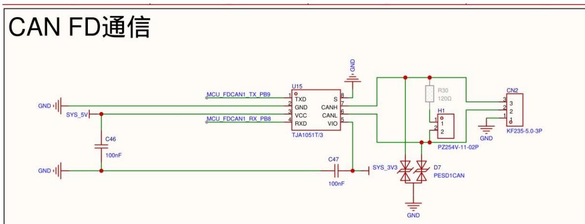
控制板 Page 6: CAN FD 收发器、ESD 和 120 欧姆终端
