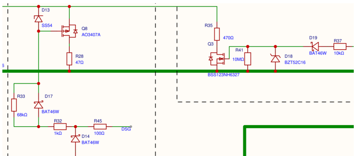
放大分区 3/4 — Q8 加速关断与 Q3/D19 反接辅助网络 (与相邻分区有重叠)
