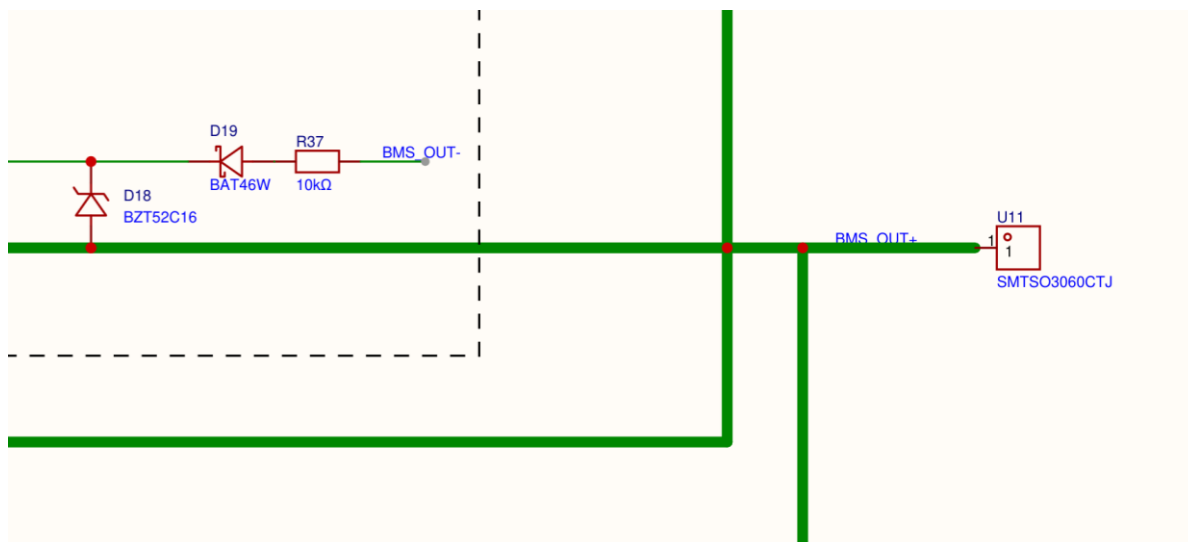
放大分区 4/4 — BMS_OUT+ 汇出、钳位与端子 (与相邻分区有重叠)
