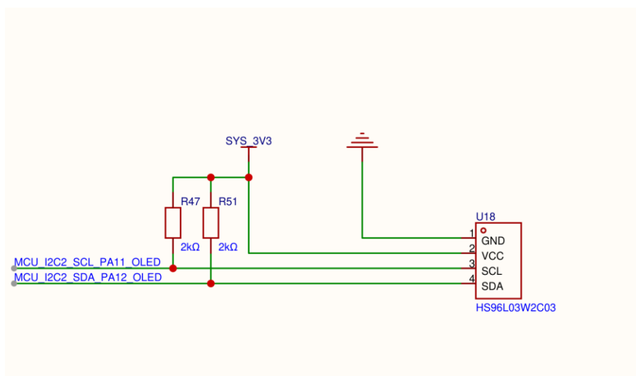
SSD1315 OLED 与 I2C2 上拉
