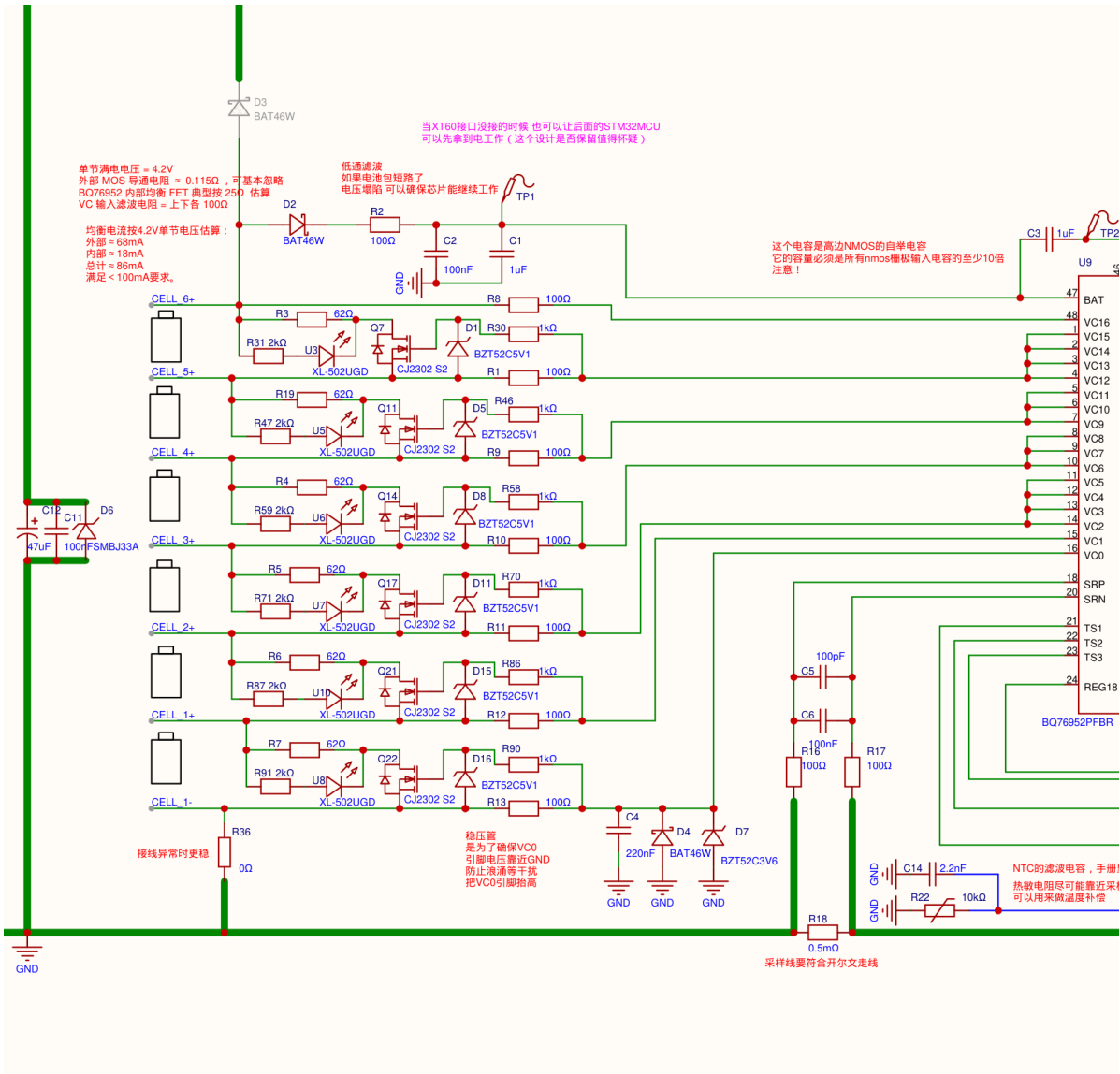
六路电芯采样滤波与外部被动均衡 (原始矢量局部放大; 图边外连接见附录整页原理图)
