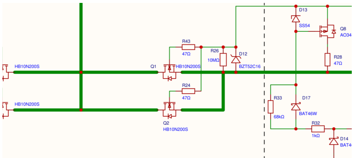
放大分区 2/4 — 共漏节点、Q1/Q2 放电 MOS 组与 DSG 驱动 (与相邻分区有重叠)
