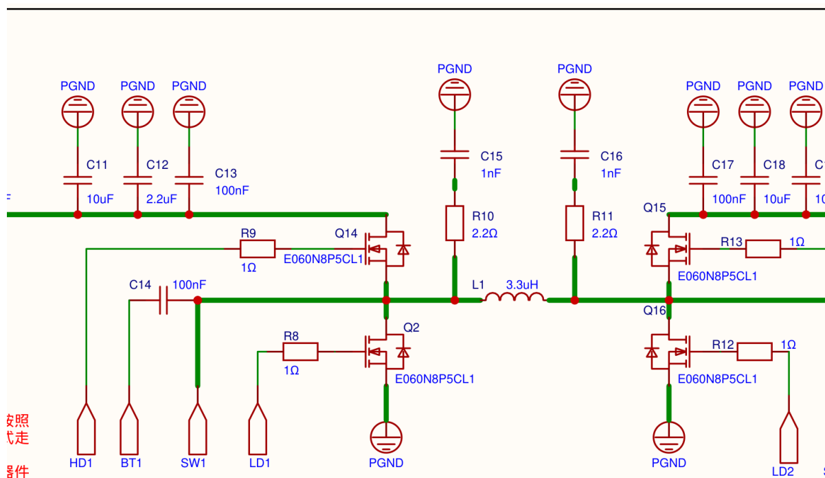
放大分区 2/4 — Q14/Q2 左桥臂、L1 与第一开关节点 (与相邻分区有重叠)
