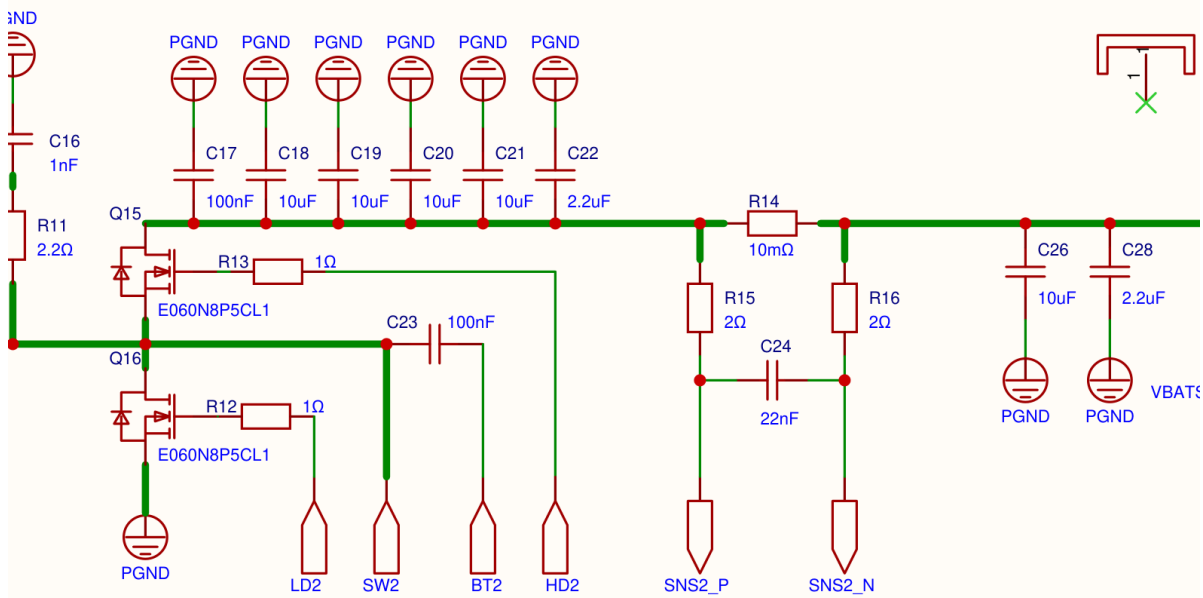
放大分区 3/4 — Q15/Q16 右桥臂与第二开关节点 (与相邻分区有重叠)
