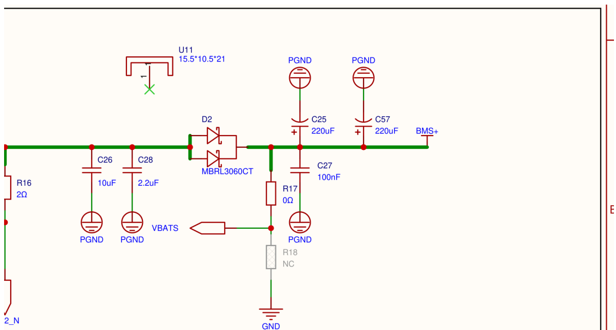
放大分区 4/4 — SNS2 分流、输出去耦、D2 与 BMS+ (与相邻分区有重叠)
