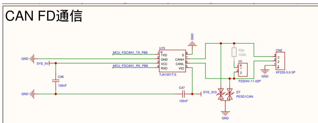
TJA1051T/3 CAN FD 收发器、ESD 与可选终端
