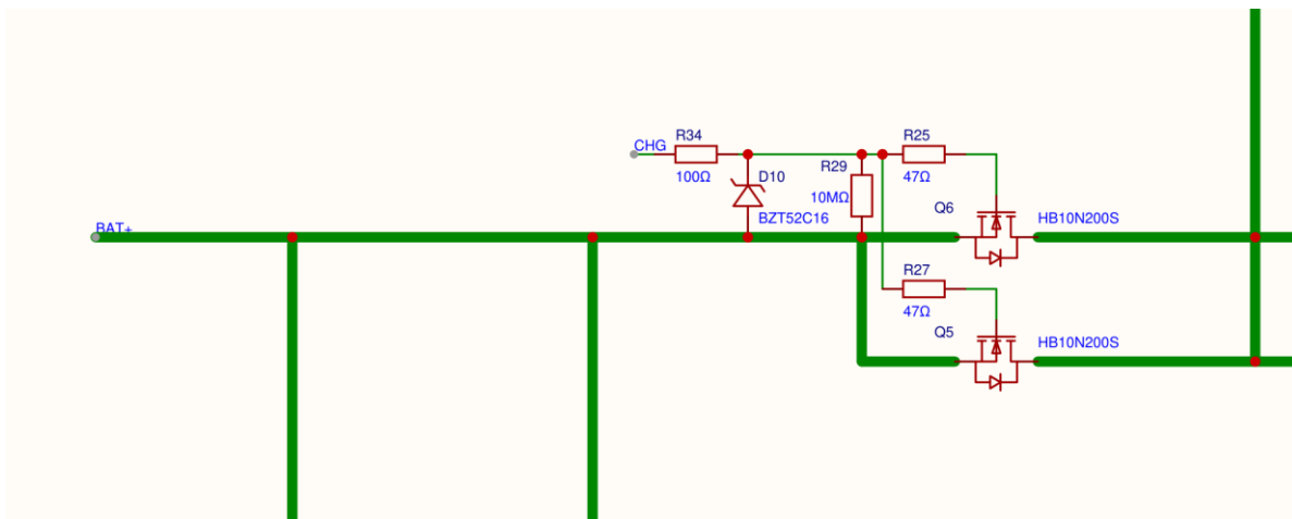
放大分区 1/4 — BAT+、CHG 驱动与 Q5/Q6 充电 MOS 组（与相邻分区有重叠）
