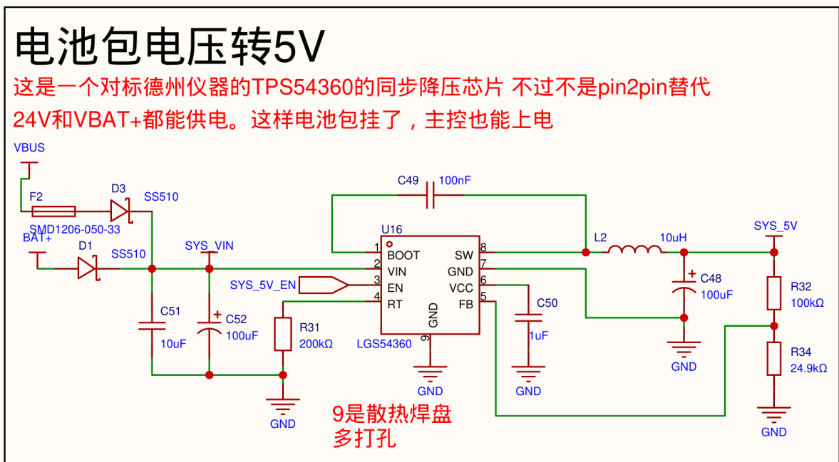
VBUS/BAT+ 辅助电源 OR 与 5V Buck
