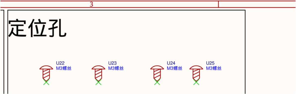
放大分区 4/4 — M3 定位件 U22-U25（与相邻分区有重叠）
