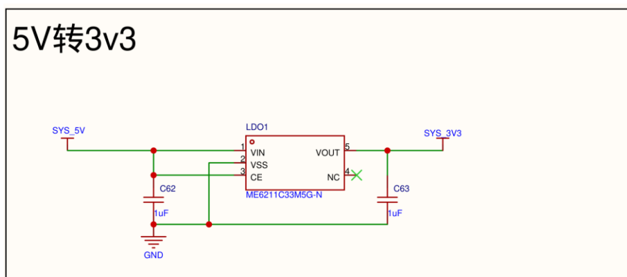
ME6211 3.3V LDO 与去耦
