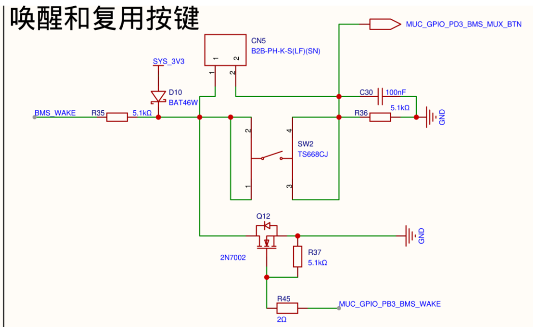
唤醒与复用按键网络
