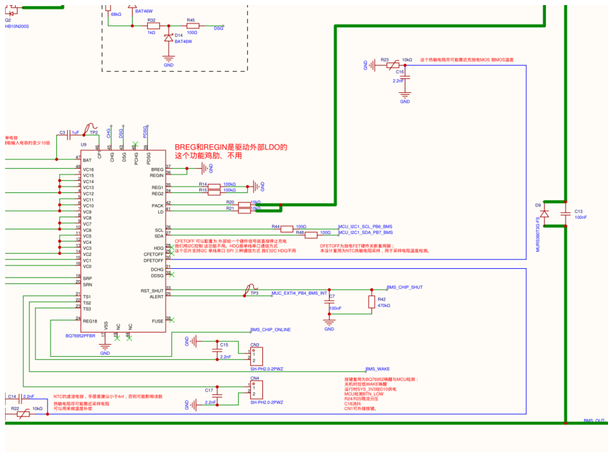
BQ76952 供电、通信与控制引脚 (原始矢量局部放大; 图边外连接见附录整页原理图)
