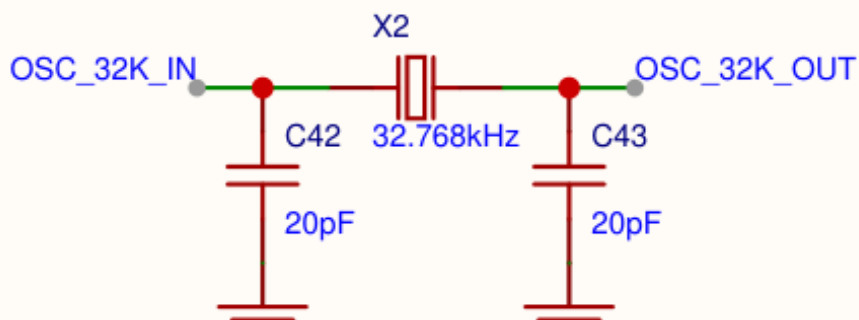
功能框 2/4 — 32.768kHz LSE 晶振
