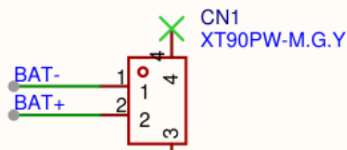
功能框 2/4 — XT90 功率线接口 CN1
