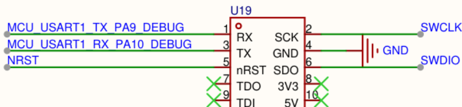
功能框 4/4 — SWD、NRST 与调试 UART 接口
