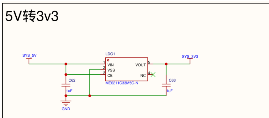
ME6211 3.3V LDO 与去耦
