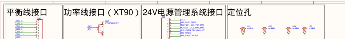
BMS 板连接器、电芯线与跨板接口 (完整总览；下列原始功能框分别放大)
