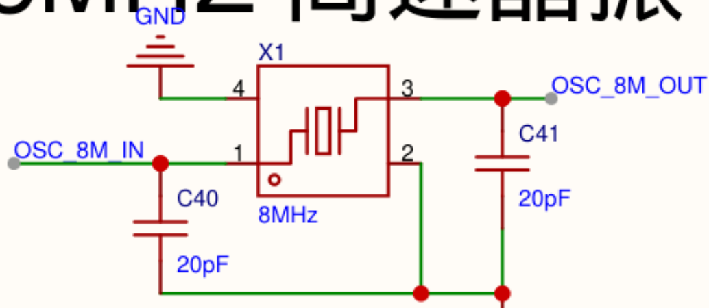
功能框 1/4 — 8MHz HSE 晶振
