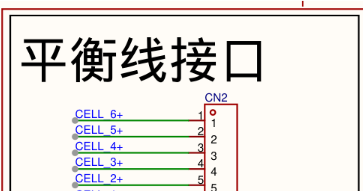
功能框 1/4 — 平衡线接口 CN2
