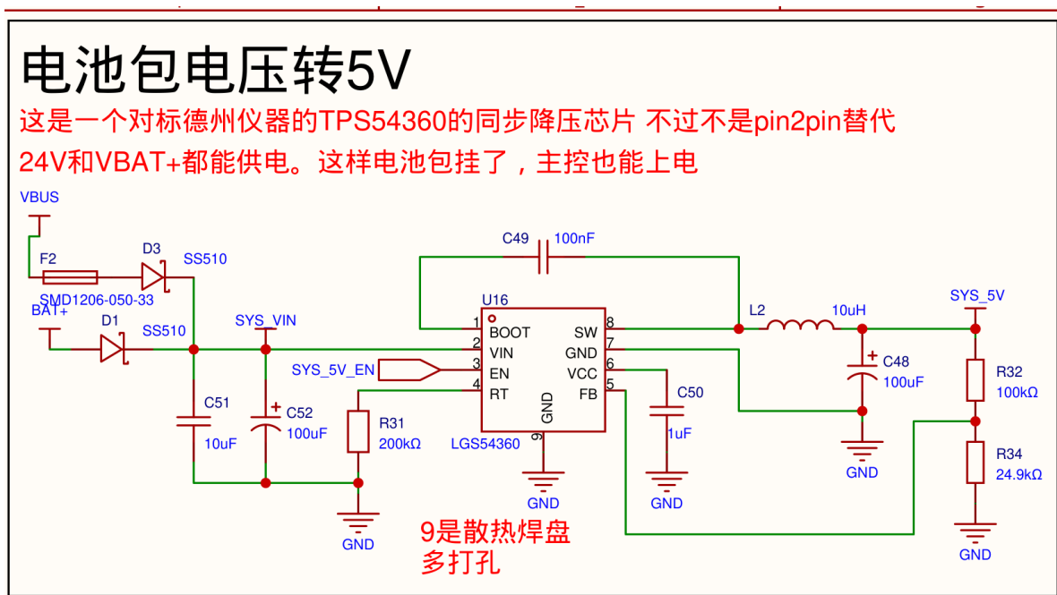
VBUS/BAT+ 辅助电源OR 与5V Buck
