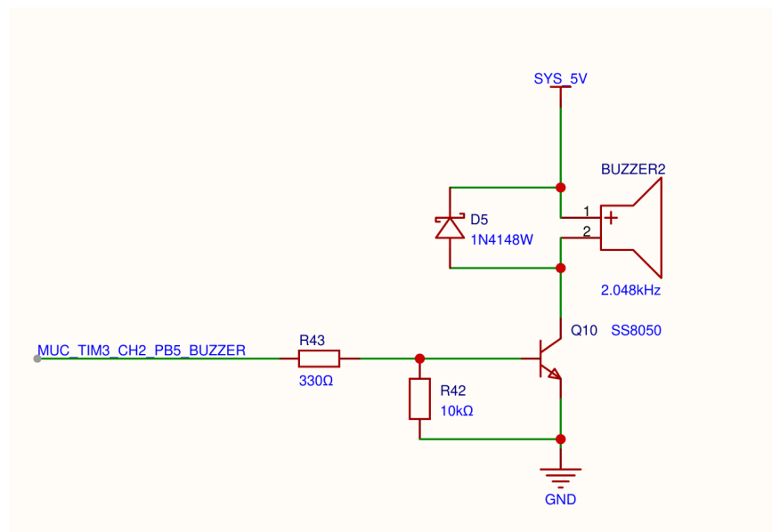
控制板 Page 7：OLED 和蜂鸣器驱动
