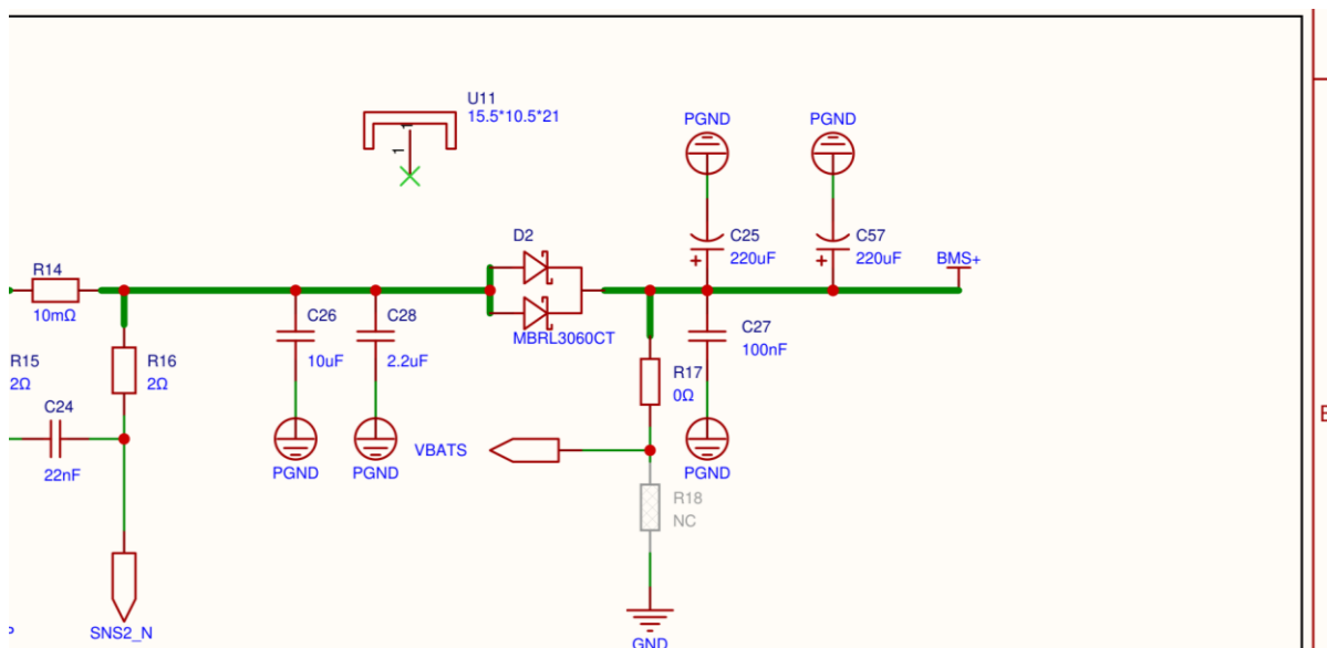
放大分区 3/3 — Q15/Q16 右桥臂、SNS2 分流、去耦、D2 与 BMS+ (与相邻分区有重叠)
