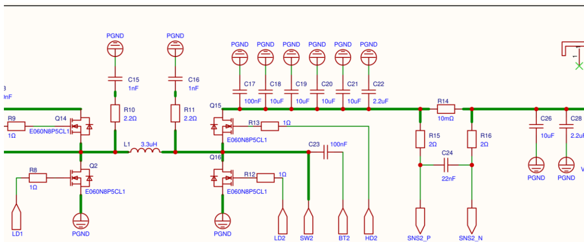
放大分区 2/3 — L1 与 Q14/Q2、Q15/Q16 四开关核心 (与相邻分区有重叠)
