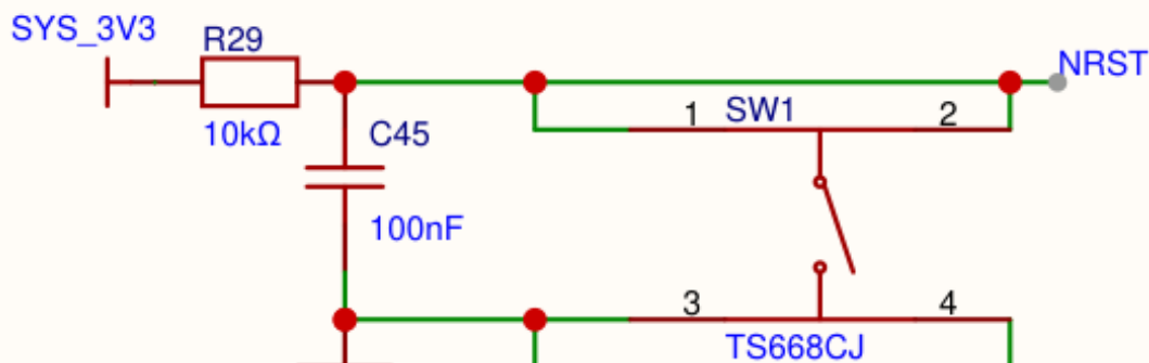
功能框 3/4 — NRST 上拉、RC 与复位按键
