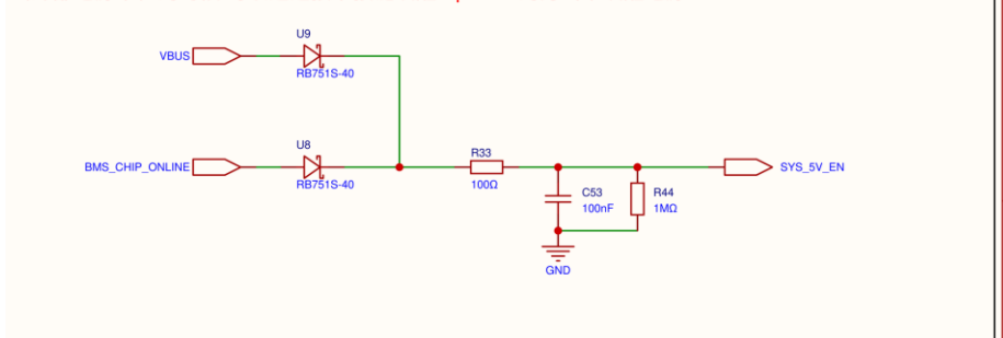
VBUS 与 BMS ONLINE 对 5V EN 的二极管 OR
