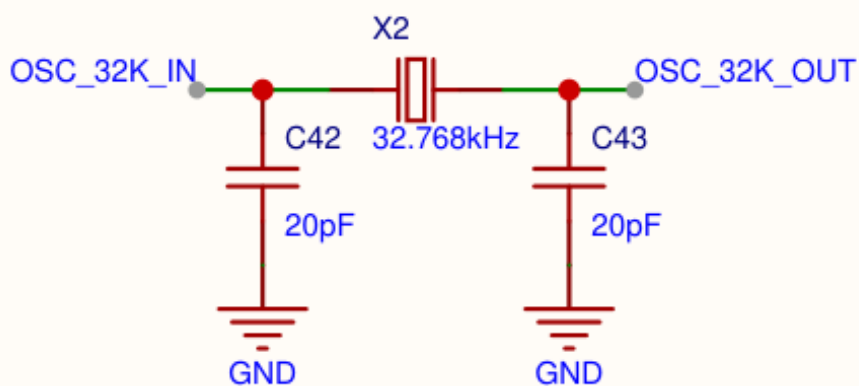
功能框 2/4 — 32.768kHz LSE 晶振
