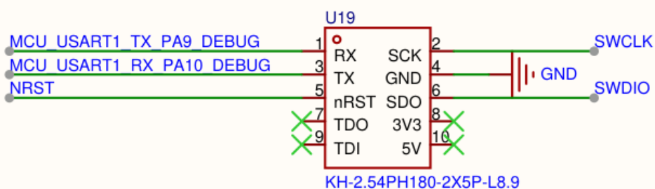
功能框4/4 — SWD、NRST 与调试UART 接口
