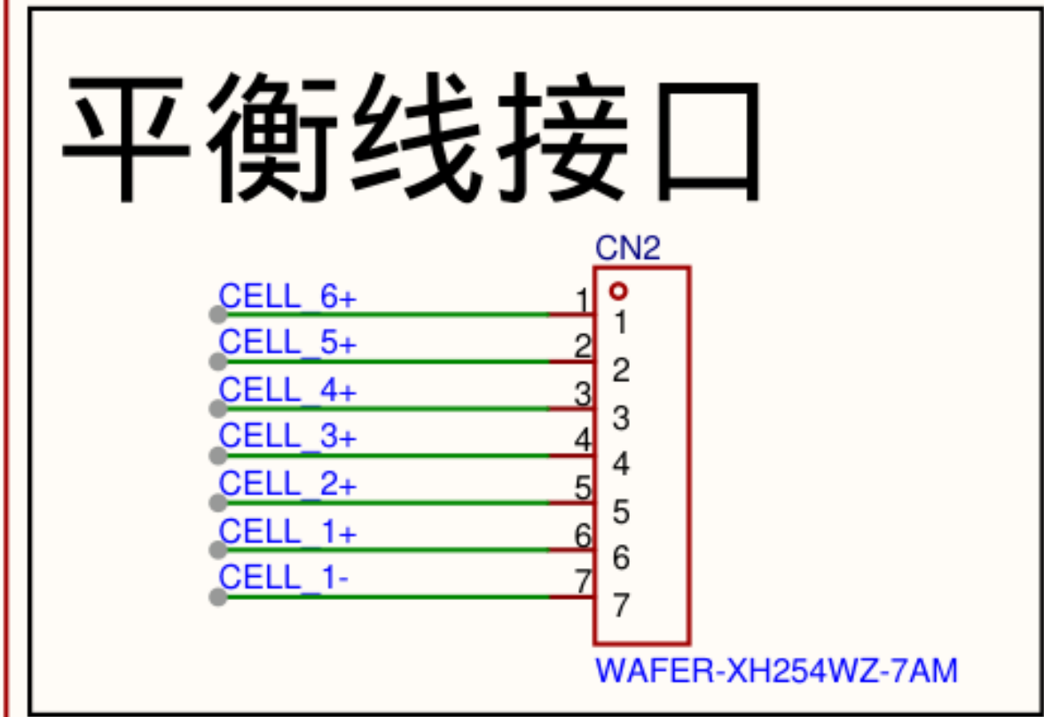
功能框 1/4 — 平衡线接口 CN2
