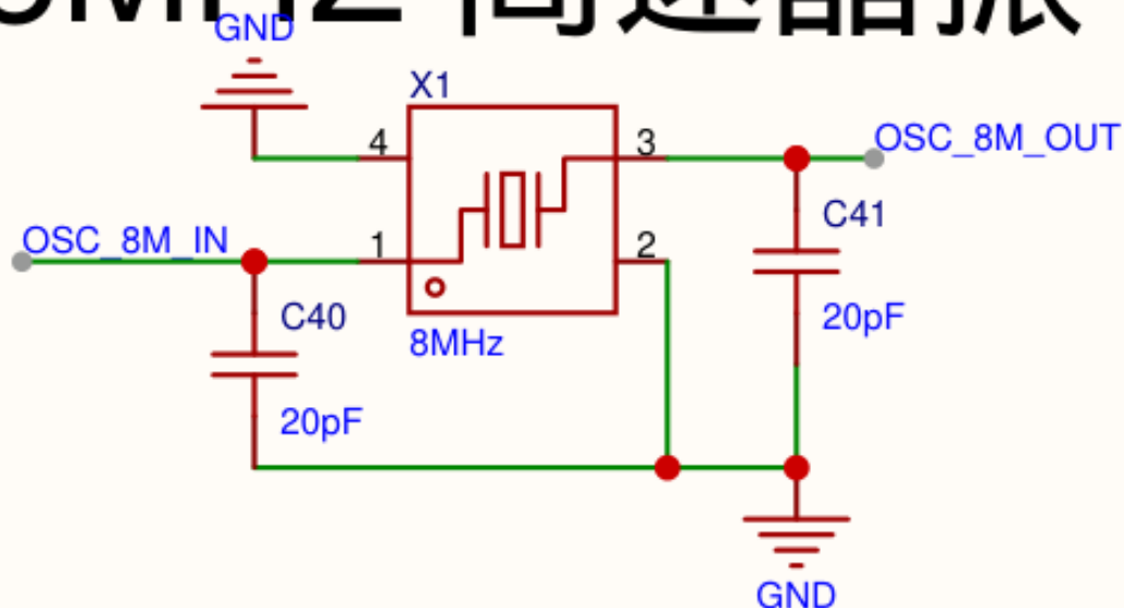
功能框 1/4 — 8MHz HSE 晶振
