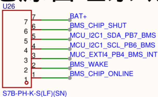
功能框 3/4 — 24V 电源管理跨板接口 U26
