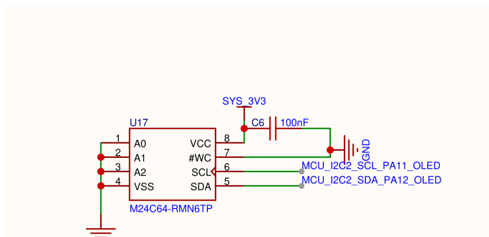
M24C64 EEPROM、地址脚与写保护
